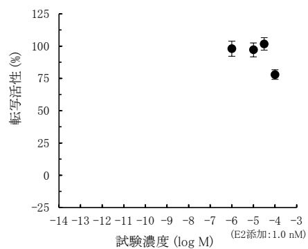
フタル酸ジ(2-エチルヘキシル)
