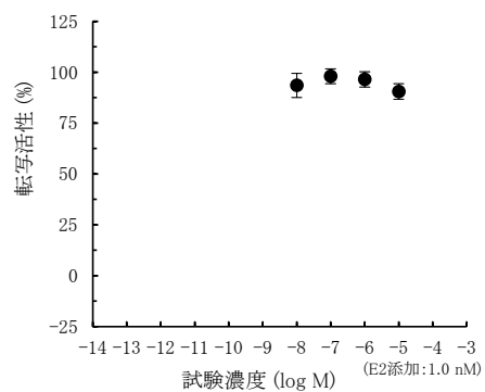
4-メチルベンジリデン=カンファー
