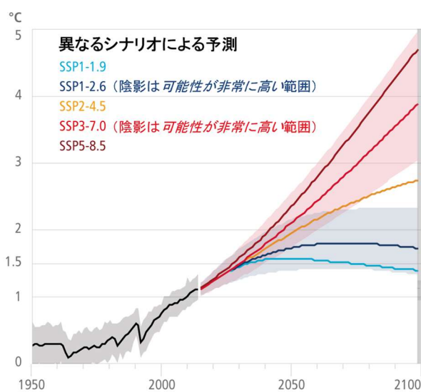
(a) 世界平均気温の変化 1850~1900年を基準とした上昇量
