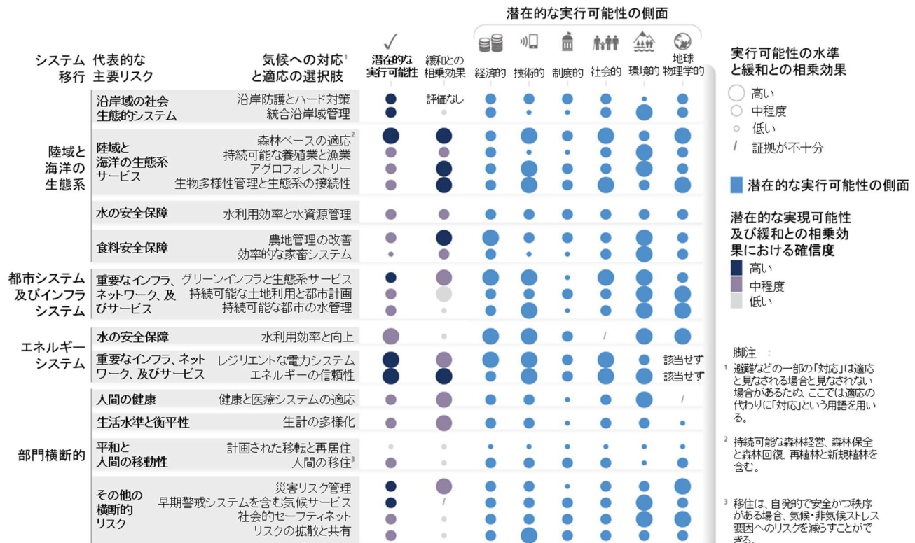
図 SPM.4: (a) 気候への対応と適応オプションを、システム移行と代表的な主要リスク（RKR）ごとに整理し、短期における、及び地球温暖化水準が 1.5°C以下における多側面の実行可能性について地球規模で評価する。1.5°Cを超える文献は限られているため、より高い水準の温暖化での実行可能性が変わるかもしれないが、これは現時点では明確に評価できない。地球規模での気候への対応と適応オプションは、実行可能性の各側面にわたって明確な証拠を有する、AR6 で評価された一連の選択肢から導き出されている。この図は、気候への対応と適応オプションの潜在的な実行可能性を算出するために使用される 6 つの実行可能性の側面（経済的、技術的、制度的、社会的、環境的、地球物理学的）と共に、それらの緩和との相乗効果を示す。潜在的な実行可能性と実行可能性の側面について、「高い」「中程度」「低い」の実行可能性の水準を図示する。緩和との相乗効果は、「高い」「中程度」「低い」で示す。証拠が不十分な場合は横棒で示す。{CCB FEASIB, 表 SMCCB FEASIB.1.1, SR1.5 4.SM.4.3}
