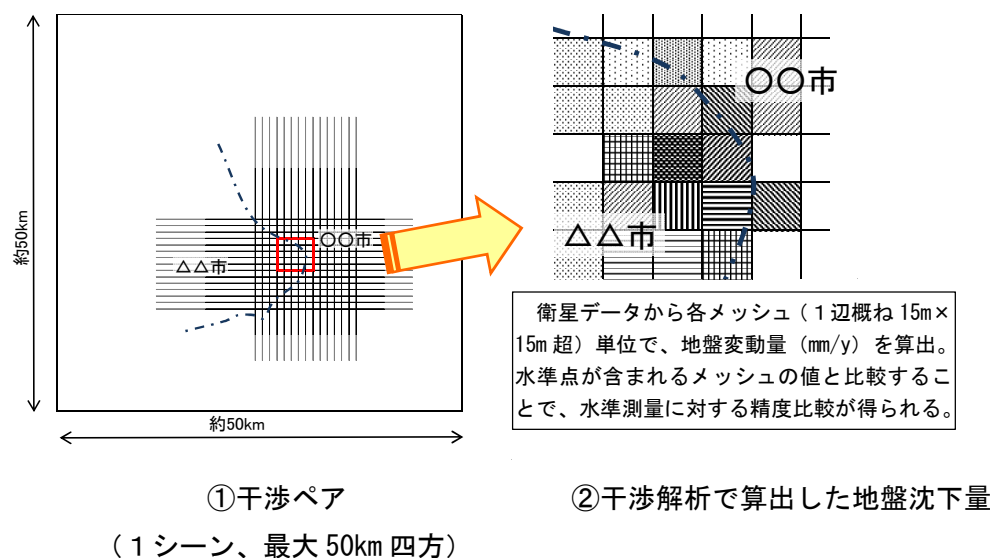
図 2-22 干渉 SAR 解析で算出される地盤変動量
