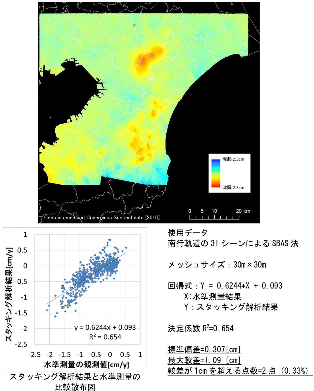
図 3-14 Sentinel-1 の南行軌道のスタッキング解析の精度検証結果
