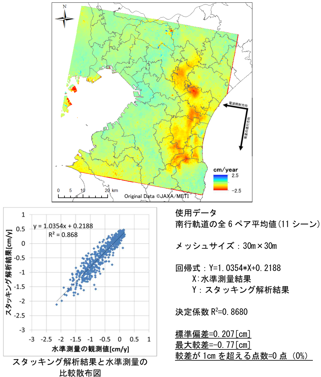
図 3-3 ALOS による南行軌道のスタッキング解析の精度検証結果
