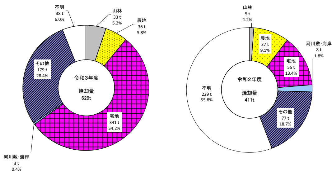
図 20.8 地目別野外焼却量
