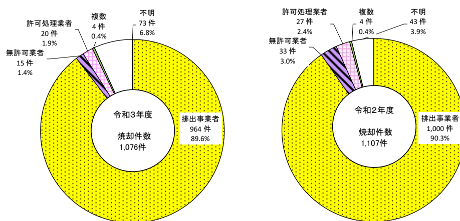
図 20.3 実行者別野外焼却件数
