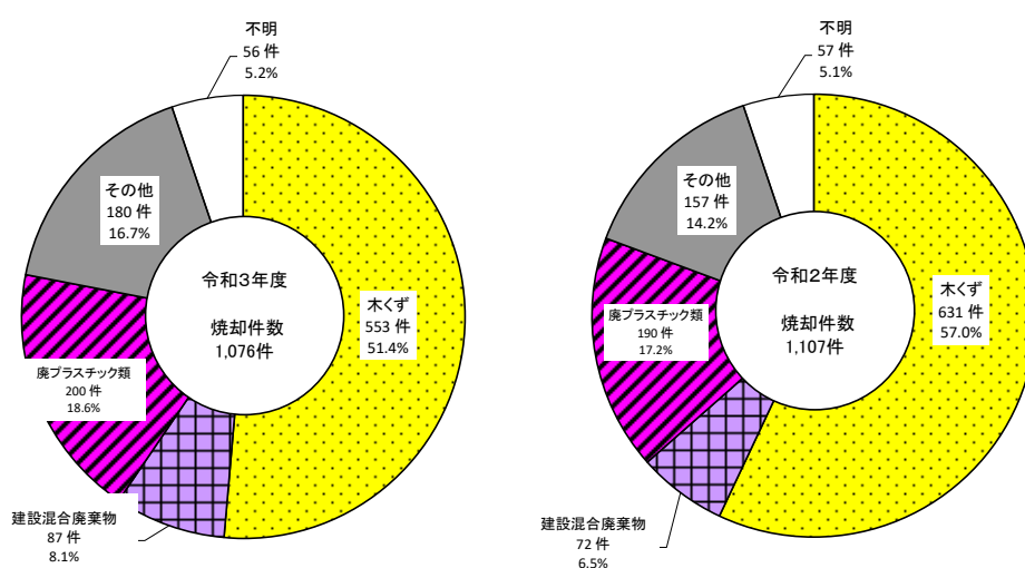
図 20.5 廃棄物の種類別野外焼却件数
