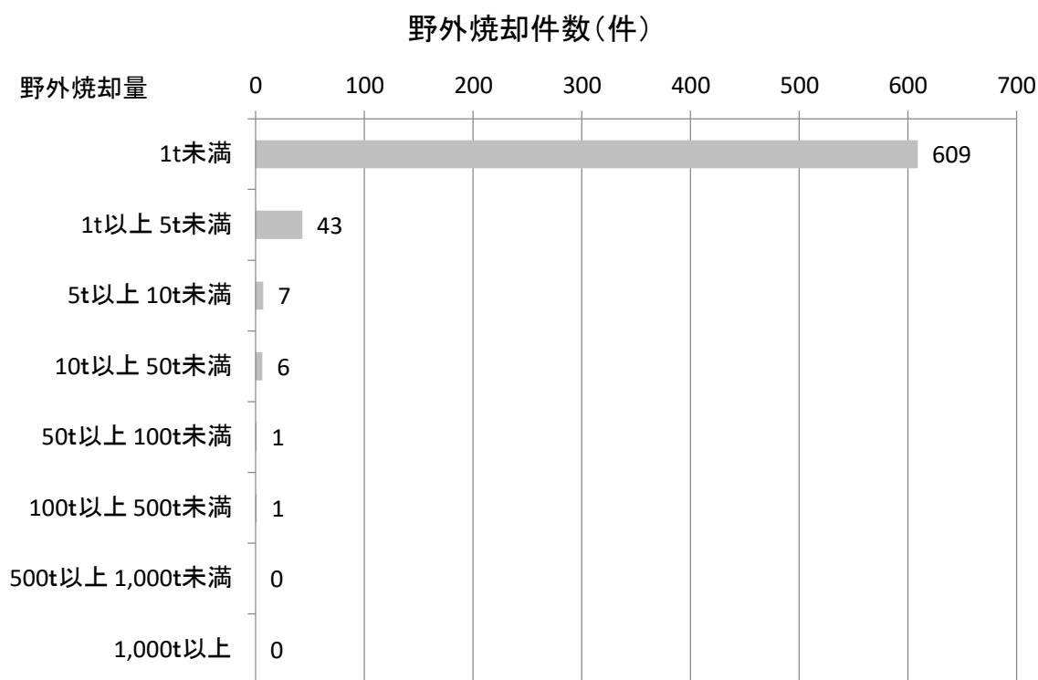
図 20.2 野外焼却量別の件数 (令和3年度)
