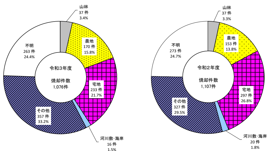
図 20.7 地目別野外焼却件数
