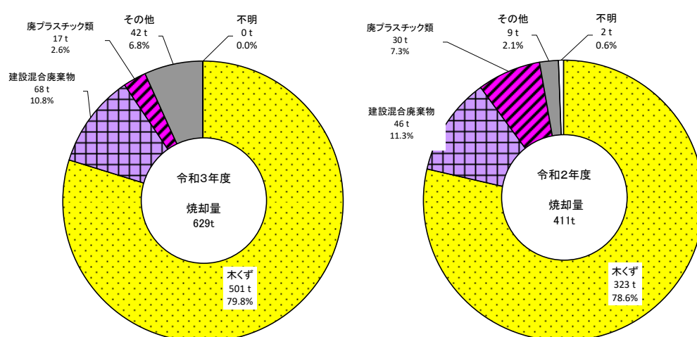
図 20.6 廃棄物の種類別野外焼却量
