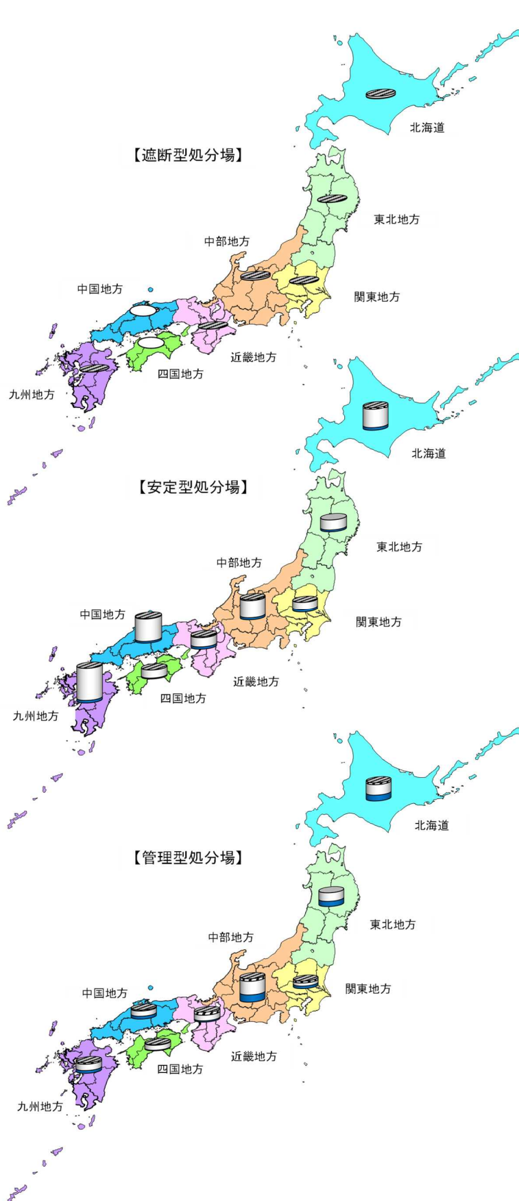
図 9.5 地域別最終処分場設置許可件数（令和 4 年 4 月 1 日現在）
