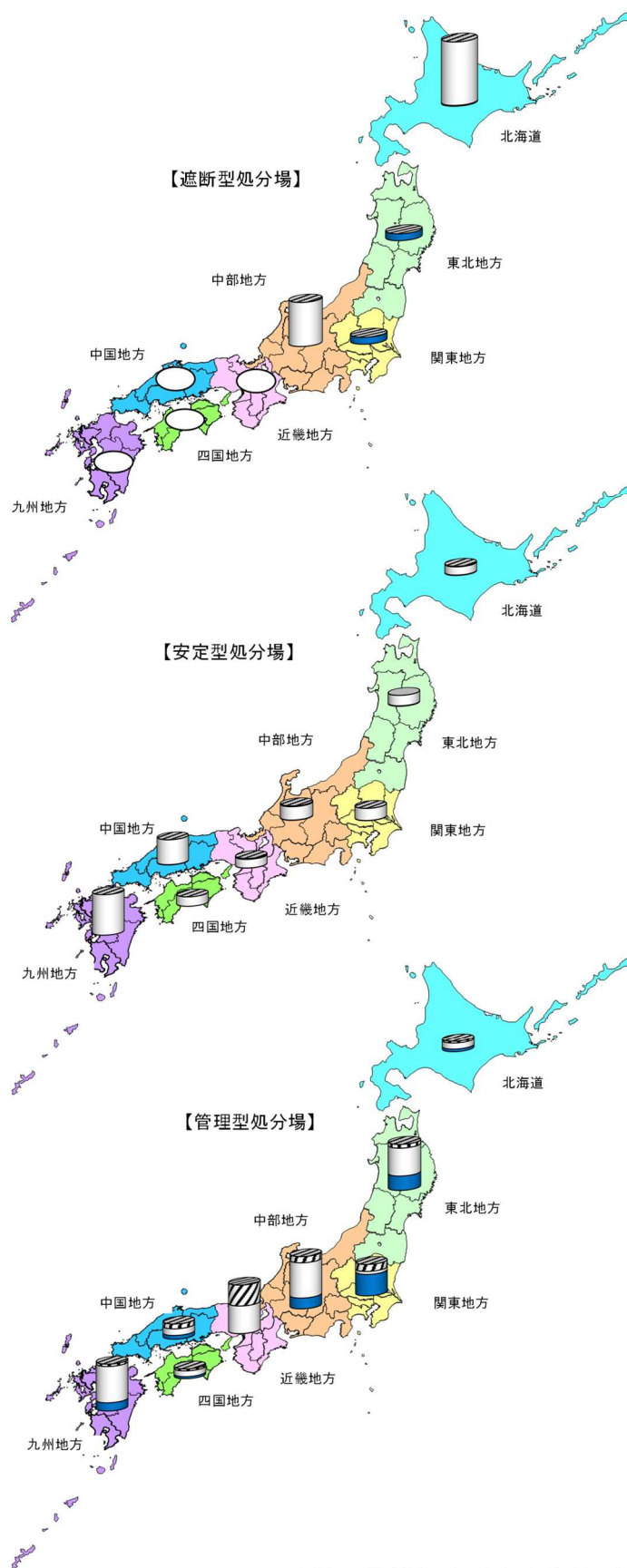
図 16.3 地域別最終処分場残存容量 (令和 4 年 4 月 1 日現在)
