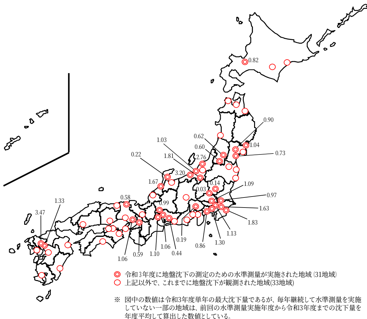
図1 令和3年度の全国の地盤沈下の状況 (cm/年) ※
