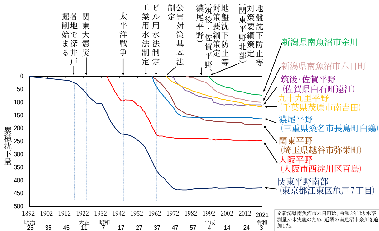
図9 代表的地域の地盤沈下の経年変化
