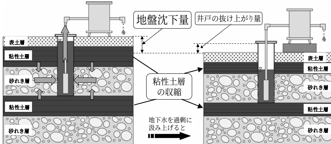
図7 地盤沈下のしくみと抜け上がり現象
