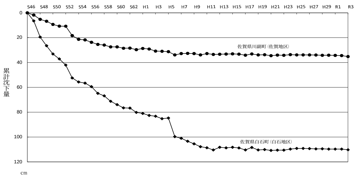
図14 地盤沈下の経年変化
