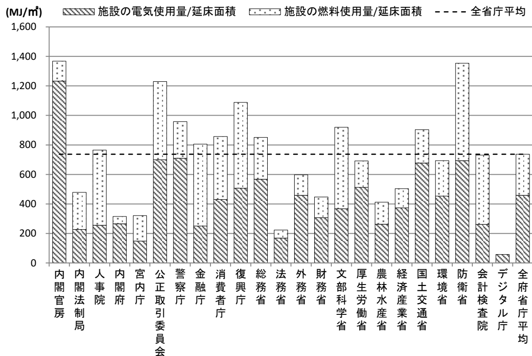
図 6.5.4 面積あたりのエネルギー消費量（施設の電気・燃料使用）（本府省庁）
