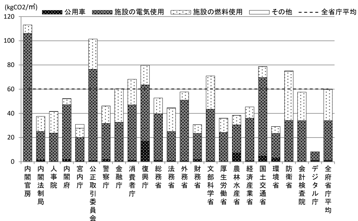
図 6.4.2 面積あたりの排出起源別温室効果ガス排出量（基礎排出係数）（省庁計）
