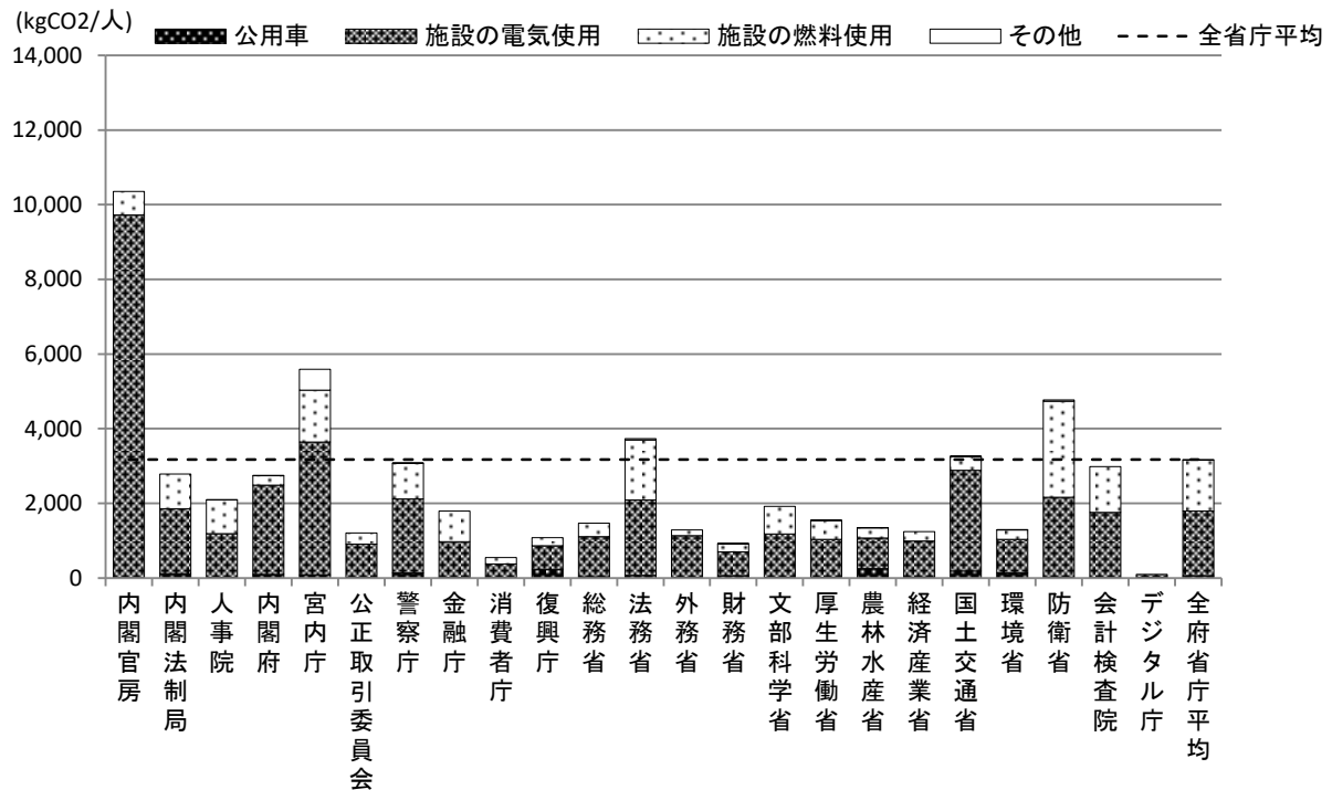
図 6.4.1 就業人数あたりの排出起源別温室効果ガス排出量（基礎排出係数）（省庁計）
