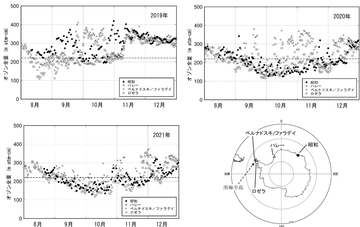
図1-資-9 南極域各国基地におけるオゾン全量の推移（2019年・2020年・2021年）
