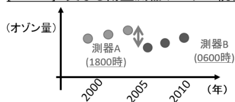
図1-資-4 オゾン量およびその長期トレンド推定に日周期変動が影響を与える例
