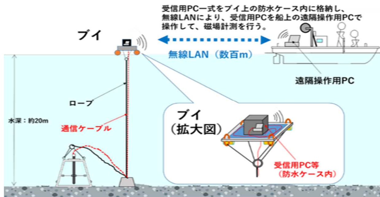
○電磁探査システムイメージ図
