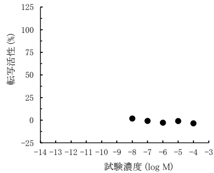
n-ヘキサン
