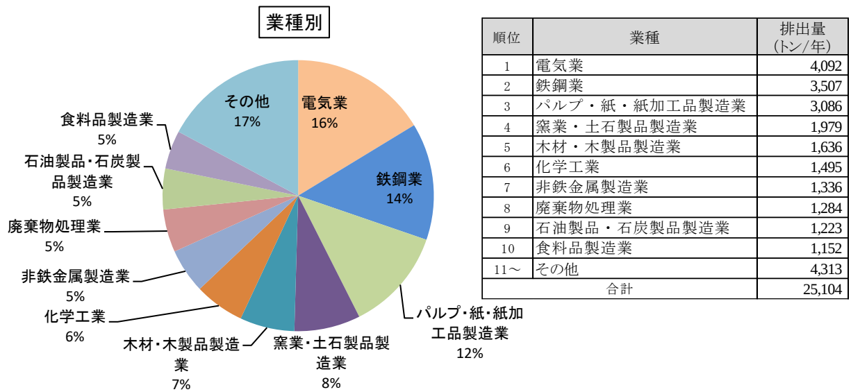
図 6 業種別のばいじん排出量内訳 (総排出量: 25,104 トン/年) (平成 29 年度速報値)
