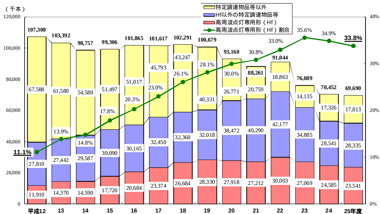
図3-15 高周波点灯専用形 (Hf) の国内出荷量及び割合
