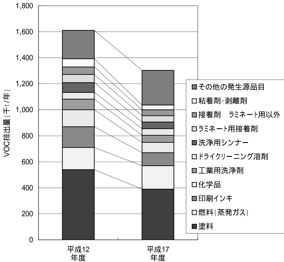
図2 全国の揮発性有機化合物（VOC）排出量の発生源別構成比
