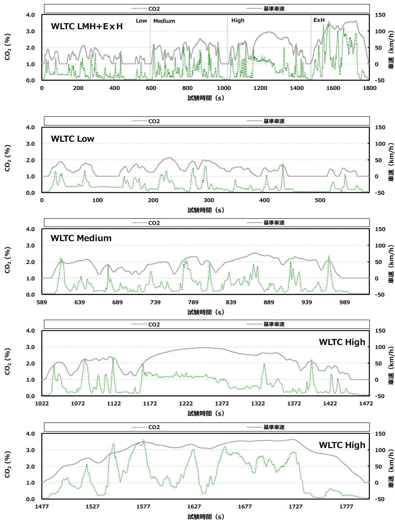
付録図 10.2 ② 認証重質化の CO 2 排出挙動 (A 車)
