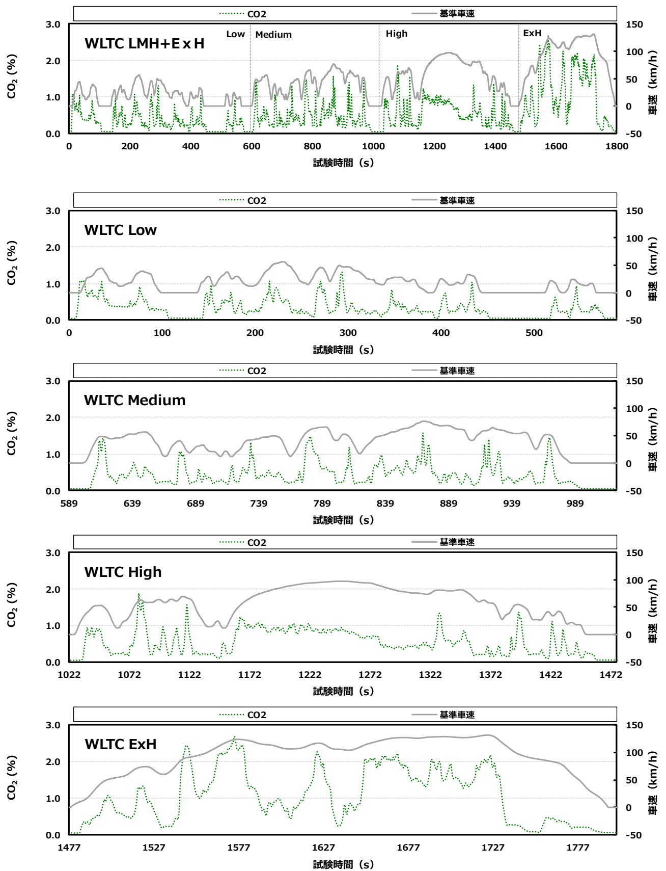
付録図 10.5 ② 認証重質化の CO 2 排出挙動 (B 車)
