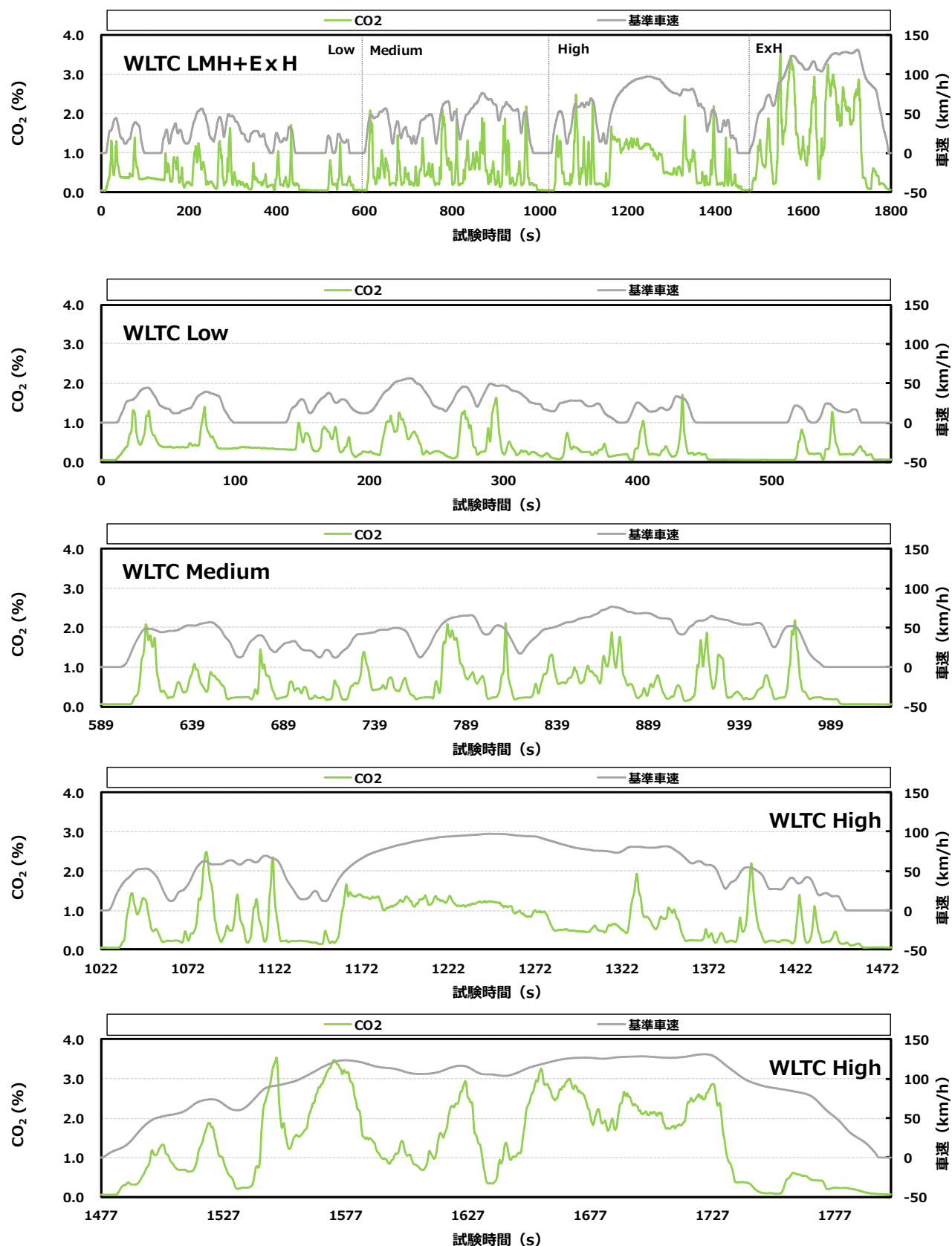
付録図 10.1 ① 認証試験用の CO 2 排出挙動 (A 車)
