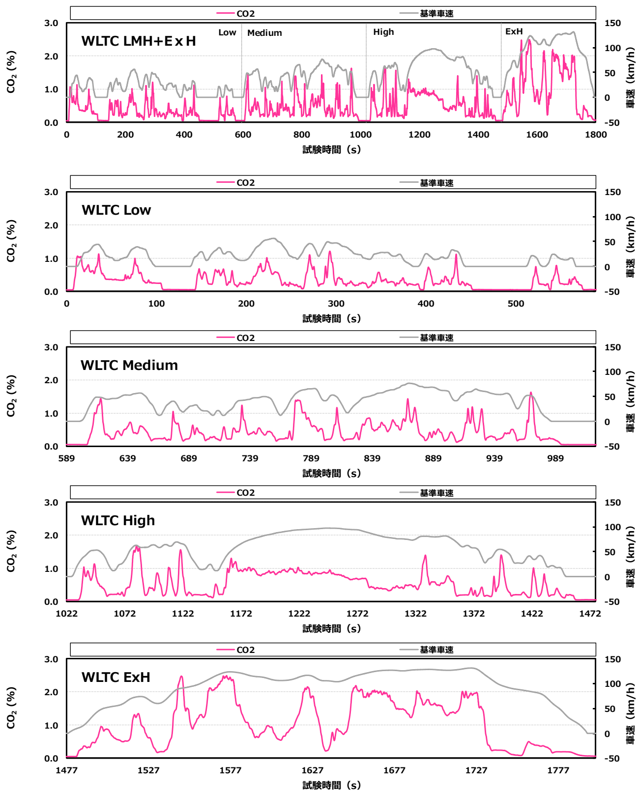
付録図 10.6 ③ 市井重質の CO 2 排出挙動 (B 車)
