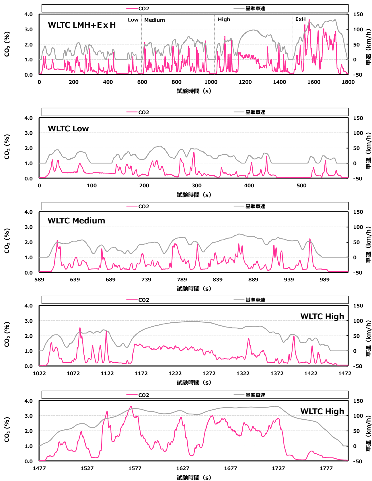
付録図 10.3 ③ 市井重質の CO 2 排出挙動 (A 車)
