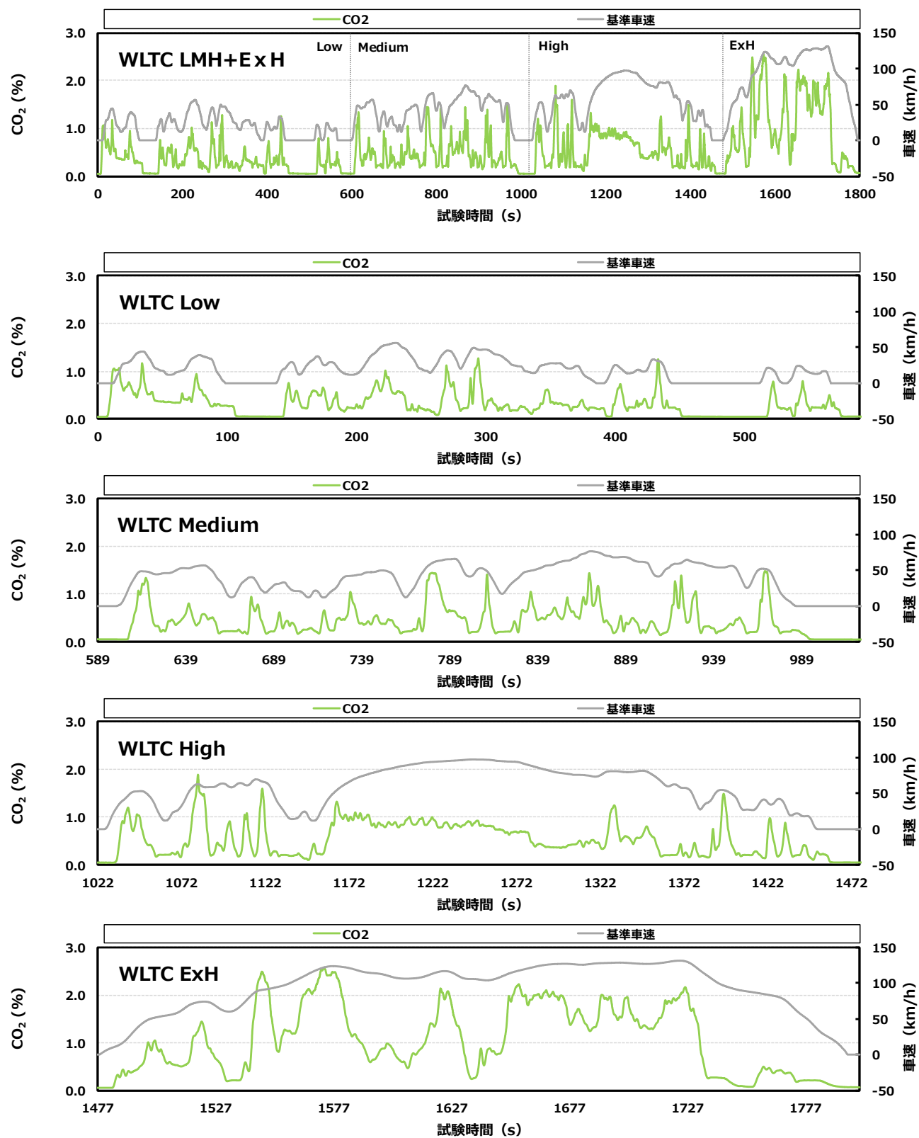
付録図 10.4 ① 認証試験用の CO 2 排出挙動 (B 車)
