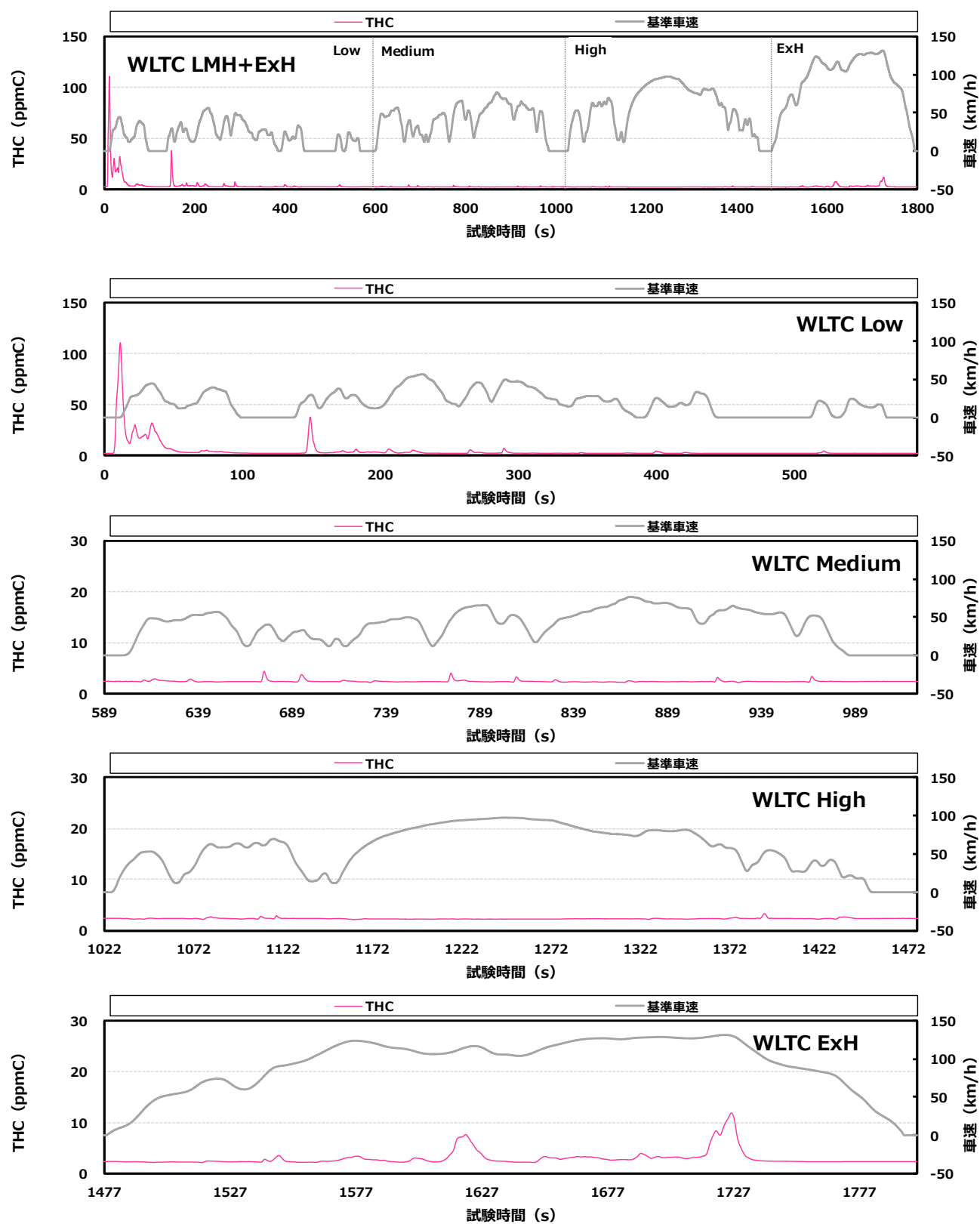
付録図 8.6 ③ 市井重質の THC 排出挙動 (B 車)
