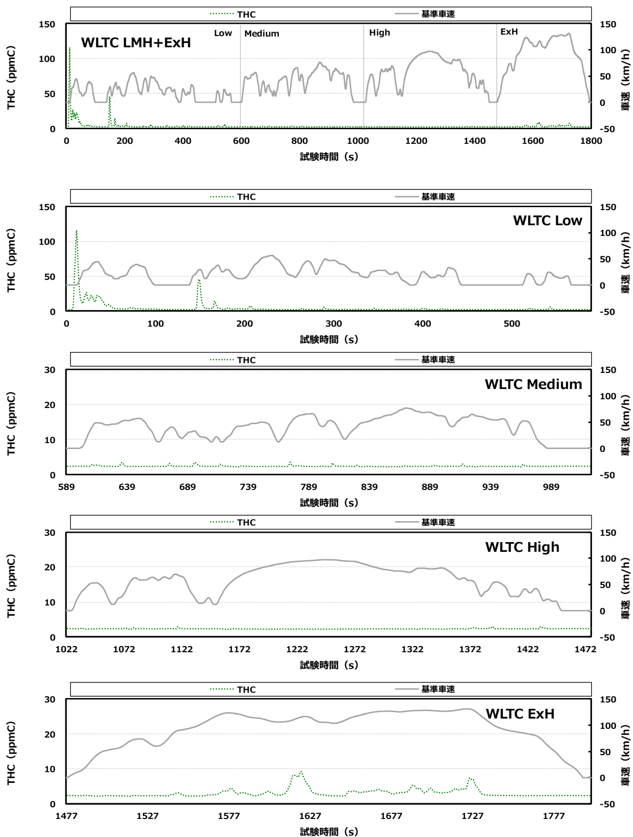
付録図 8.5 ② 認証重質化の THC 排出挙動 (B 車)
