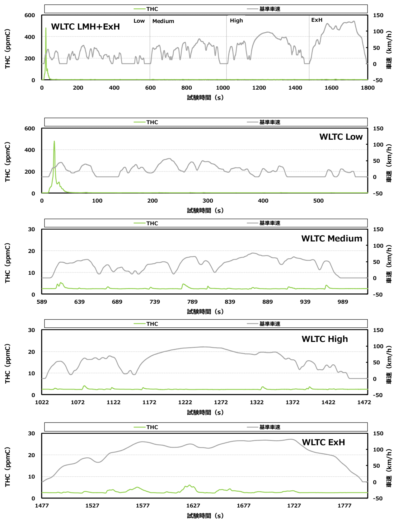
付録図 8.1 ① 認証試験用の THC 排出挙動 (A 車)
