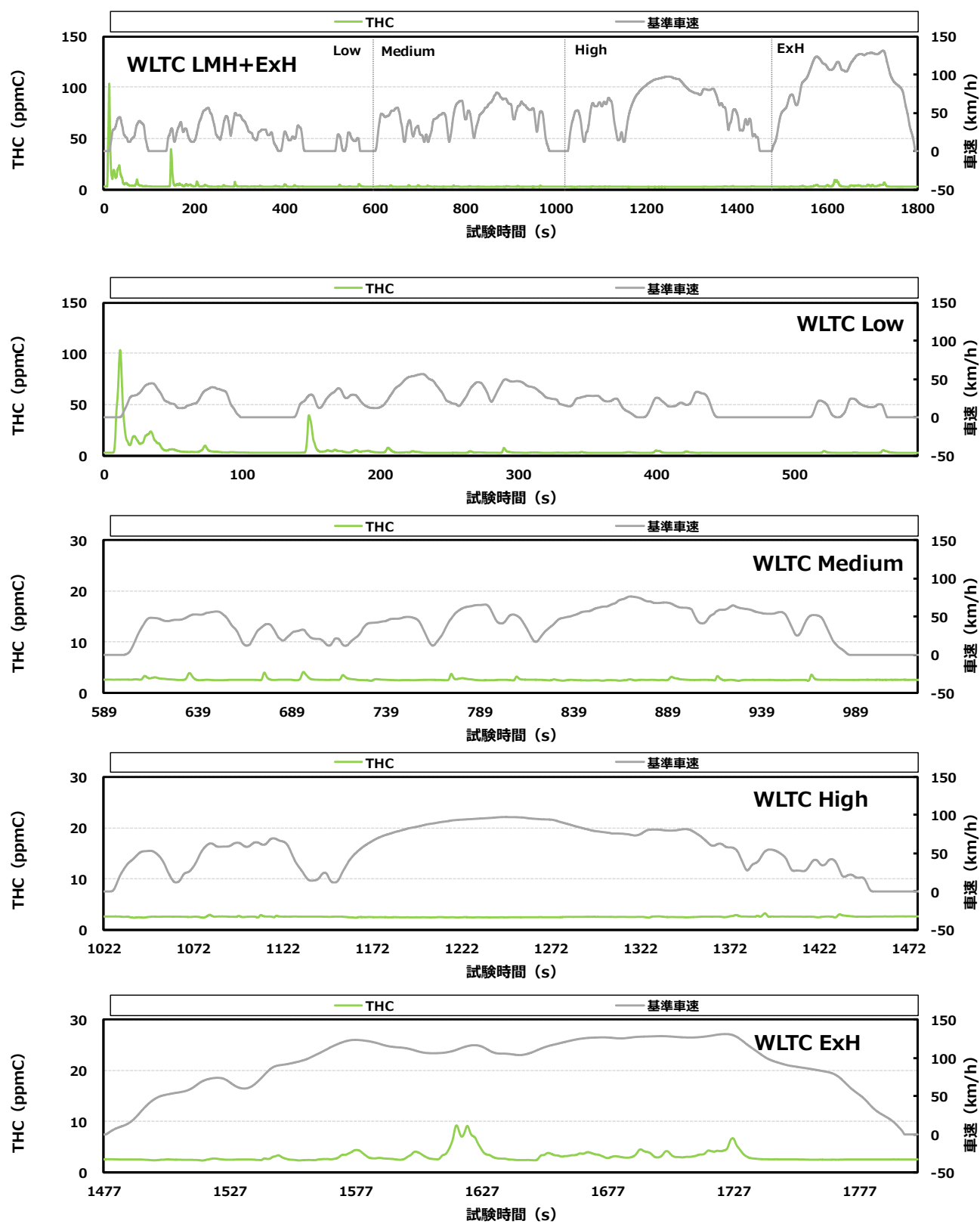
付録図 8.4 ① 認証試験用の THC 排出挙動 (B 車)
