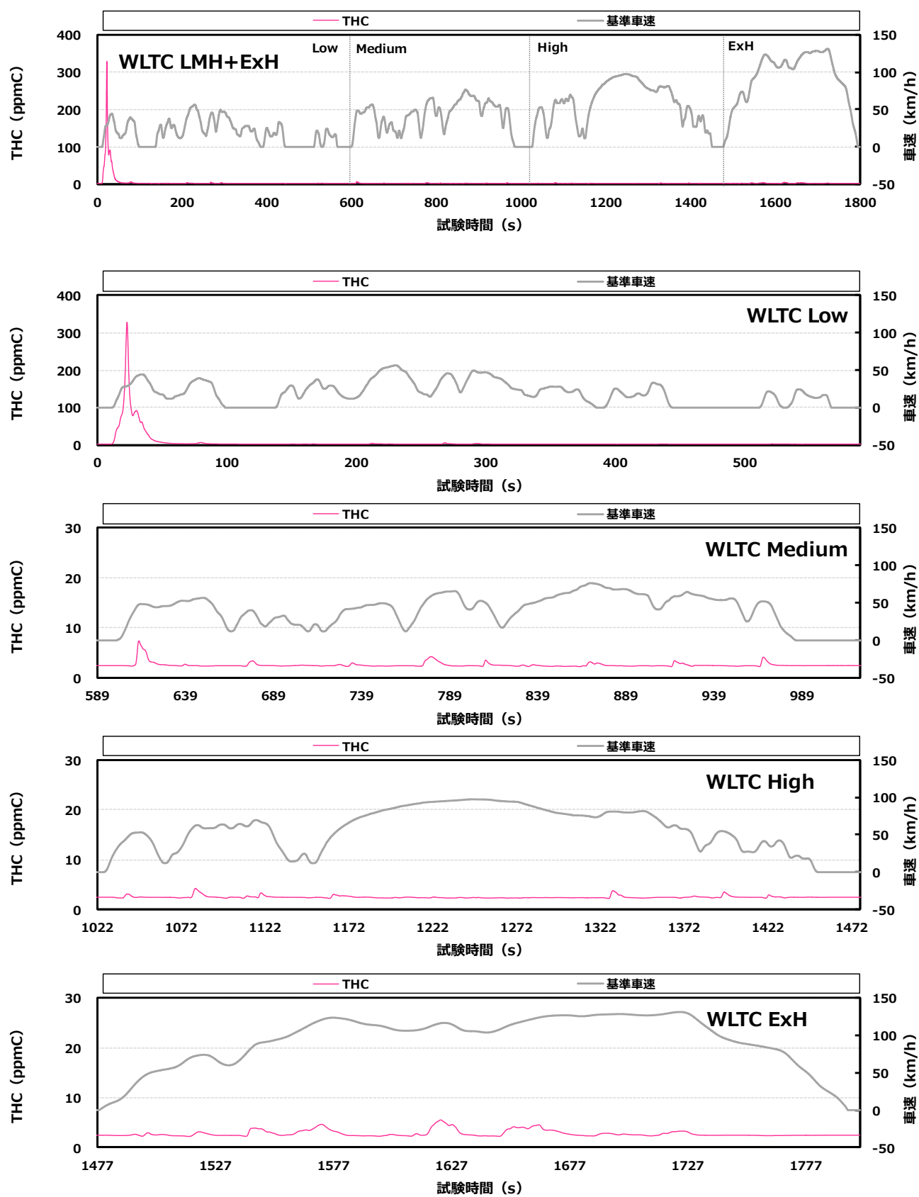
付録図 8.3 ③ 市井重質の THC 排出挙動 (A 車)
