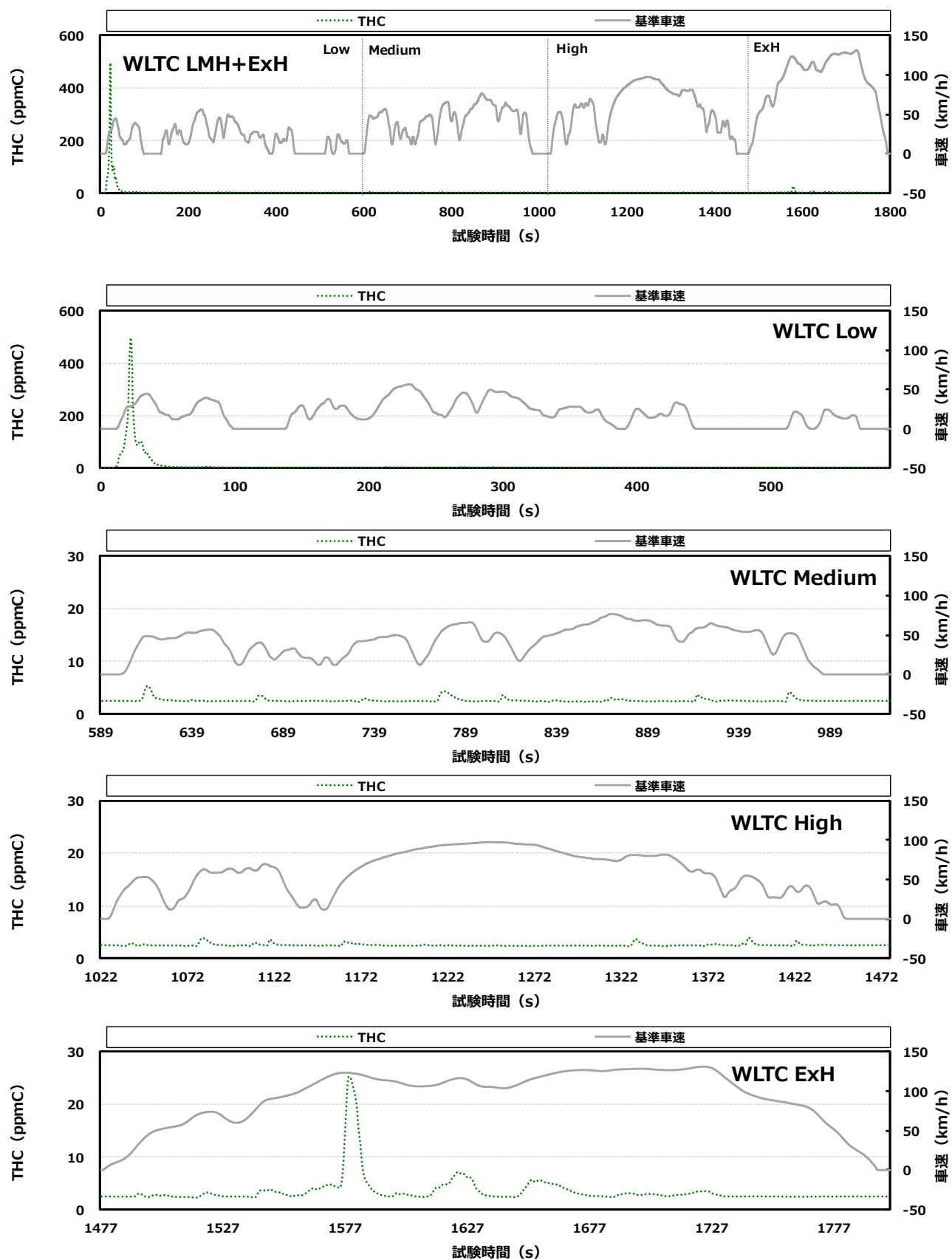
付録図 8.2 ② 認証重質化の THC 排出挙動 (A 車)
