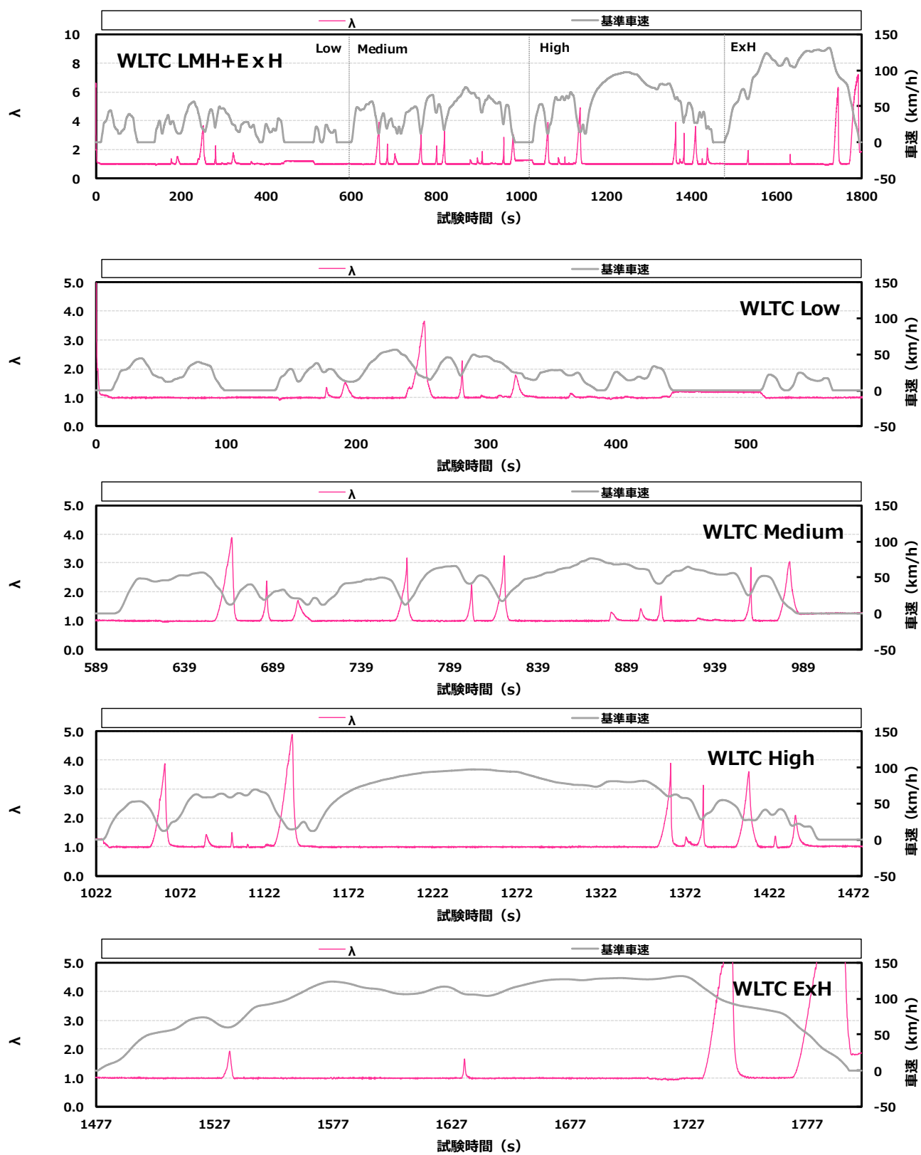
付録図 7.6 ③ 市井重質の挙動 (B 車)
