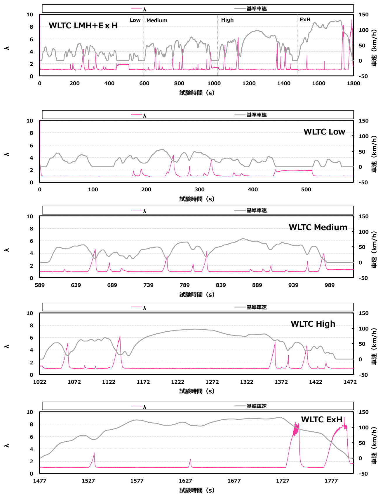
付録図 7.3 ③ 市井重質の挙動 (A 車)
