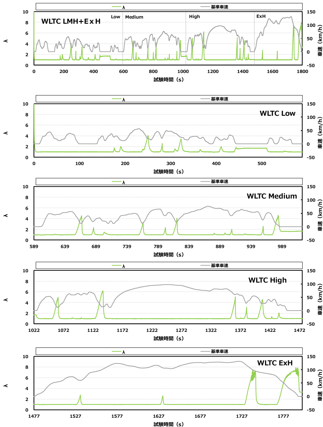
付録図 7.1 ① 認証試験用の 挙動 (A 車)
