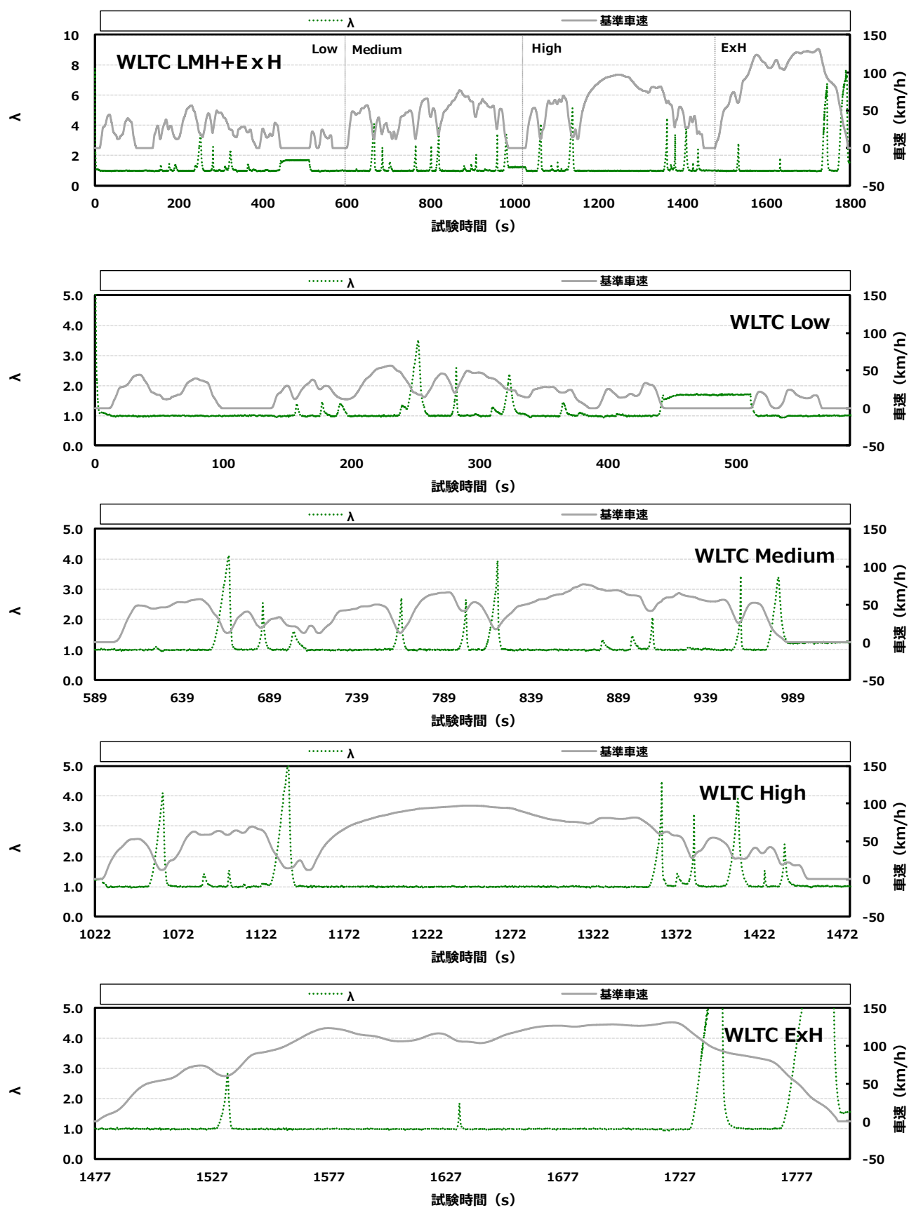
付録図 7.5 ② 認証重質化の挙動 (B 車)
