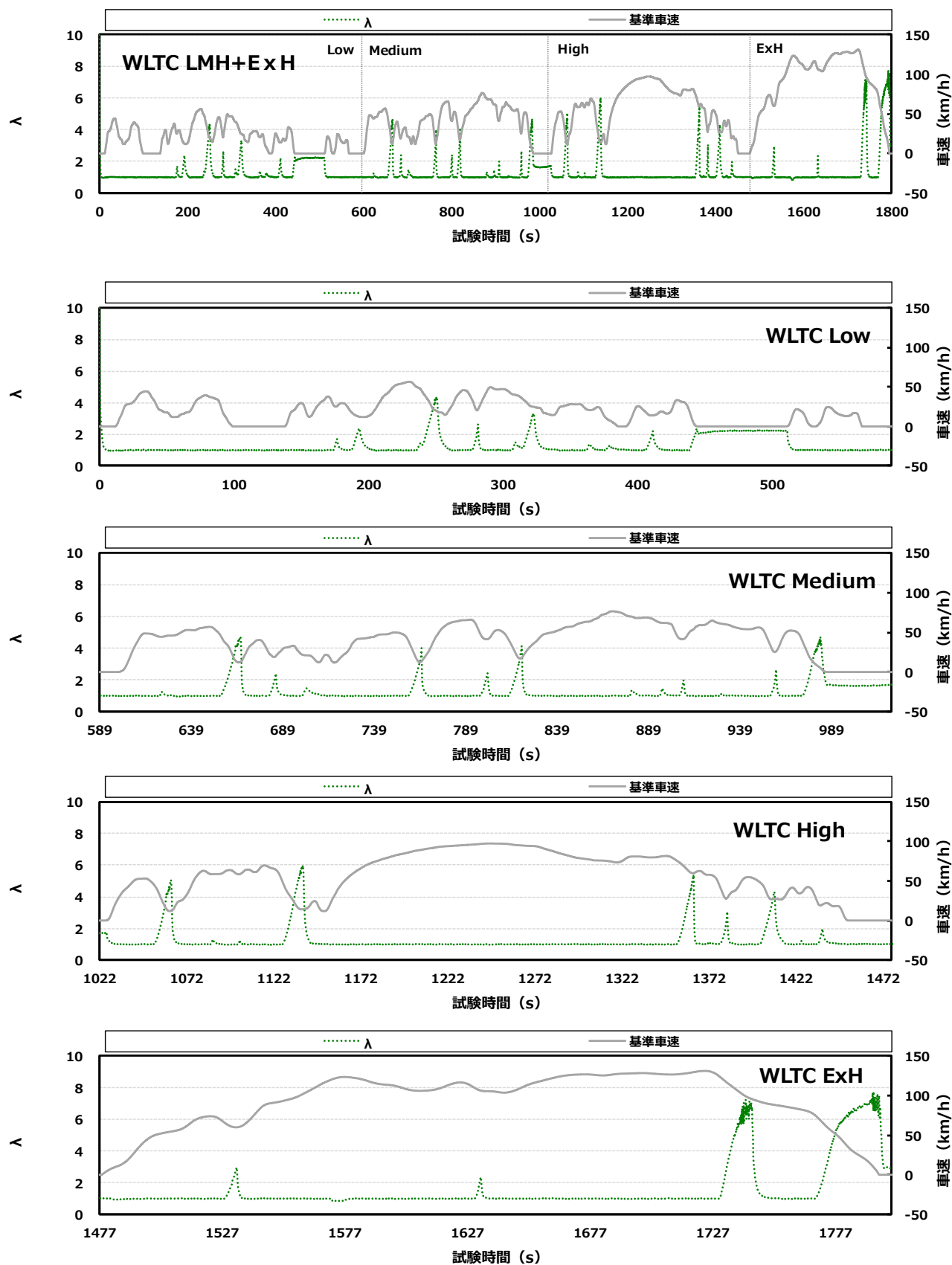
付録図 7.2 ② 認証重質化の 挙動 (A 車)
