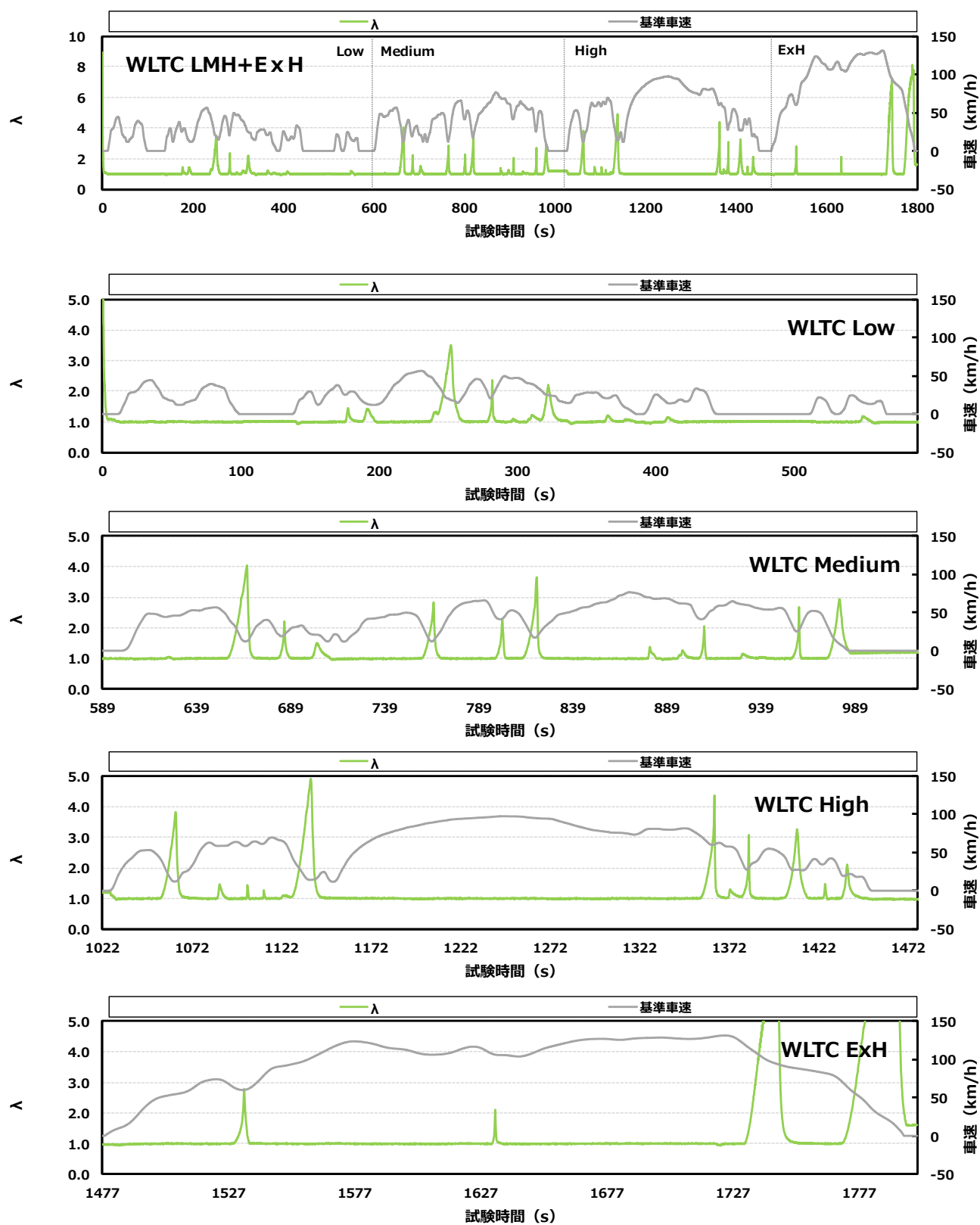
付録図 7.4 ① 認証試験用の 挙動 (B 車)
