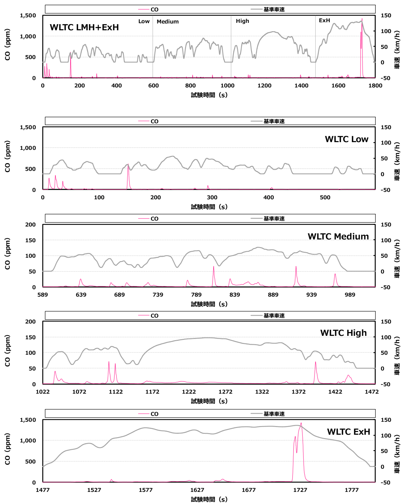
付録図 6.6 ③ 市井重質の CO 排出挙動 (B 車)
