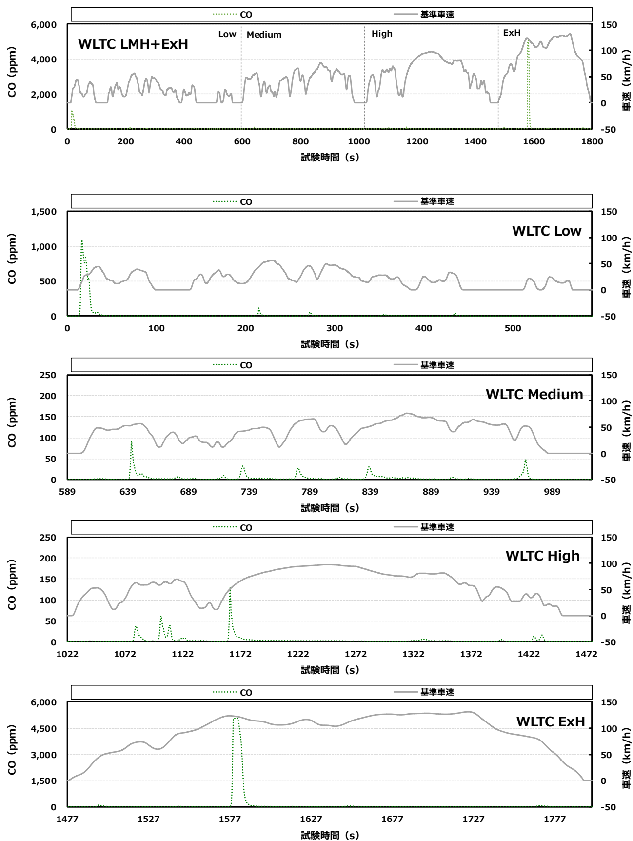
付録図 6.2 ② 認証重質化の CO 排出挙動 (A 車)
