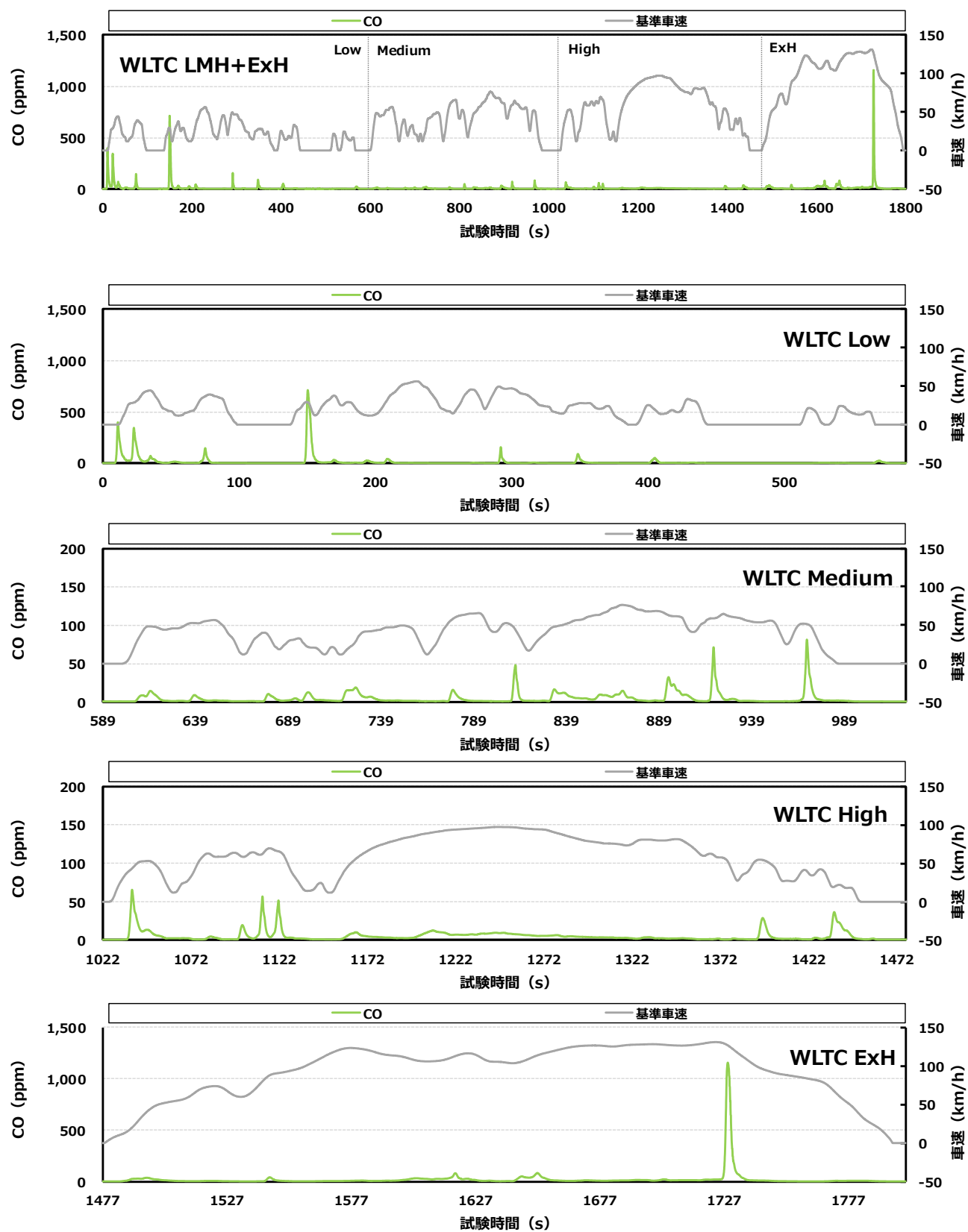
付録図 6.4 ① 認証試験用の CO 排出挙動 (B 車)
