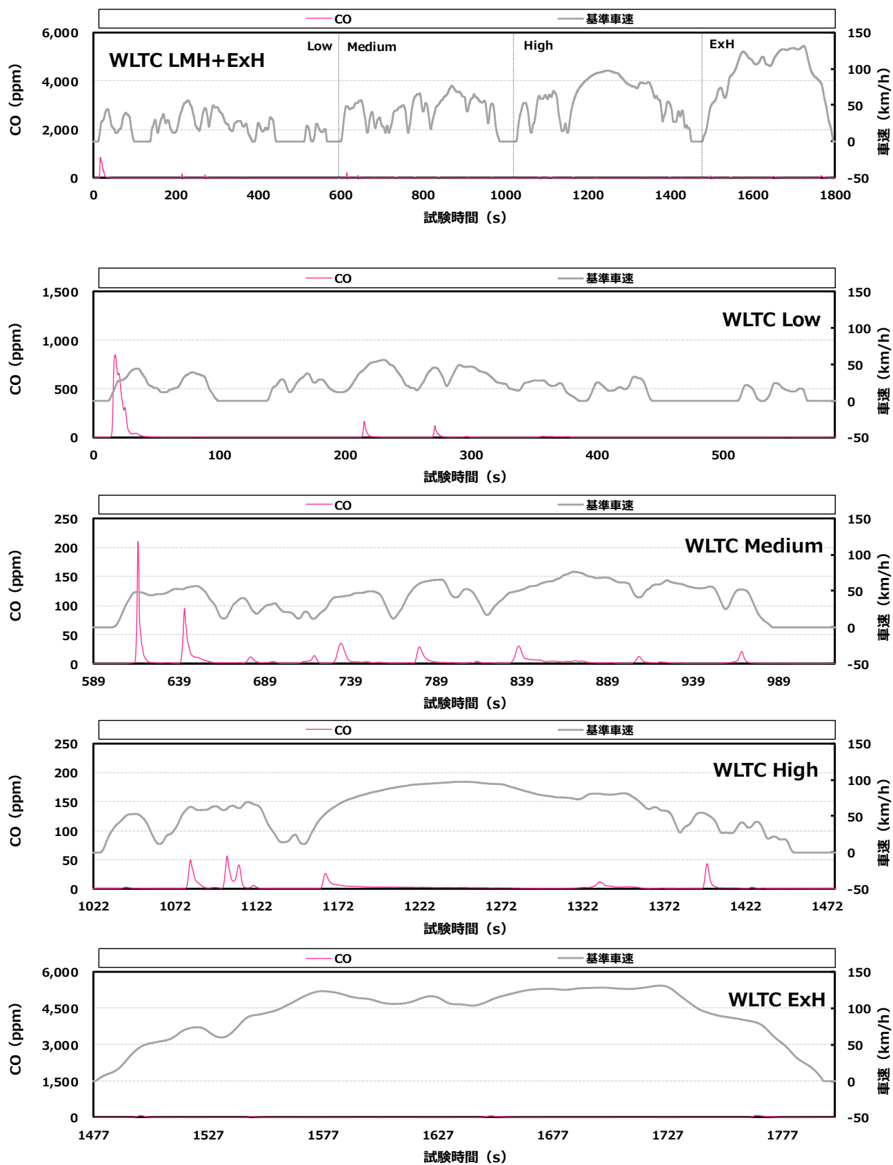
付録図 6.3 ③ 市井重質の CO 排出挙動 (A 車)
