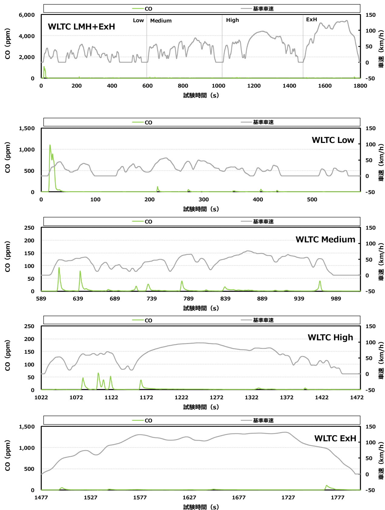
付録図 6.1 ① 認証試験用の CO 排出挙動 (A 車)
