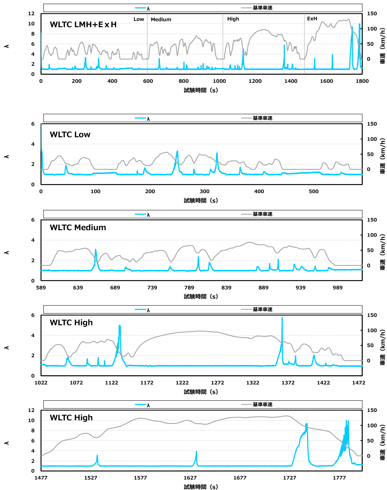
付録図 10.4 ④ 認証試験用 P の挙動 (D 車)
