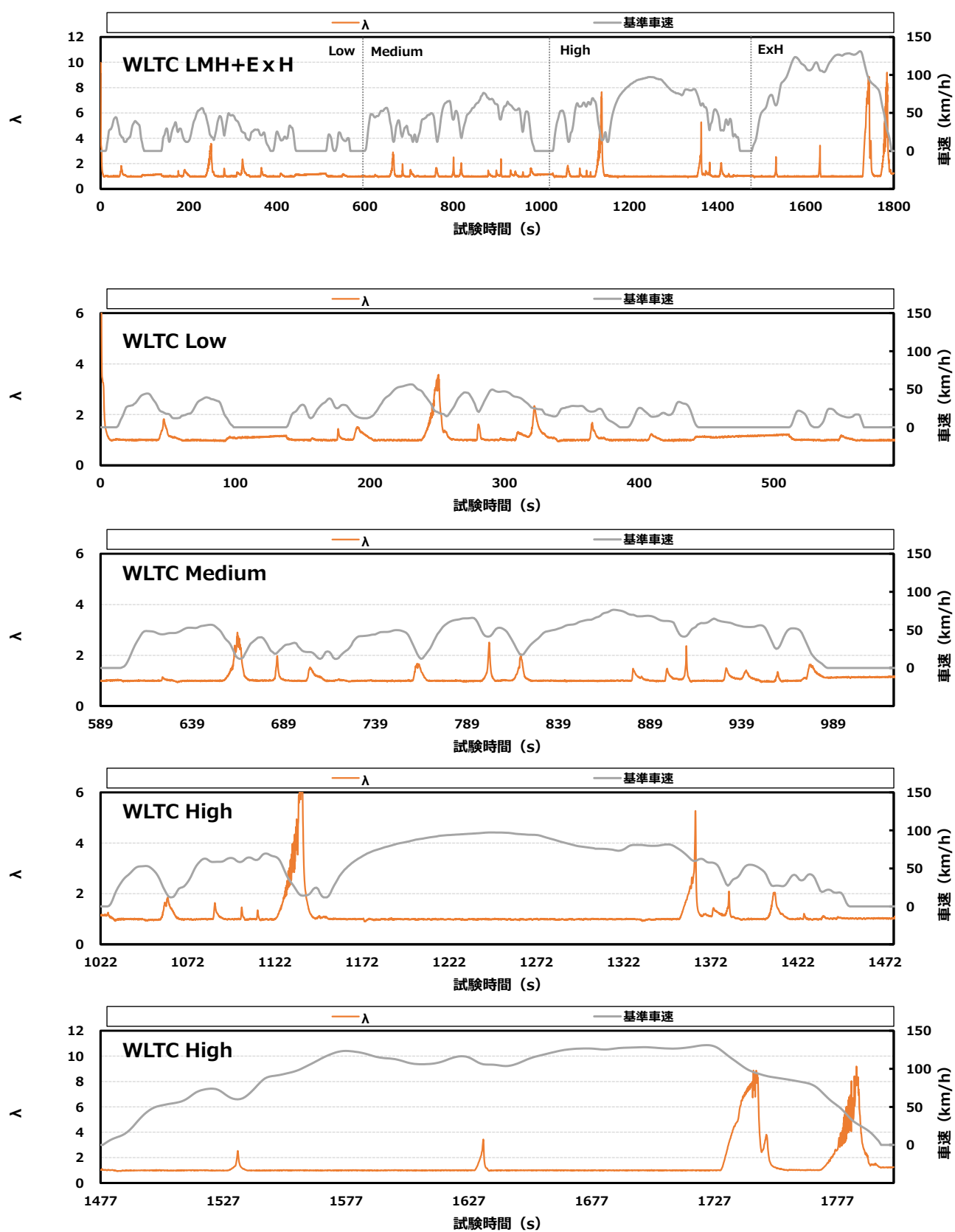
付録図 10.6 ⑥ 市井相当の挙動 (D 車)
