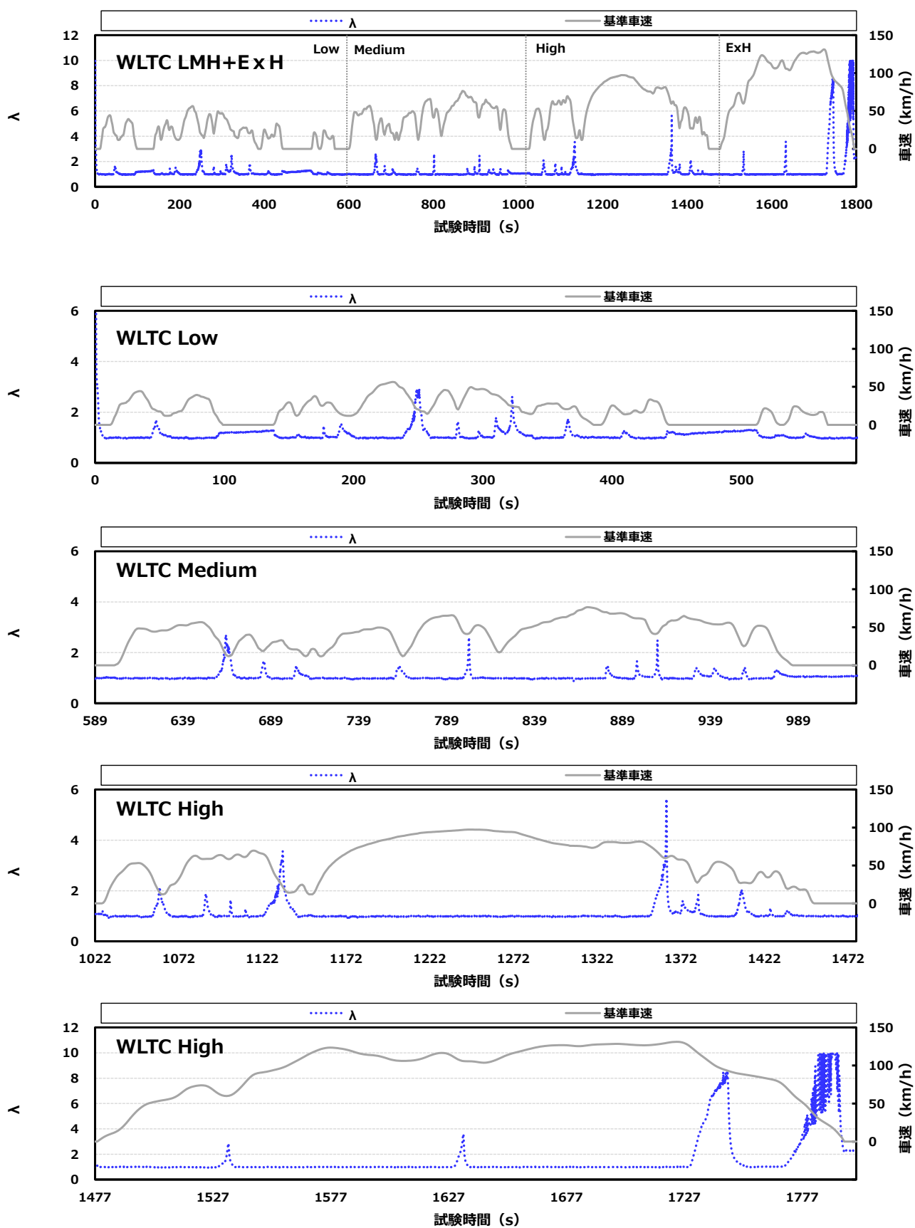
付録図 10.5 ⑤ 認証重質化Pの挙動 (D車)
