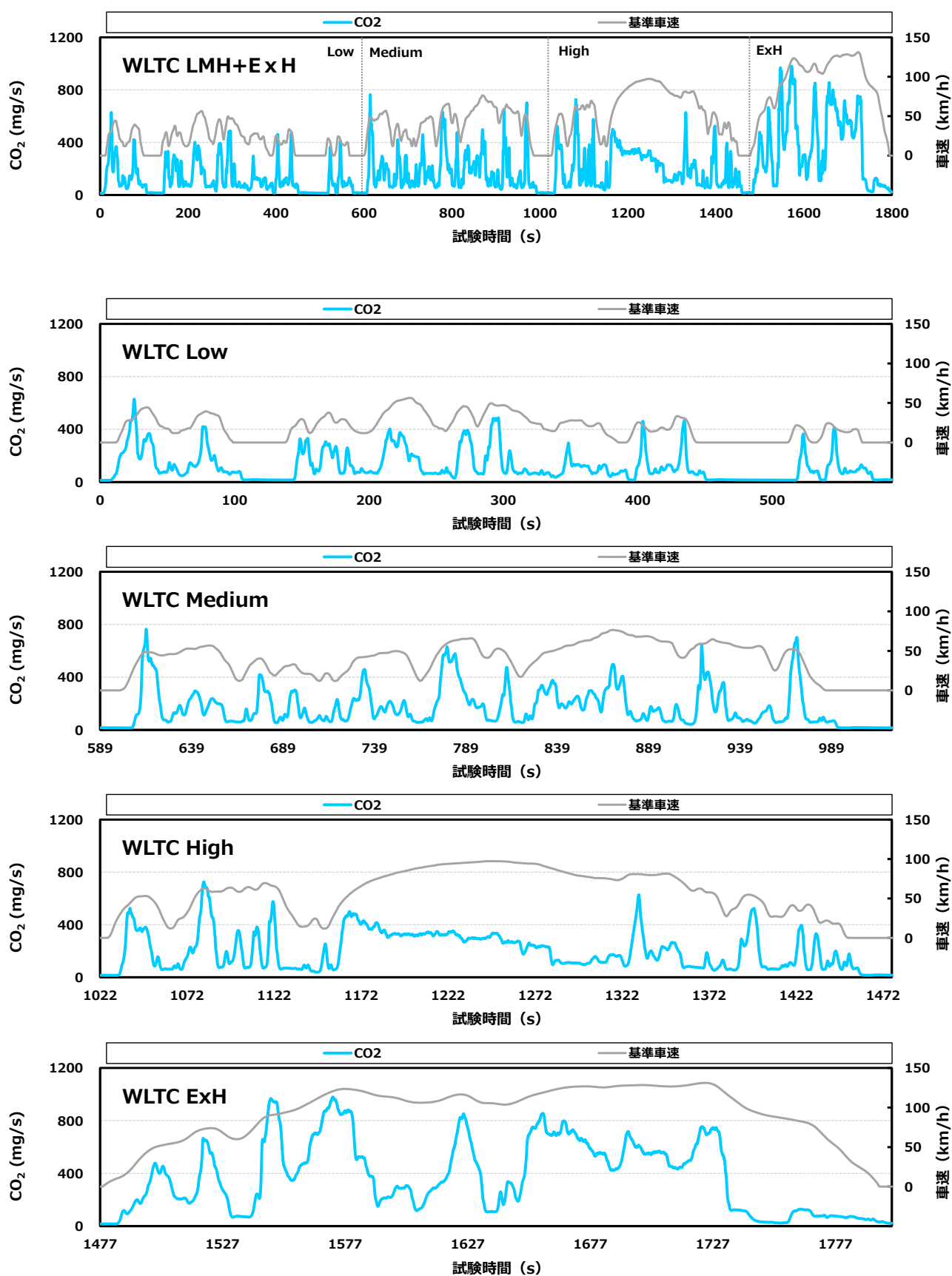
付録図 9.4 ④ 認証試験用の CO 2 排出挙動 (D 車)
