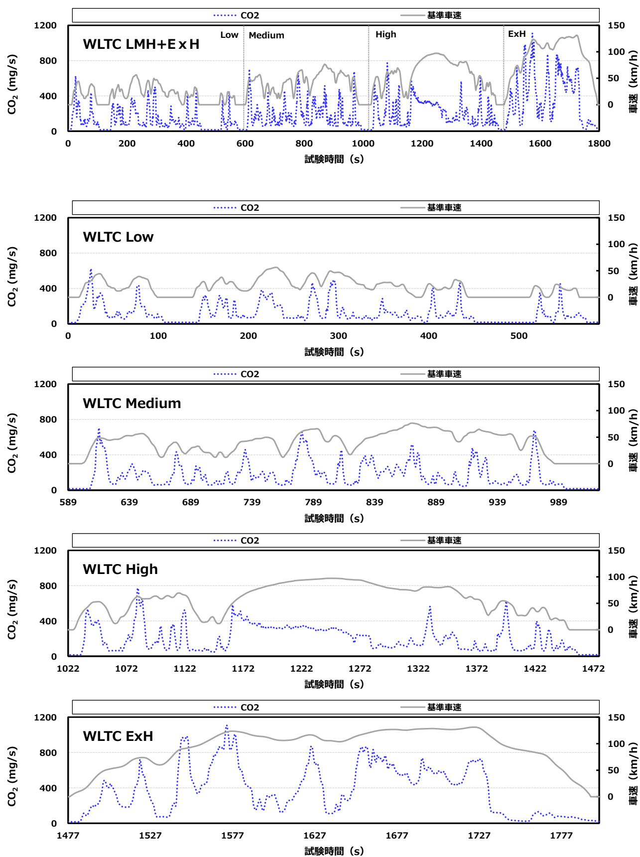
付録図 9.5 ⑤ 認証重質化PのCO 2 排出挙動 (D車)
