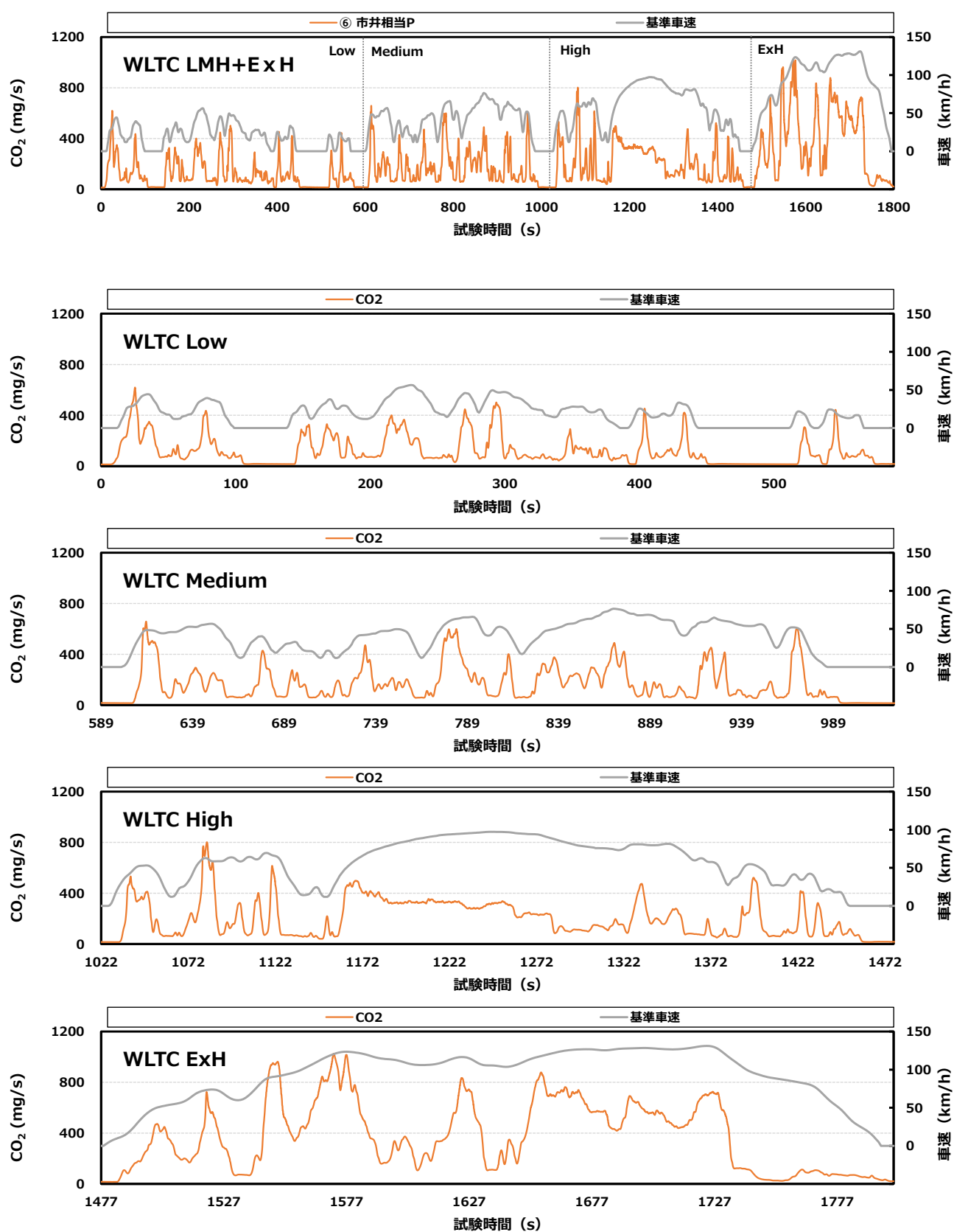
付録図 9.6 ⑥ 市井相当PのCO 2 排出挙動 (D車)
