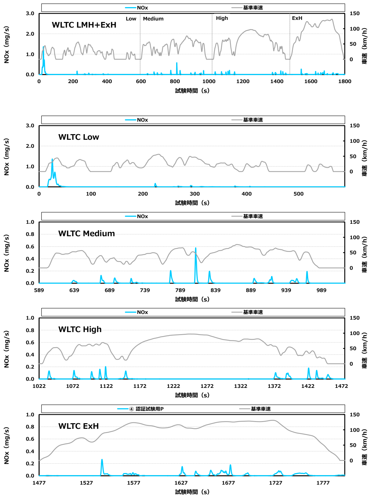
付録図 8.1 ④ 認証試験用 P の NO x 排出挙動 (C 車)
