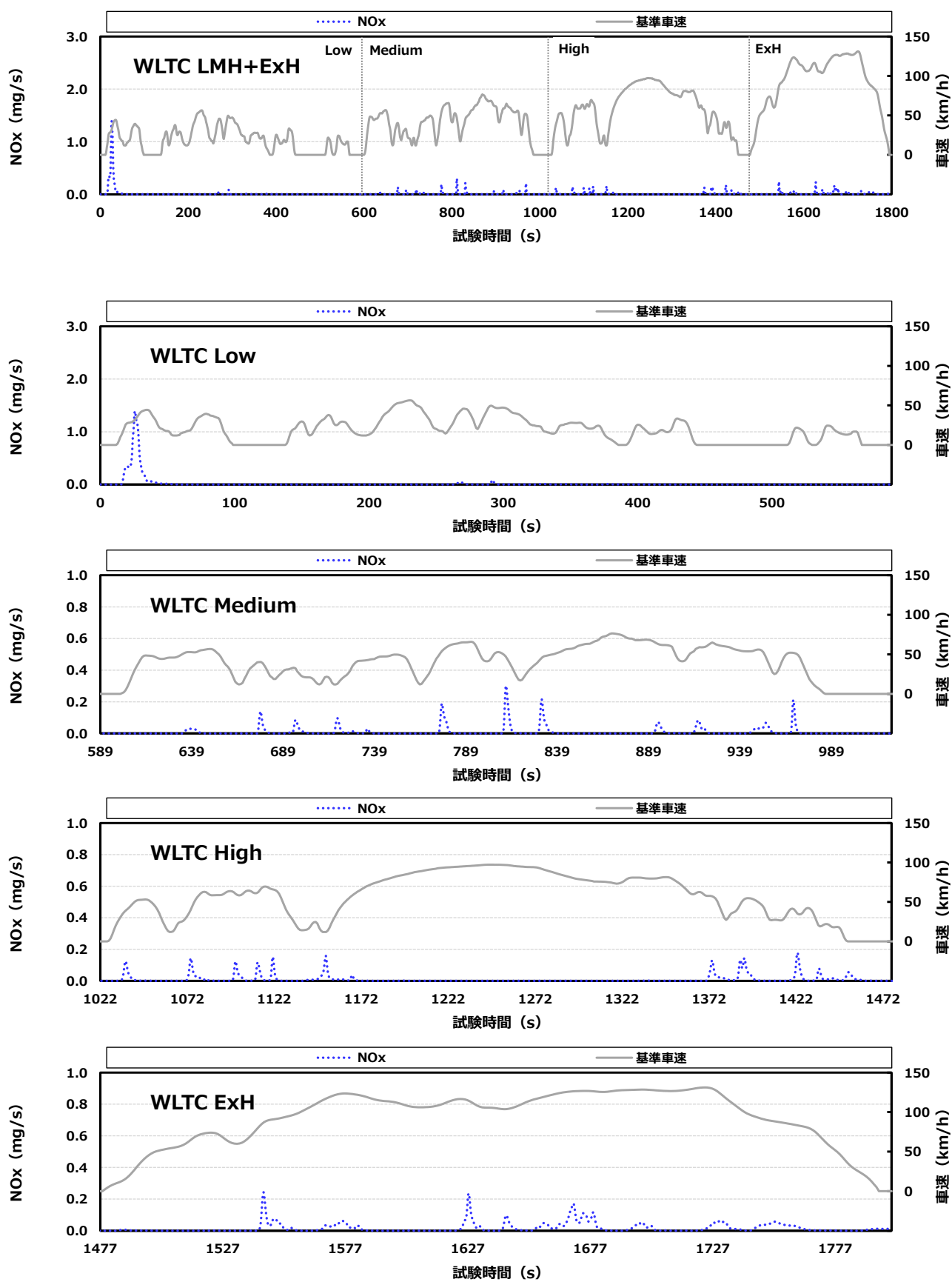
付録図 8.2 ⑤ 認証重質化 P の NOx 排出挙動 (C 車)
