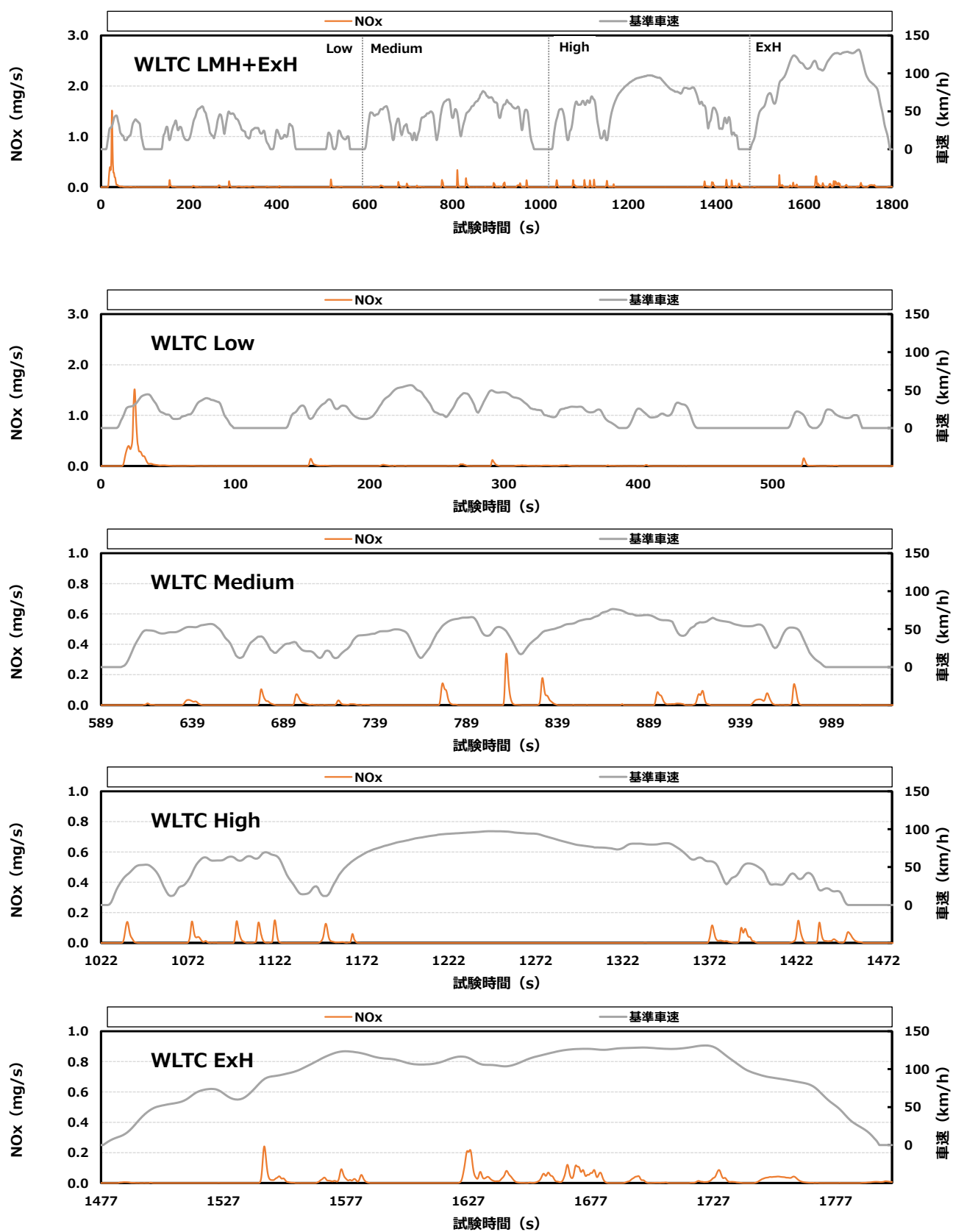
付録図 8.3 ⑥ 市井相当の NOx 排出挙動 (C 車)
