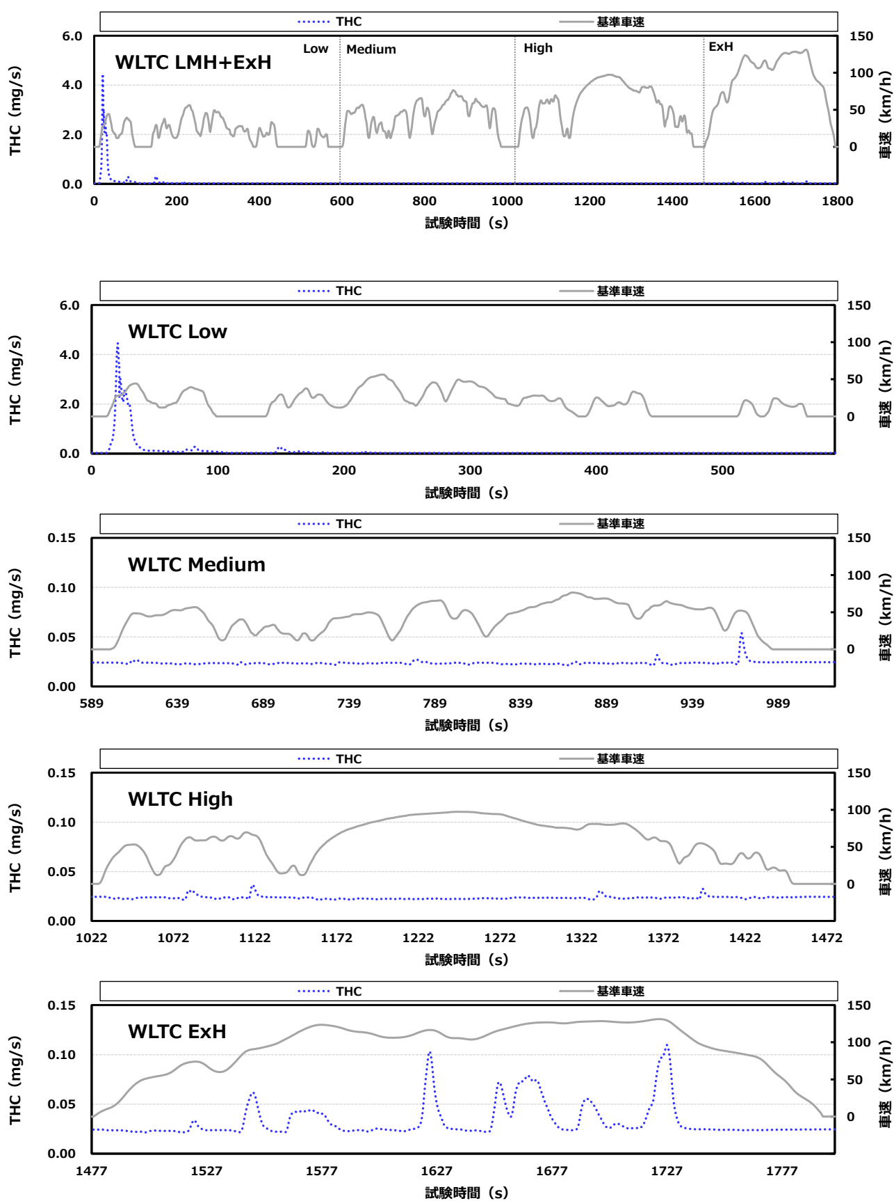
付録図 7.2 ⑤ 認証重質化 P の THC 排出挙動 (C 車)
