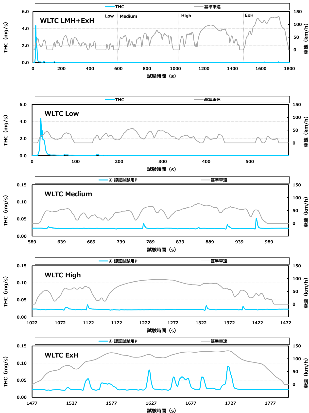
付録図 7.1 ④ 認証試験用 P の THC 排出挙動 (C 車)
