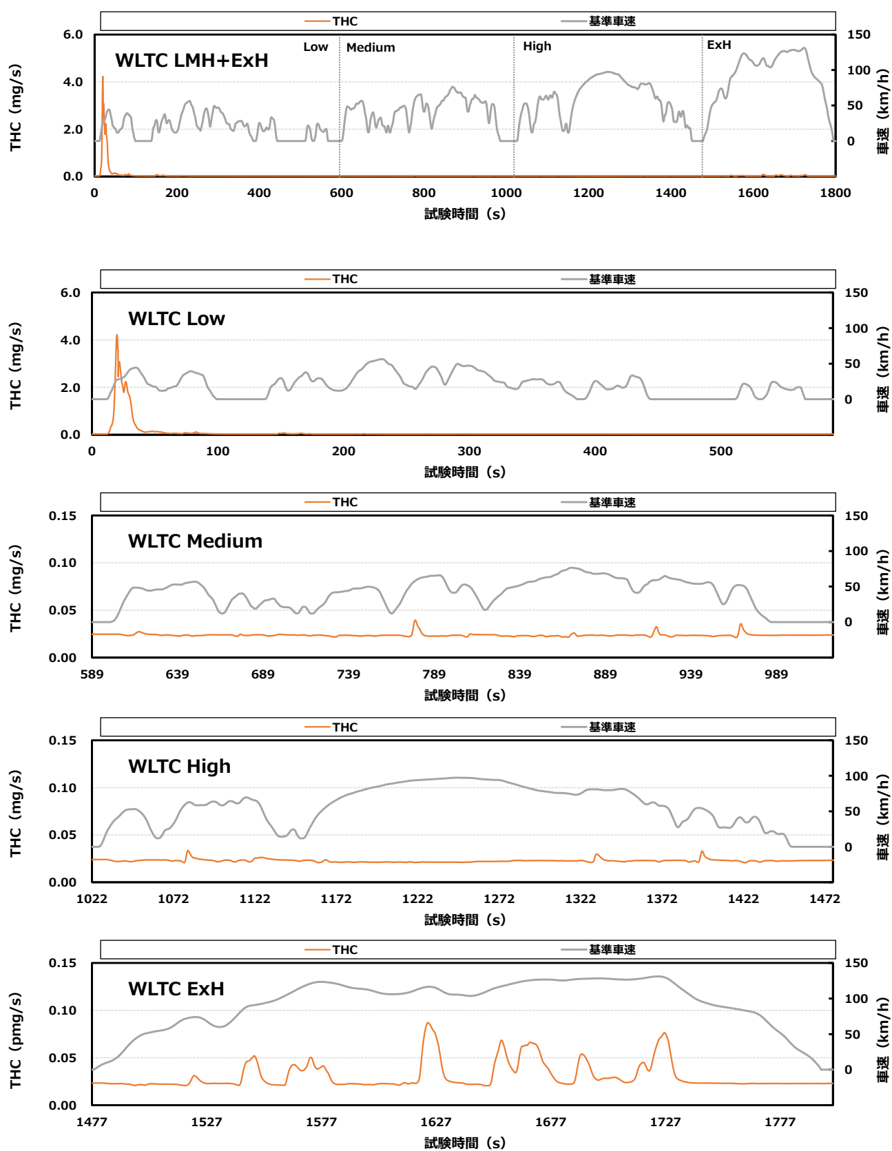
付録図 7.3 ⑥ 市井相当の THC 排出挙動 (C 車)
