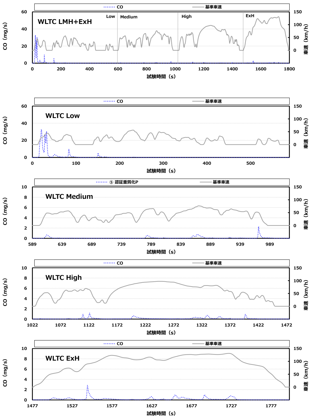
付録図 6.2 ⑤ 認証重質化PのCO排出挙動 (C車)
