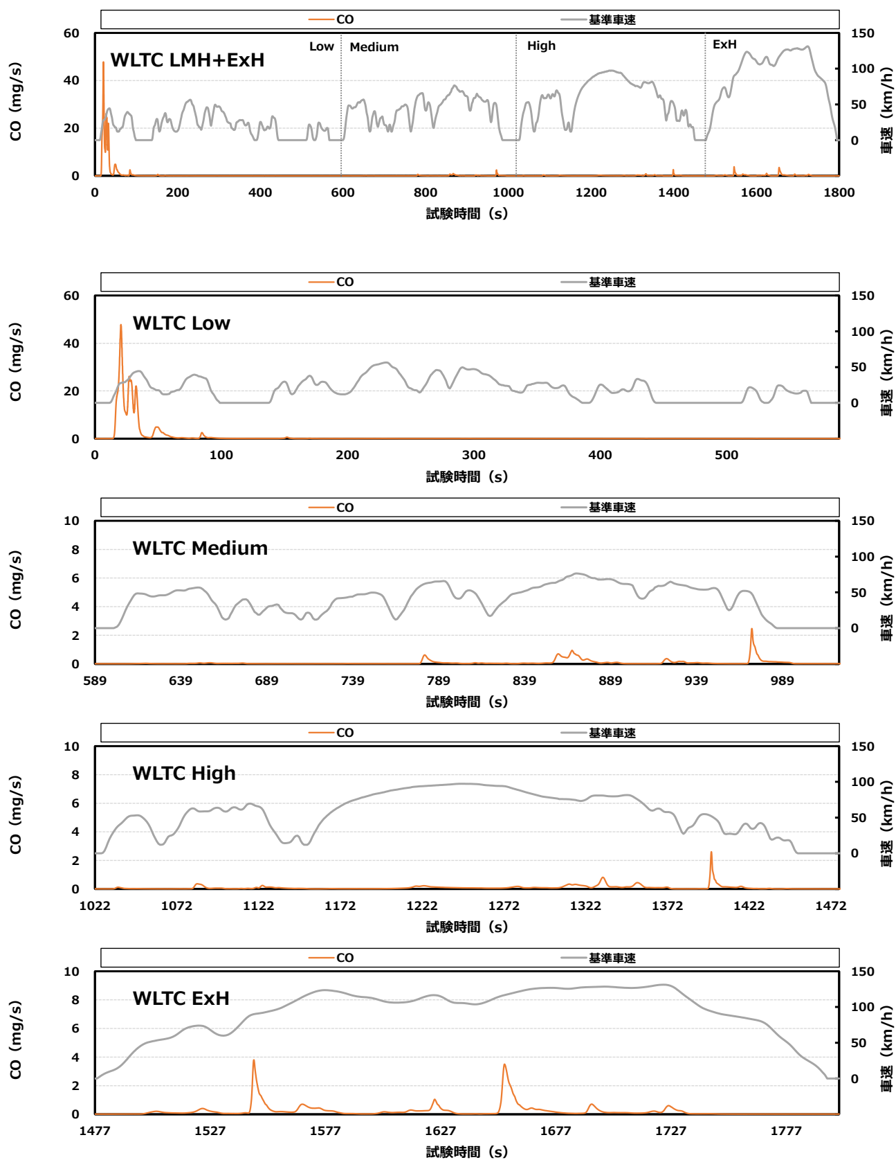
付録図 6.3 ⑥ 市井相当 P の CO 排出挙動 (C 車)
