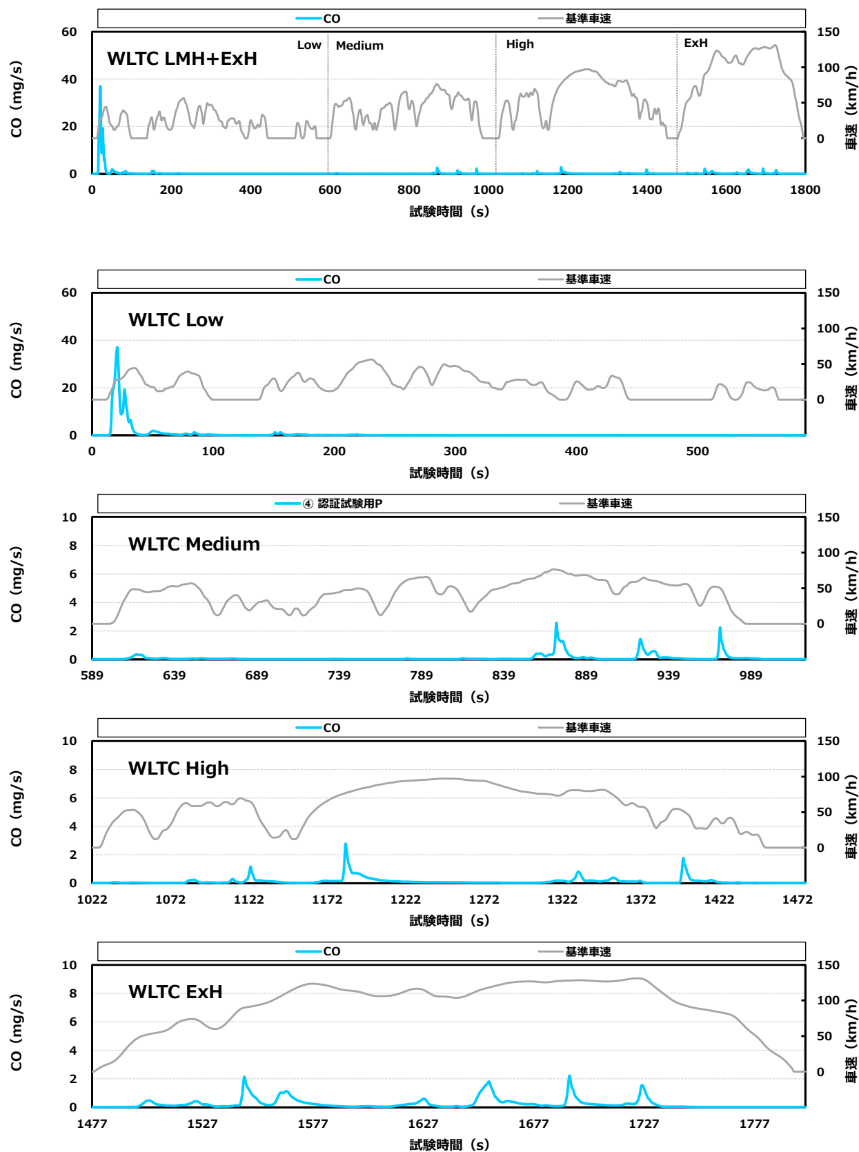
付録図 6.1 ④ 認証試験用 P の CO 排出挙動 (C 車)
