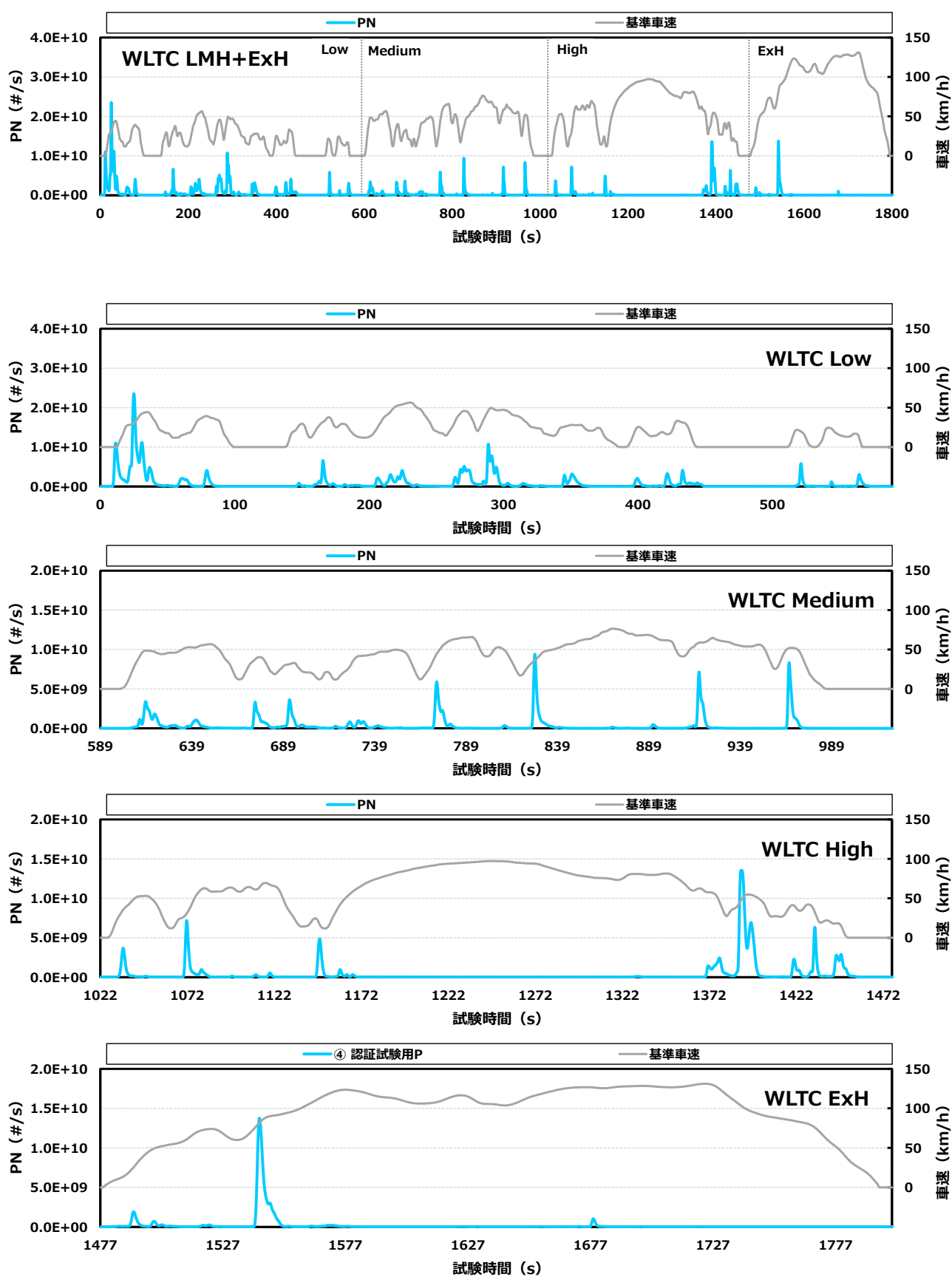
付録図 5.4 ④ 認証試験用 P の PN 排出挙動 (D 車)
