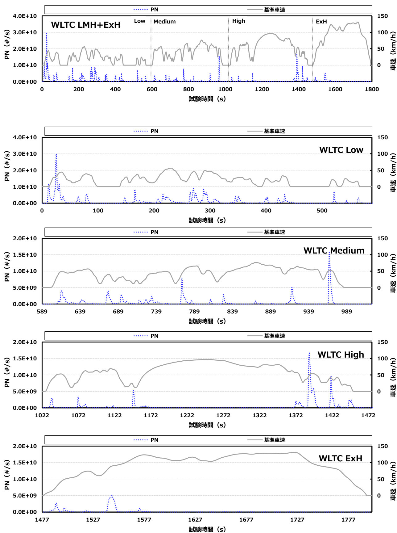
付録図 5.5 ⑤ 認証重質化 P の PN 排出挙動 (D 車)
