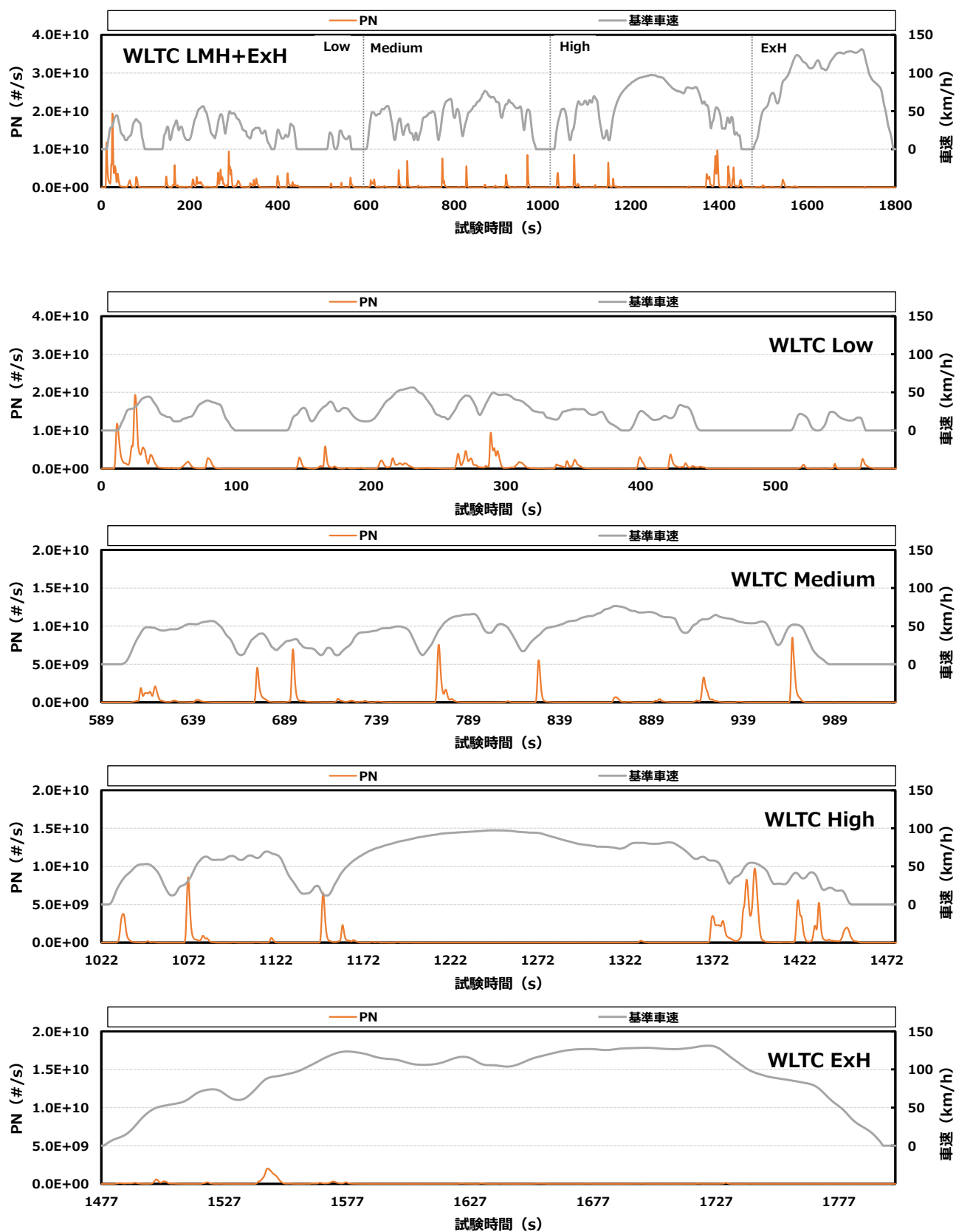
付録図 5.6 ⑥ 市井相当 P の PN 排出挙動 (D 車)
