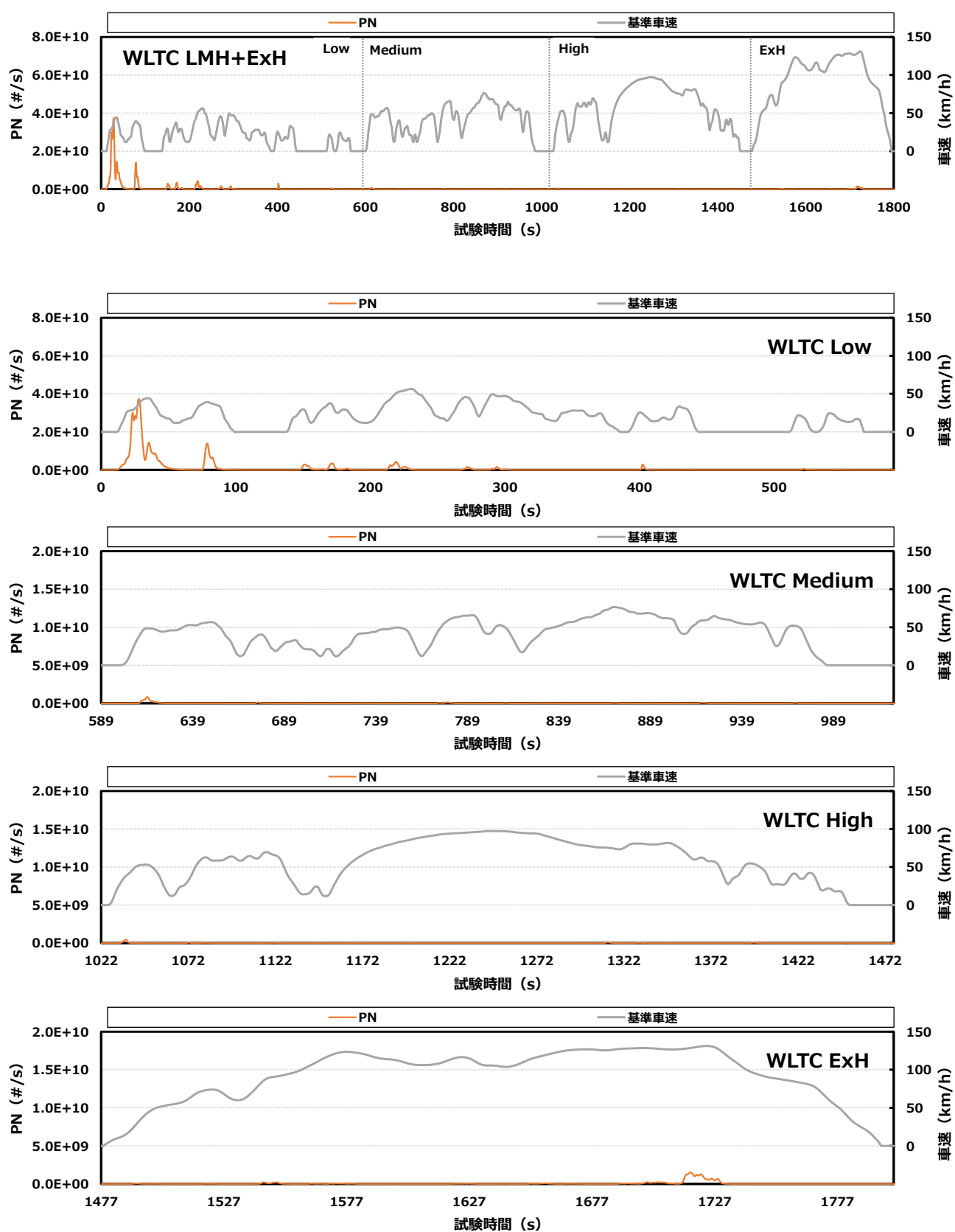
付録図 5.3 ⑥ 市井相当 P の PN 排出挙動 (C 車)
