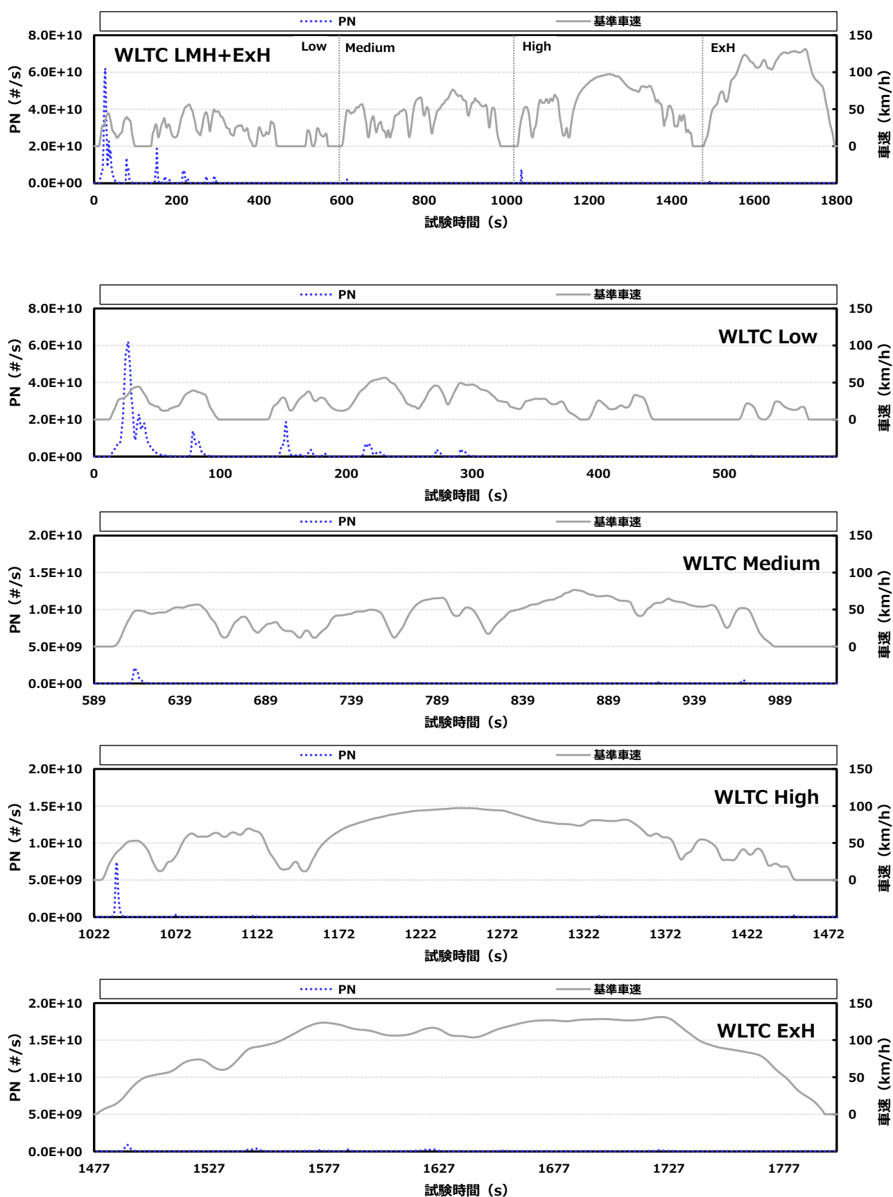
付録図 5.2 ⑤ 認証重質化PのPN排出挙動 (C車)
