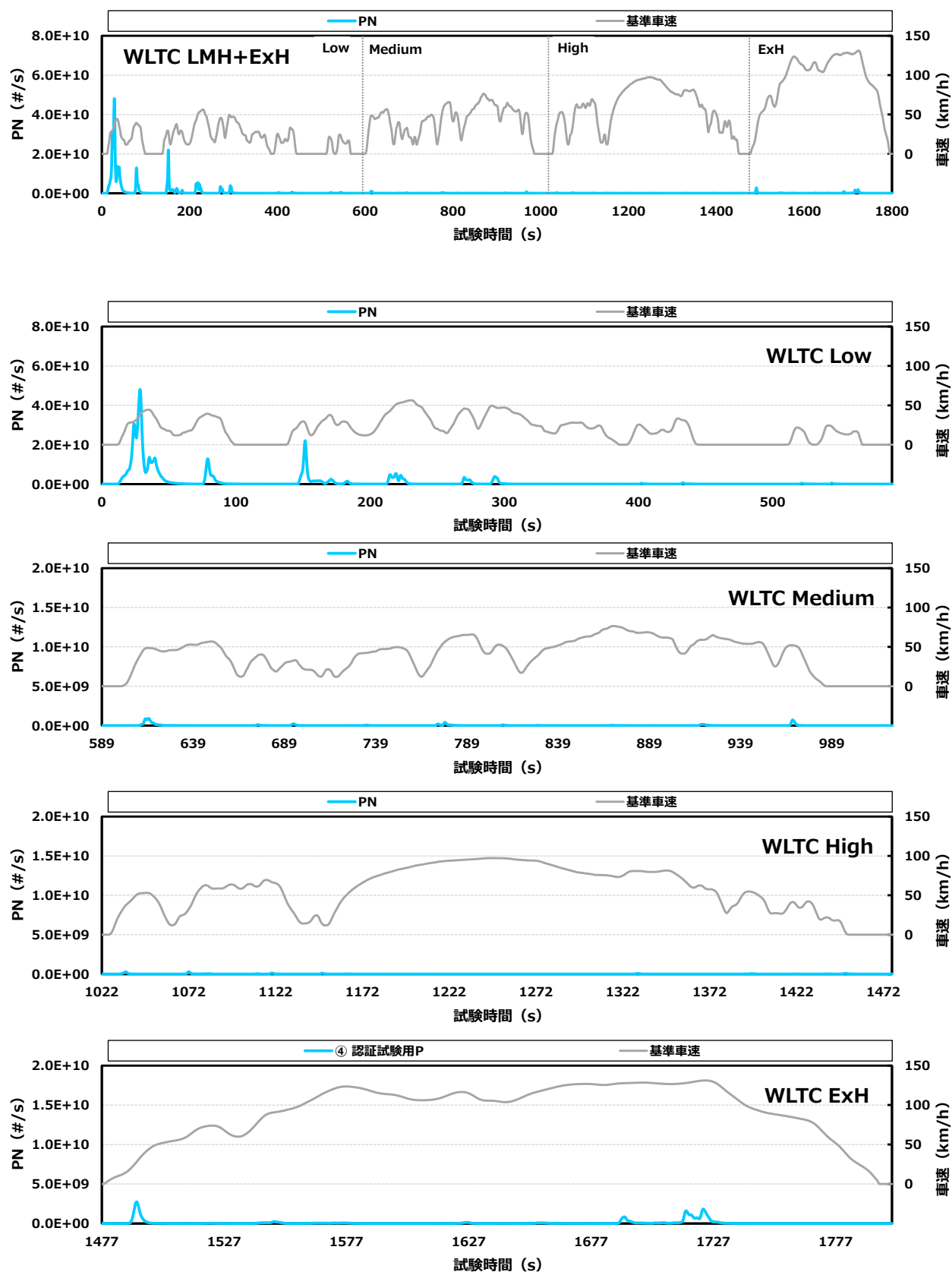
付録図 5.1 ④ 認証試験用PのPN 排出挙動 (C 車)
