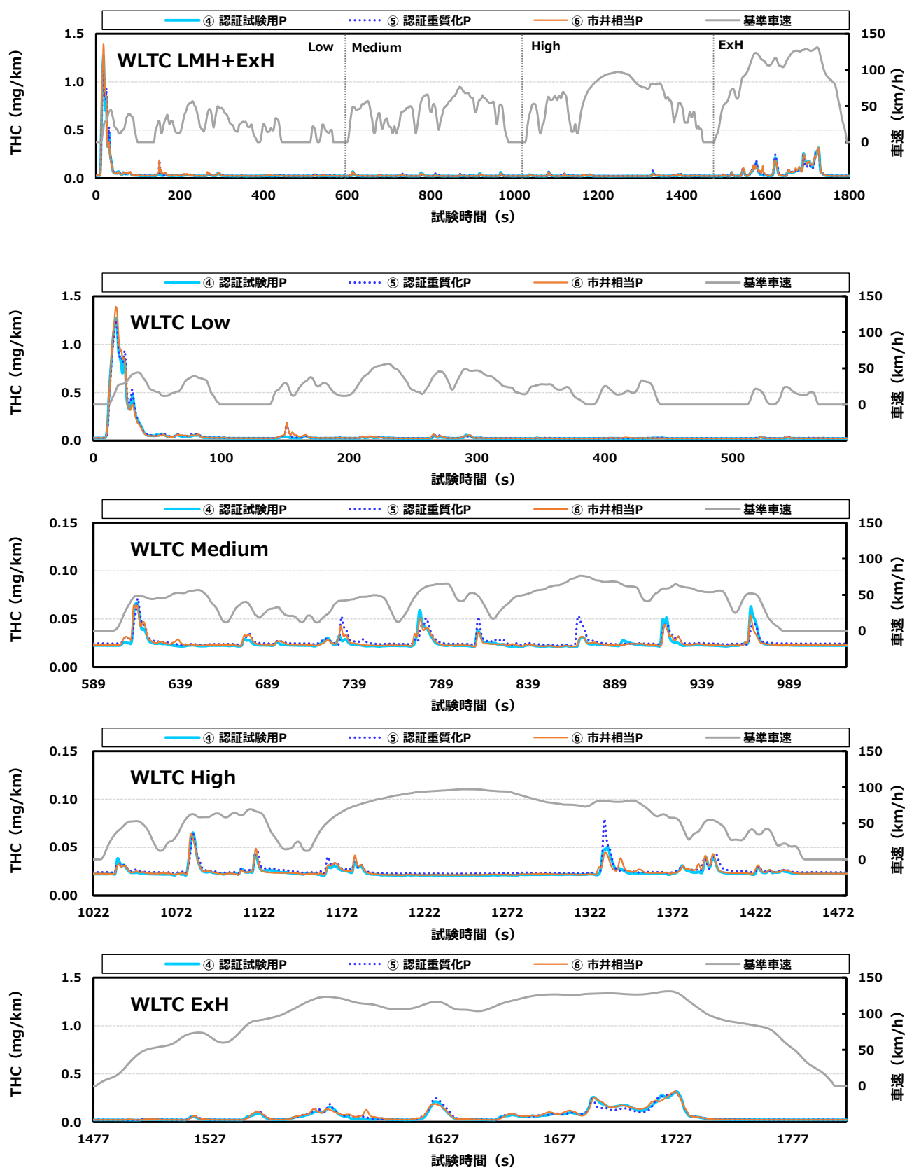
図 3.24 D 車の THC 排出挙動の例
