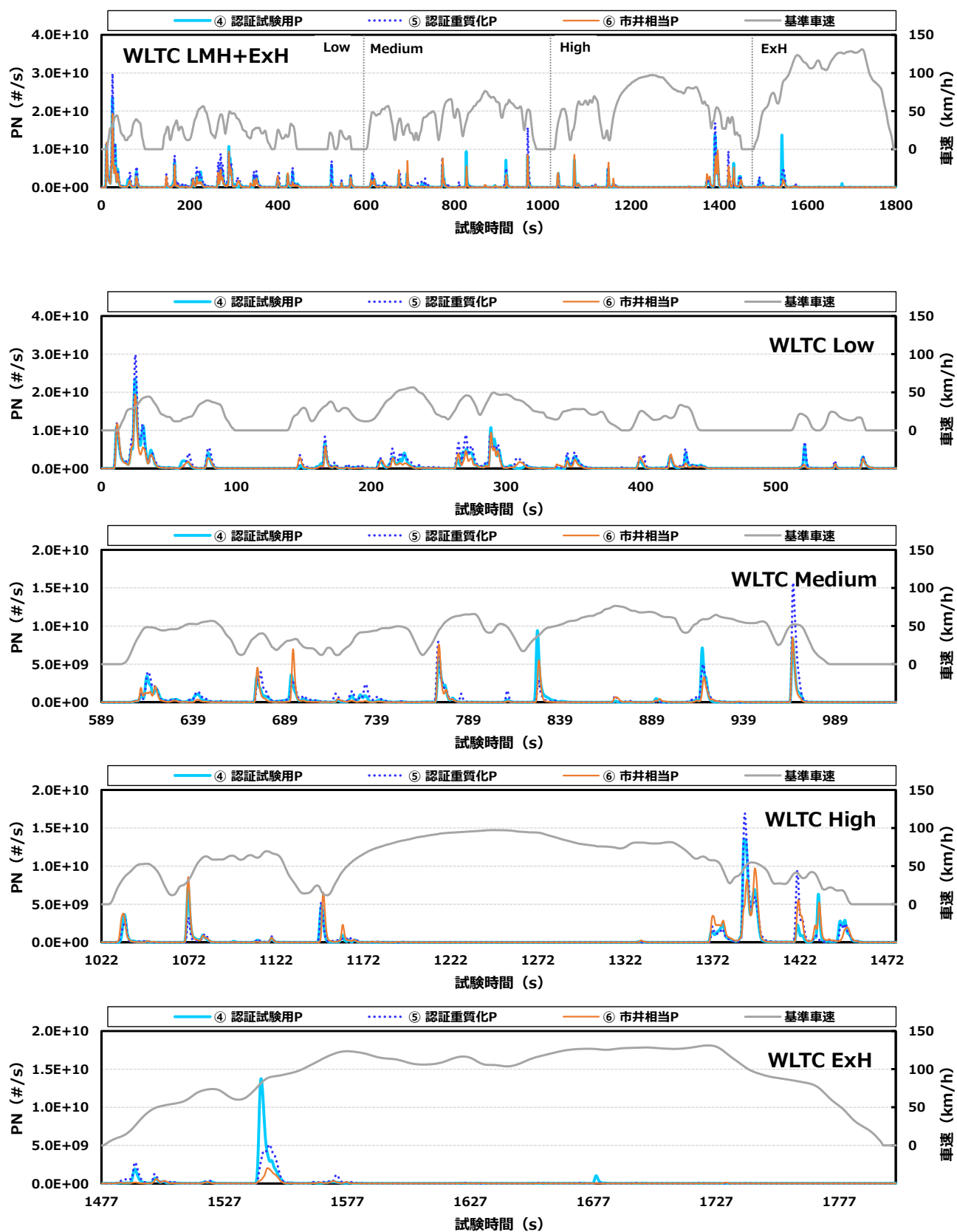
図 3.5 D 車の PN 排出挙動
