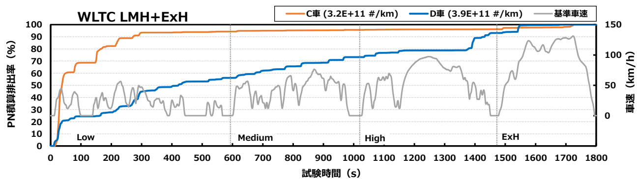
図 3.6 WLTC LMH+ExH における PN 積算排出量の例（燃料は ④認証試験用 P）
