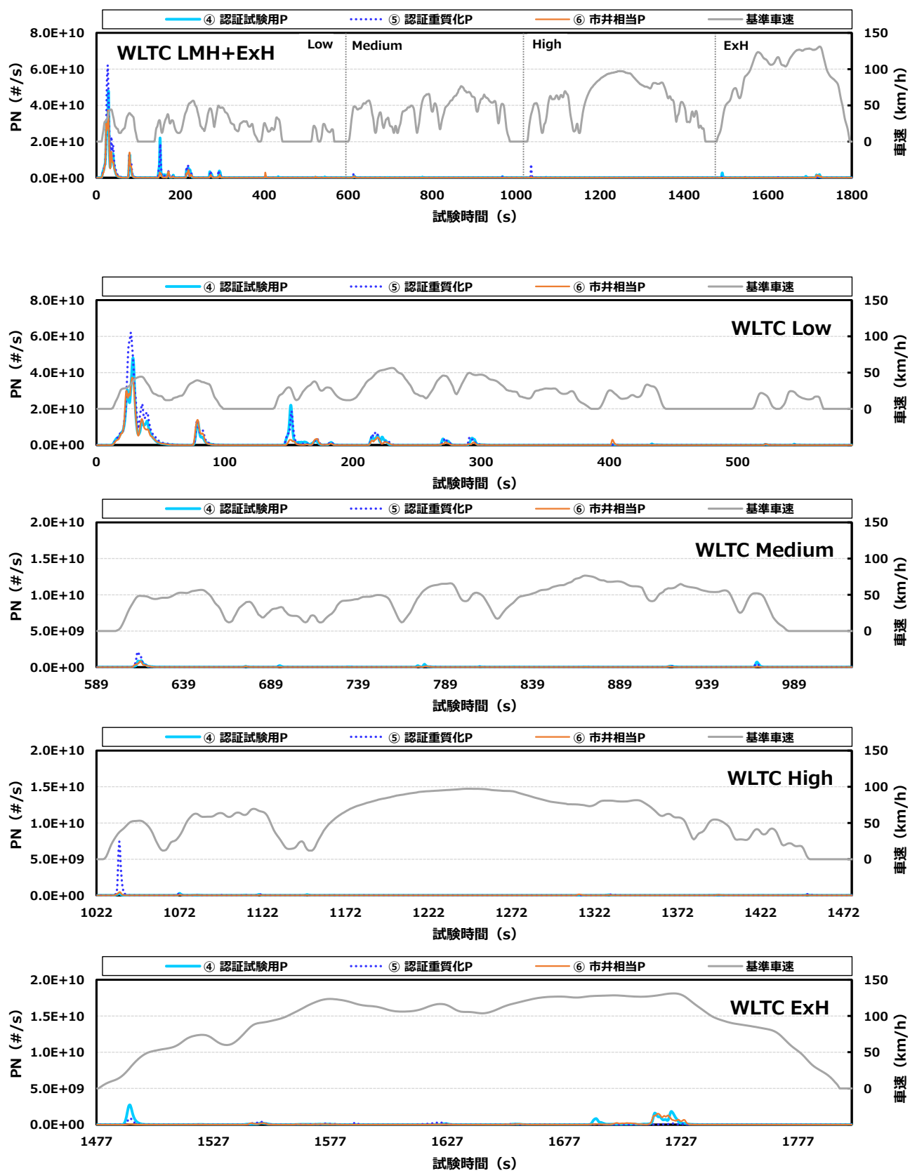
図 3.4 C 車の PN 排出挙動
