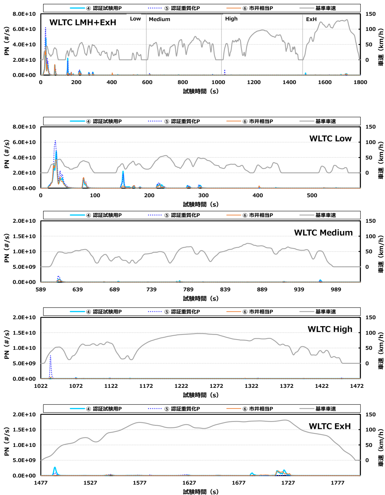
概要図 6 C車のPN排出挙動の例
