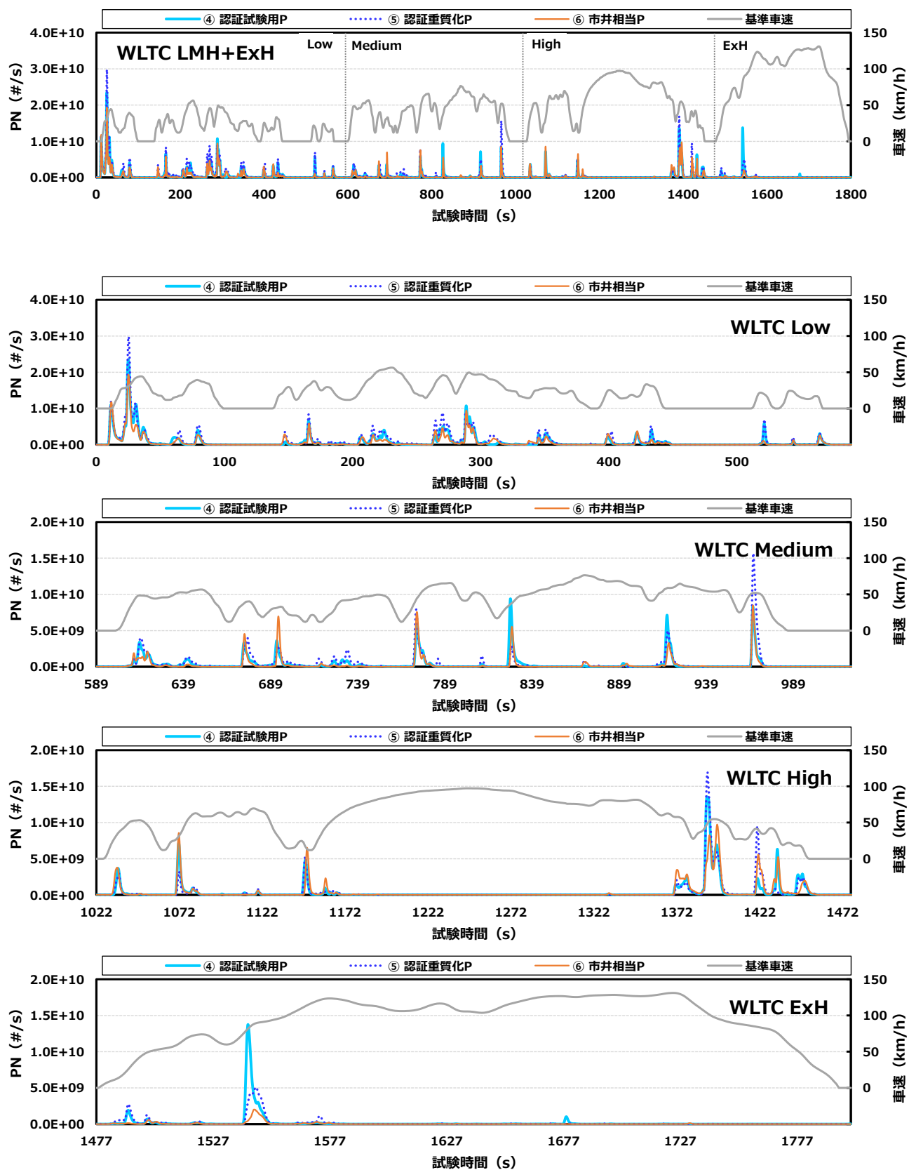
概要図 7 D車のPN排出挙動の例
