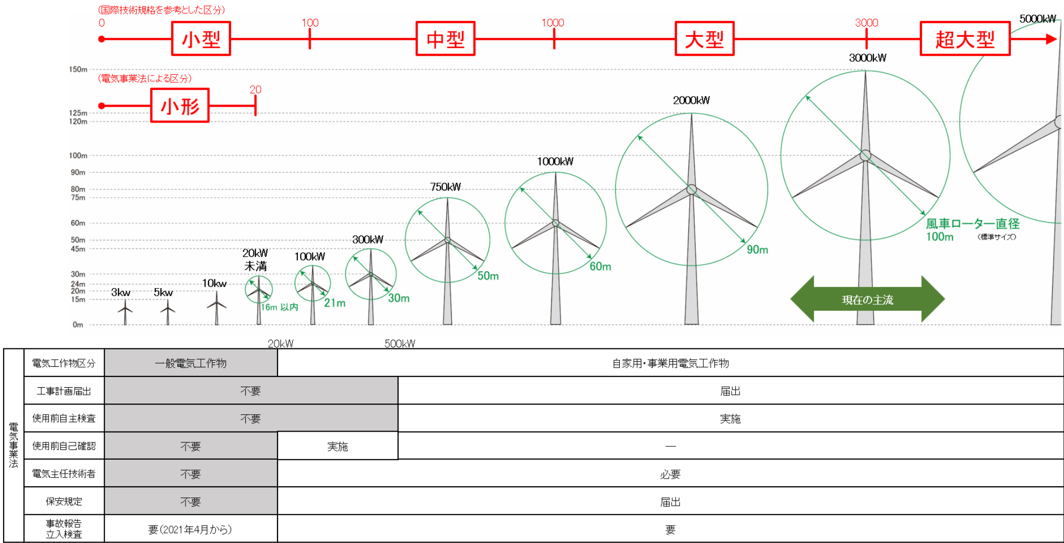
図－82 風力発電施設の規模 29 と電気事業法の規制対象
