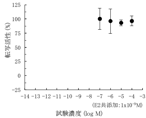
ジブロモクロロメタン
