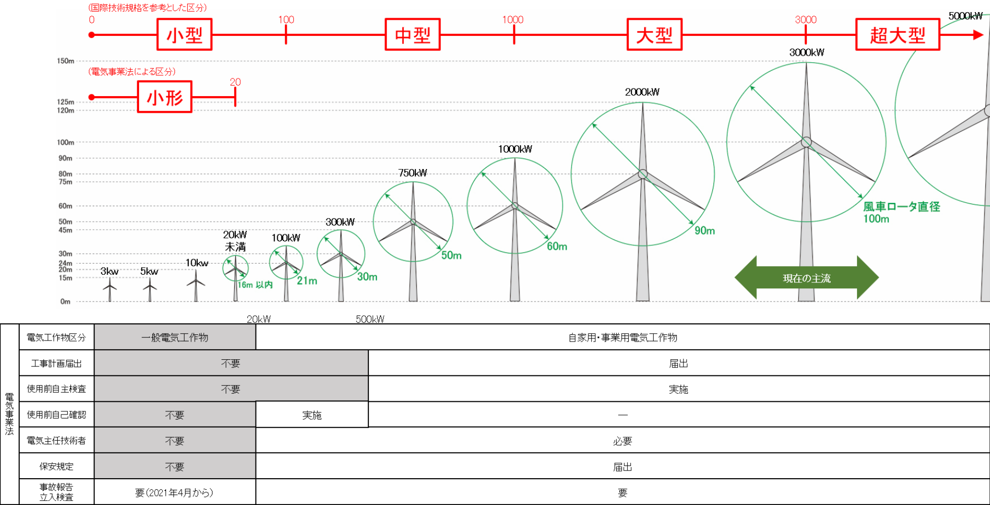
図－72 風力発電施設の規模と電気事業法の規制対象
