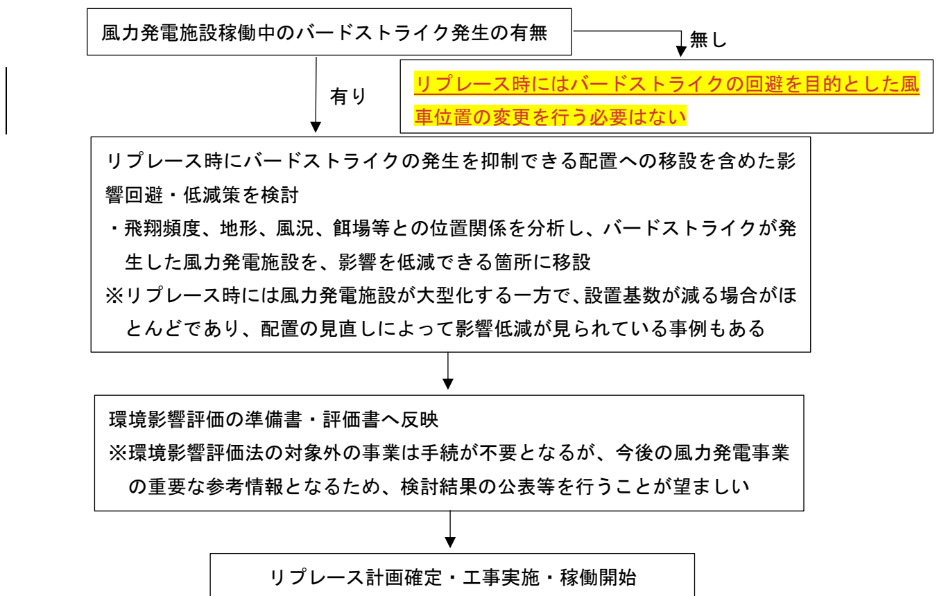
図-52 リプレイス事業におけるバードストライク防止策の検討フロー
