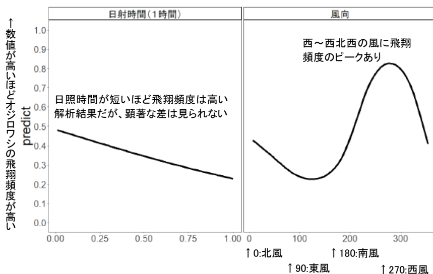
図-49 日照時間、風向とオジロワシの飛翔頻度解析した例
