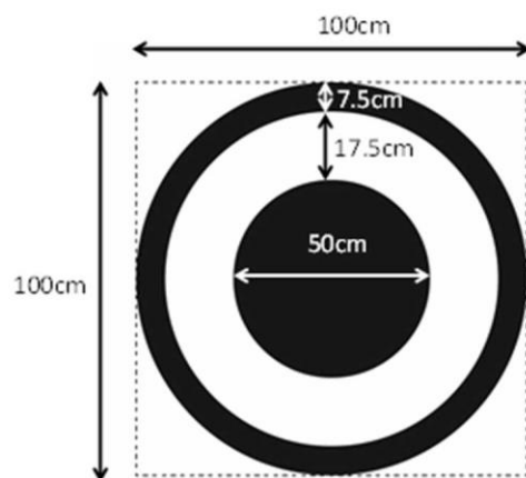
図一65 目玉模様彩色の例
