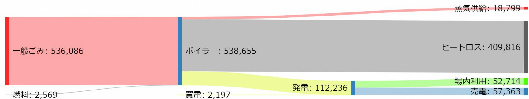
図 2-7 本施設のエネルギー収支 (2020 年度, 単位 : GJ/年)
