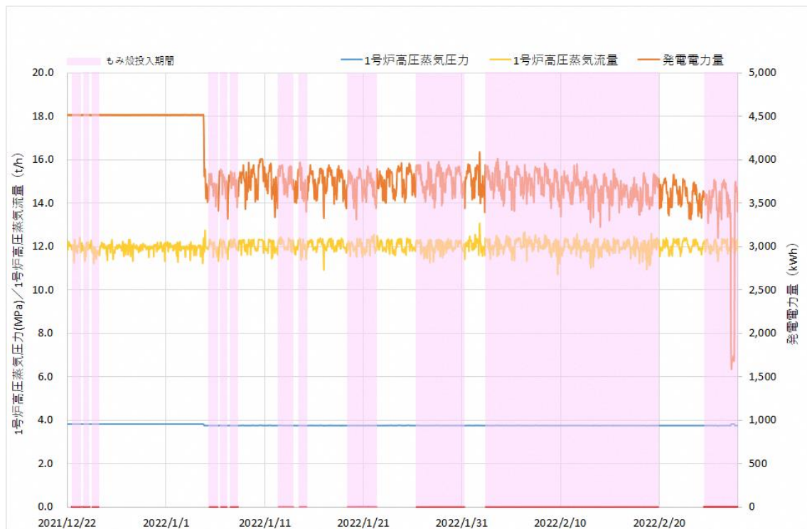
図 3-11 混焼前後運転データ（1号炉高压蒸汽压力/流量/発電電力量）
