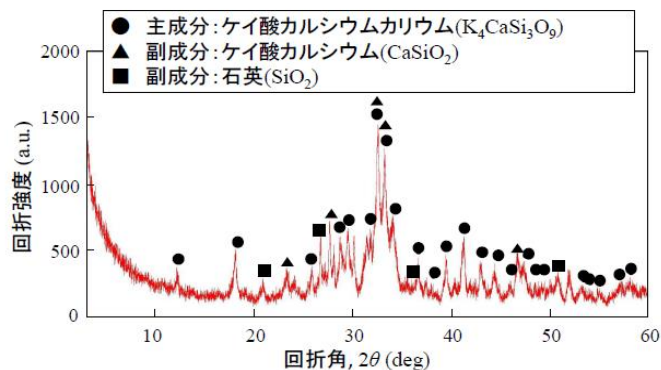
図 2-22 杉樹皮にクリンカ生成防止剤を配合したペレット燃焼灰組成と X 線回折スペクトル
