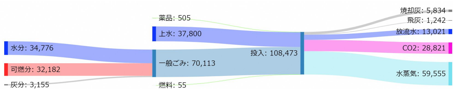
図 2-6 本施設の物質収支 (2020 年度, 単位 : t/年)
