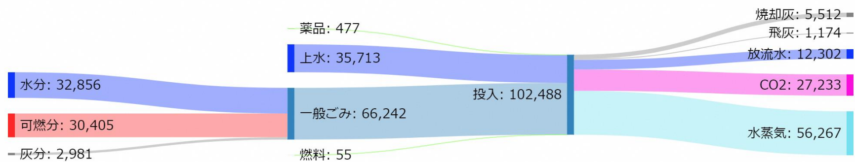
図 2-10 本施設の物質収支 (2024 年度予測, 単位 : t/年)
