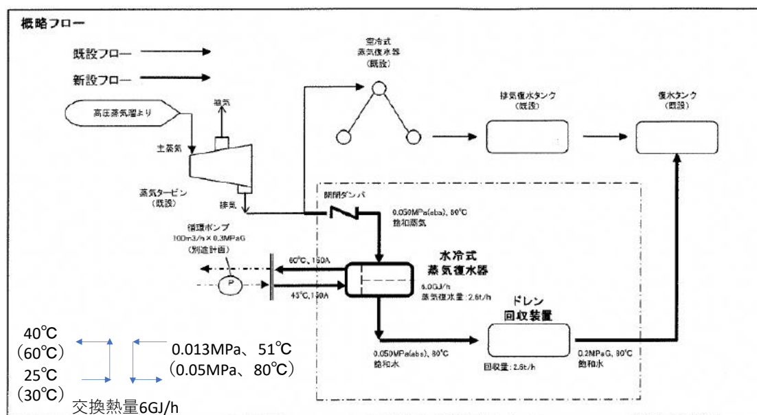
図 4-9 水冷式復水器導入時の概略フロー
