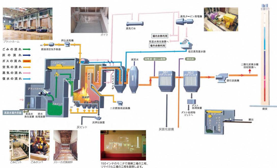
図 2-2 本施設の概要図 [2-2]
