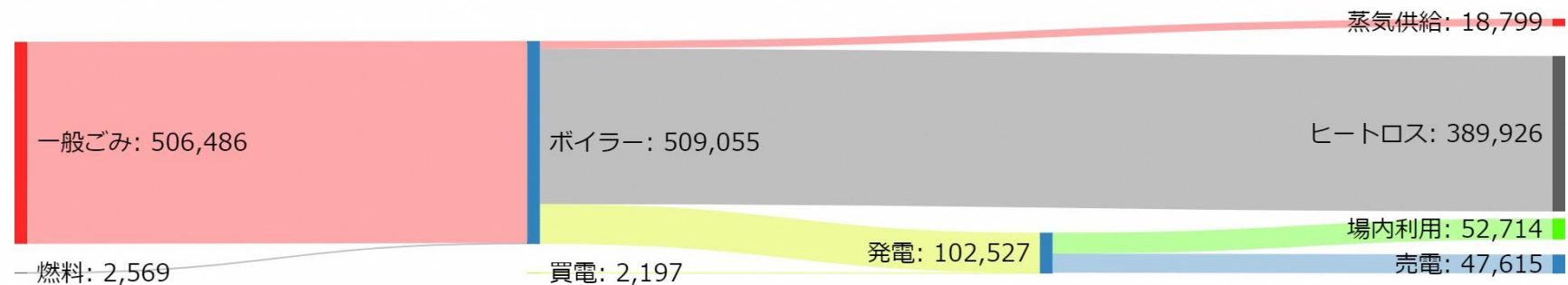
図 2-11 本施設のエネルギー収支 (2024 年度予測, 単位 : GJ/年)
