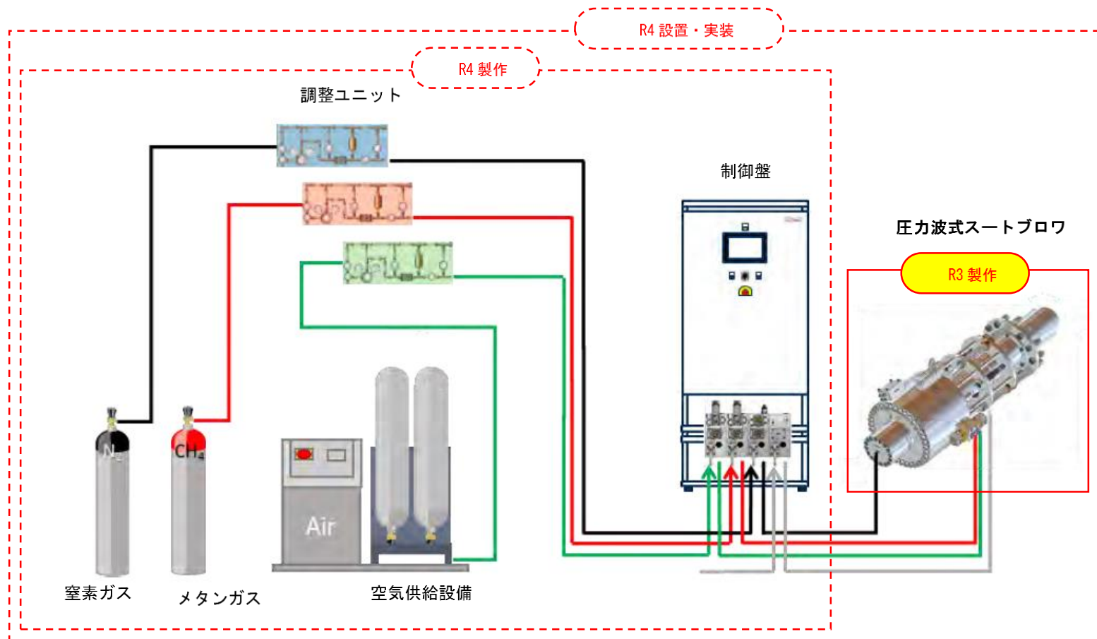
図 3-24 圧力波式ストロブ本体および付帯設備フロー図
