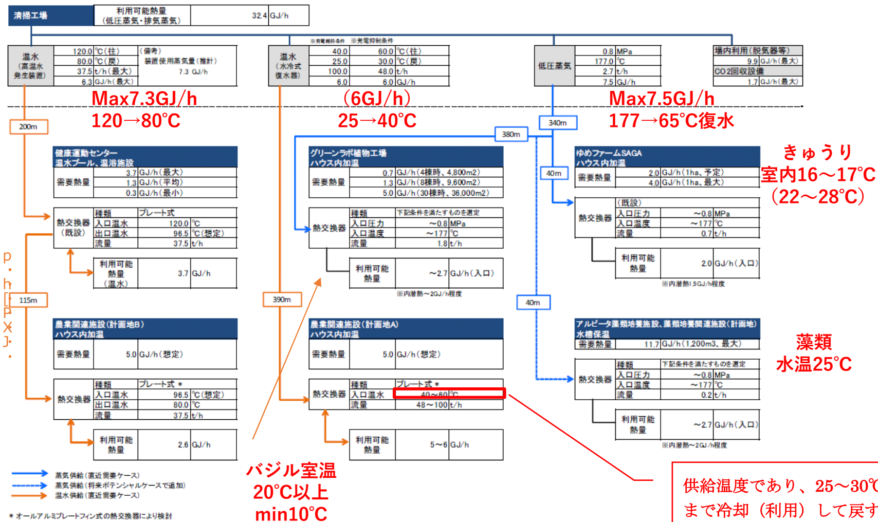
図 4-6 熱供給フロー
