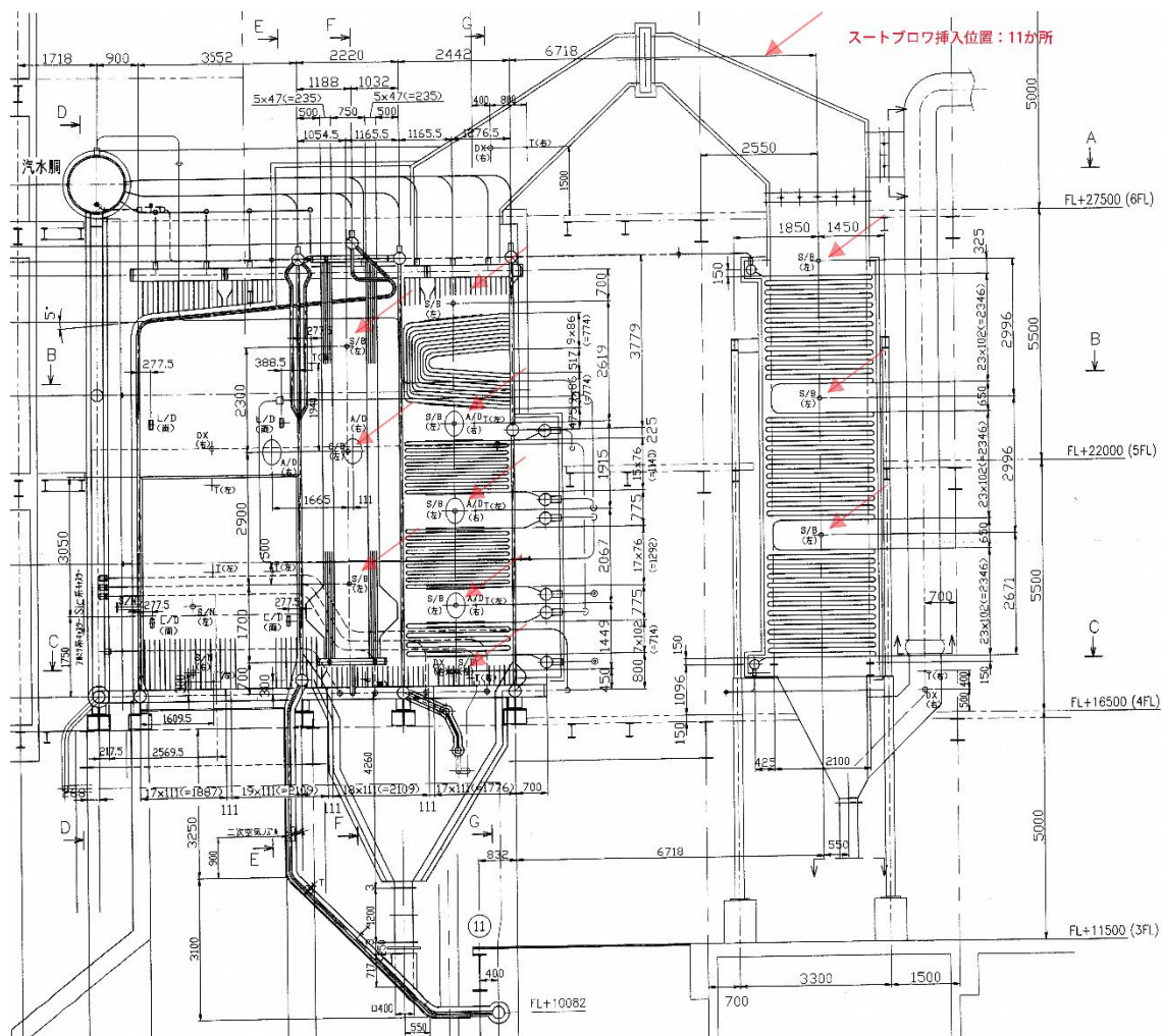
図 3-17 ボイラ構造図 (スートブロウ設置個所)
