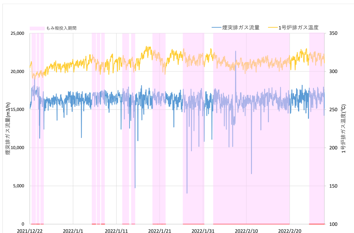
図 3-10 混焼前後運転データ（煙突排ガス流量/1号炉排ガス温度）
