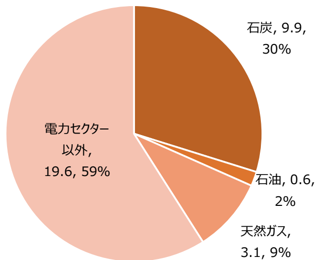
グローバルのCO2排出量（単位：Gt）
