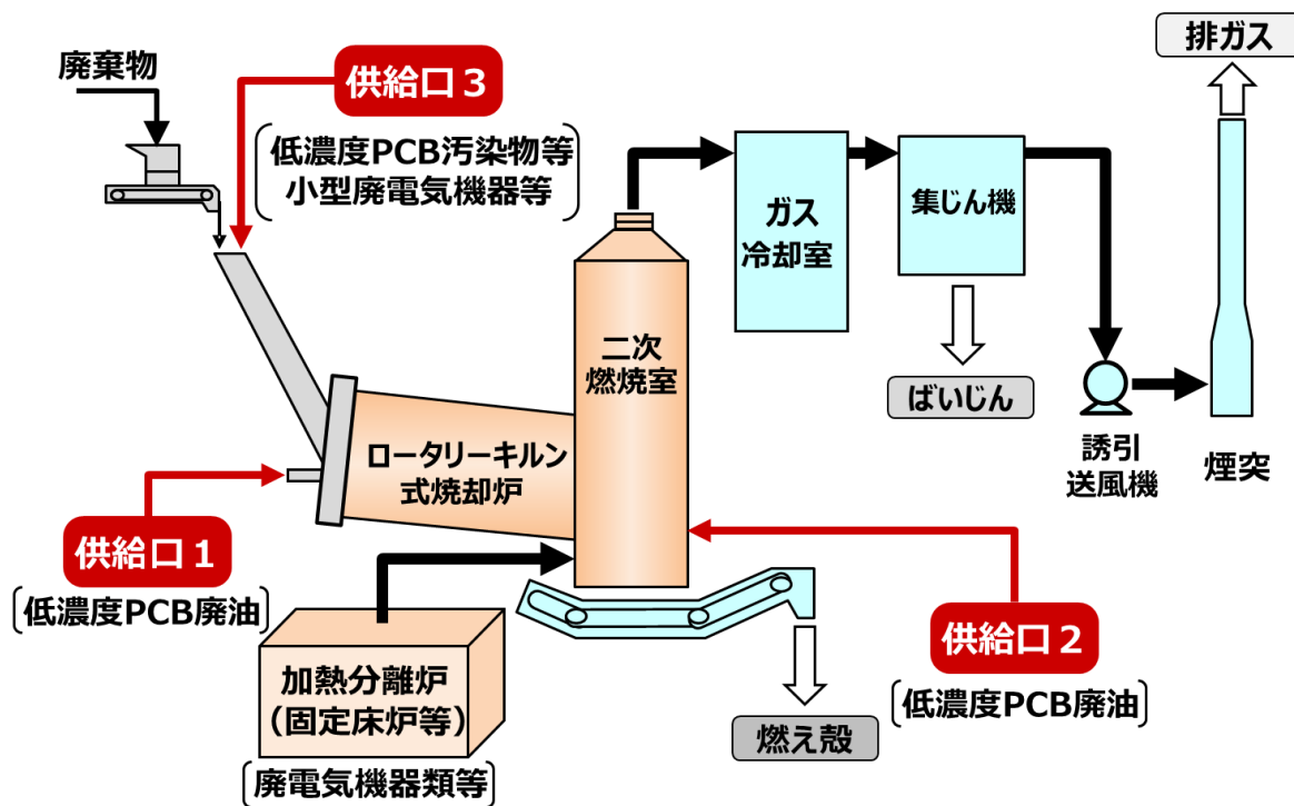
廃棄物焼却炉による PCB 汚染物等の焼却処理（例）
