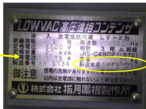
銘板 (昭和 48 年(1973 年) 6 月製造)
