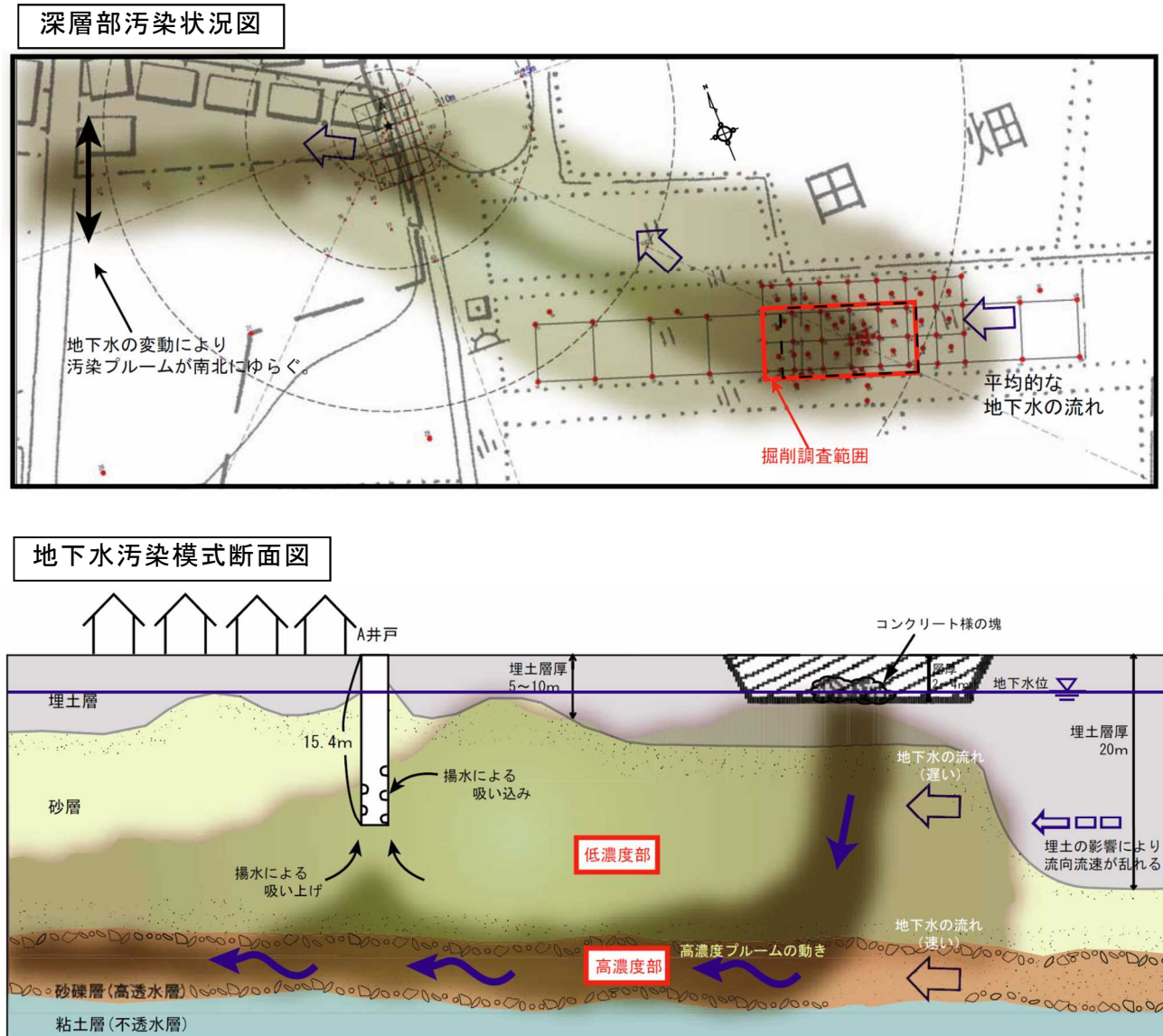
図 2-1 A 井戸周辺の汚染メカニズム
