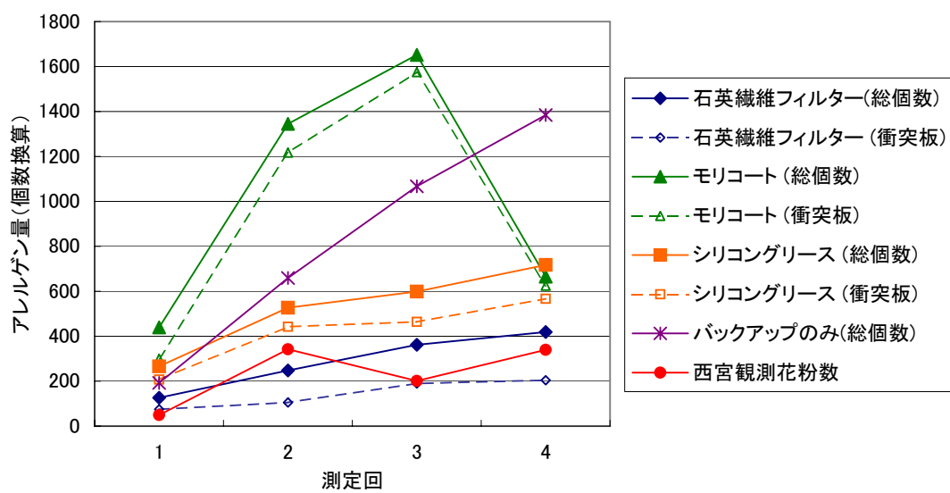
図1 衝突板の捕集効率に関する予備実験結果
