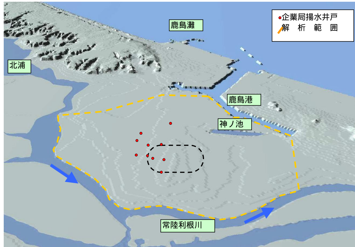
図 6.2.1 広域地下水シミュレーション範囲（標高 5 倍表示）
