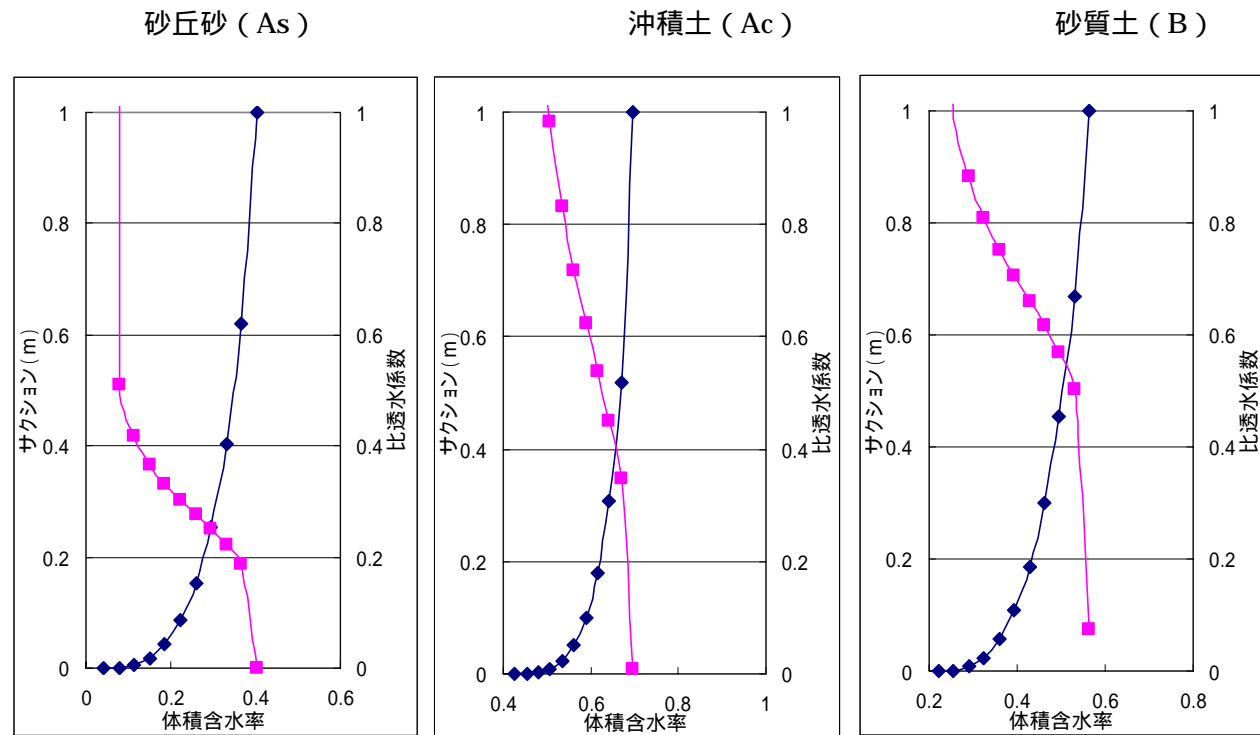
図 6.2.2 不飽和特性曲線
