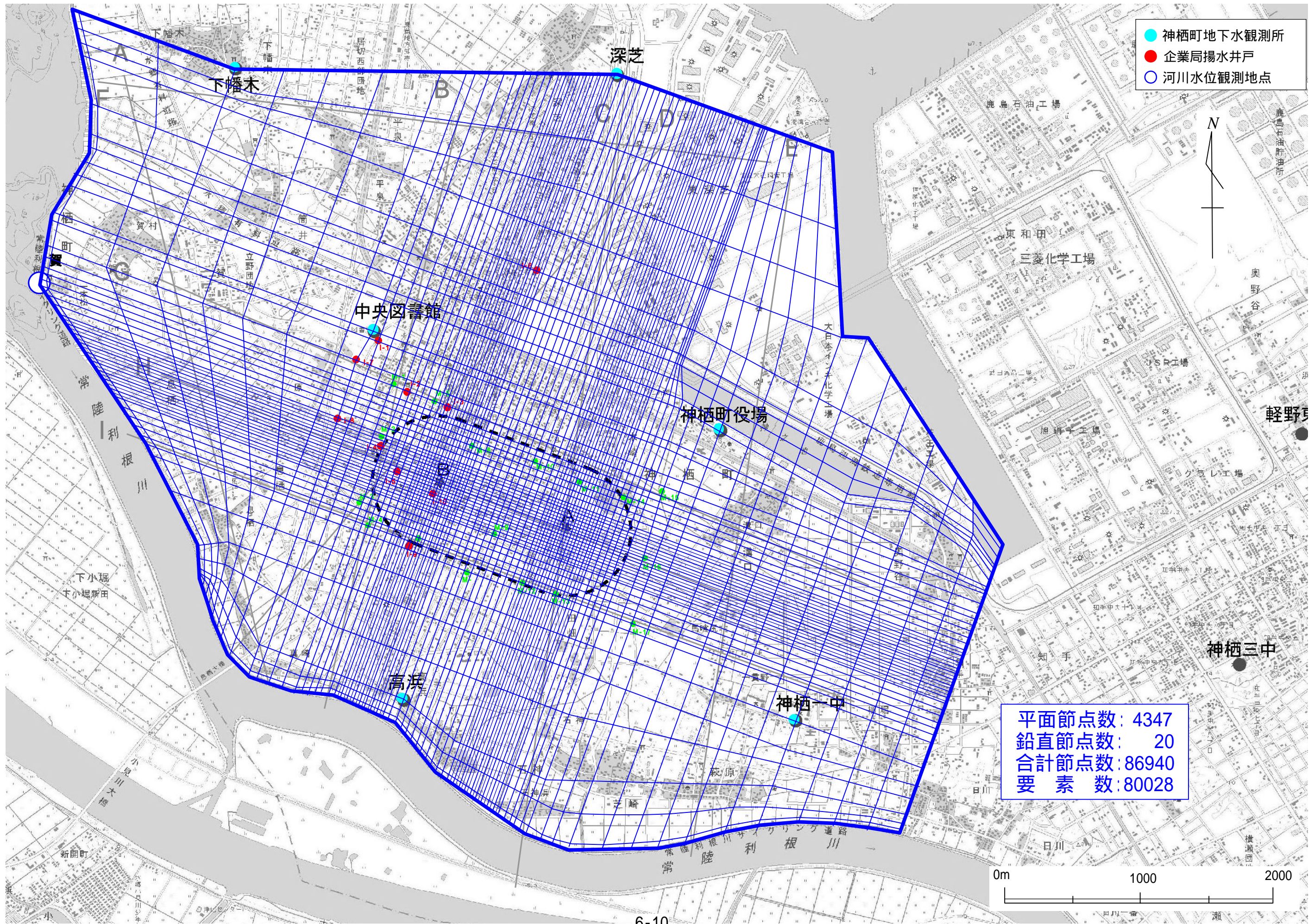
図6.2.2 三次元解析メッシュ分割図
