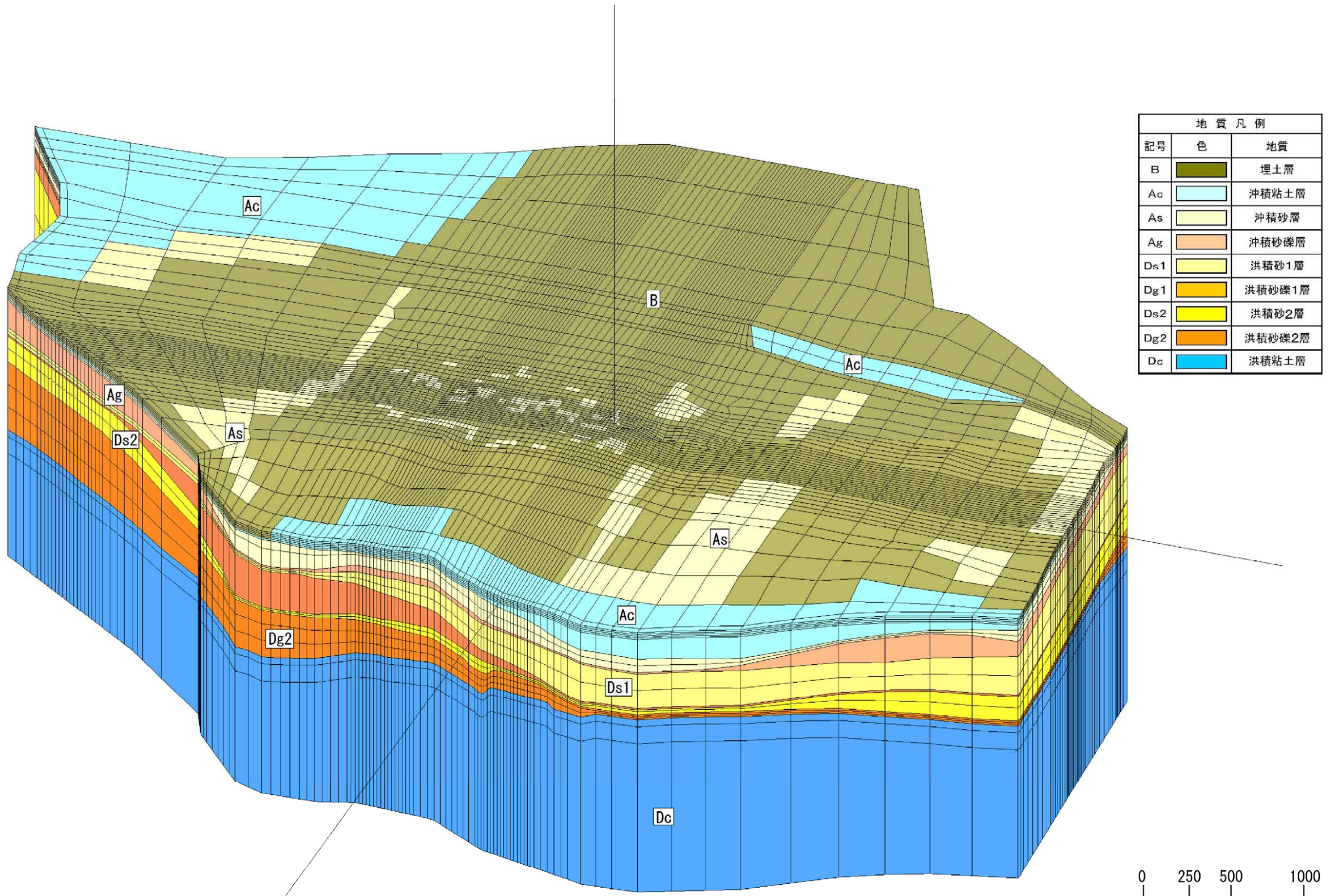
図6.2.3 三次元地盤モデル
