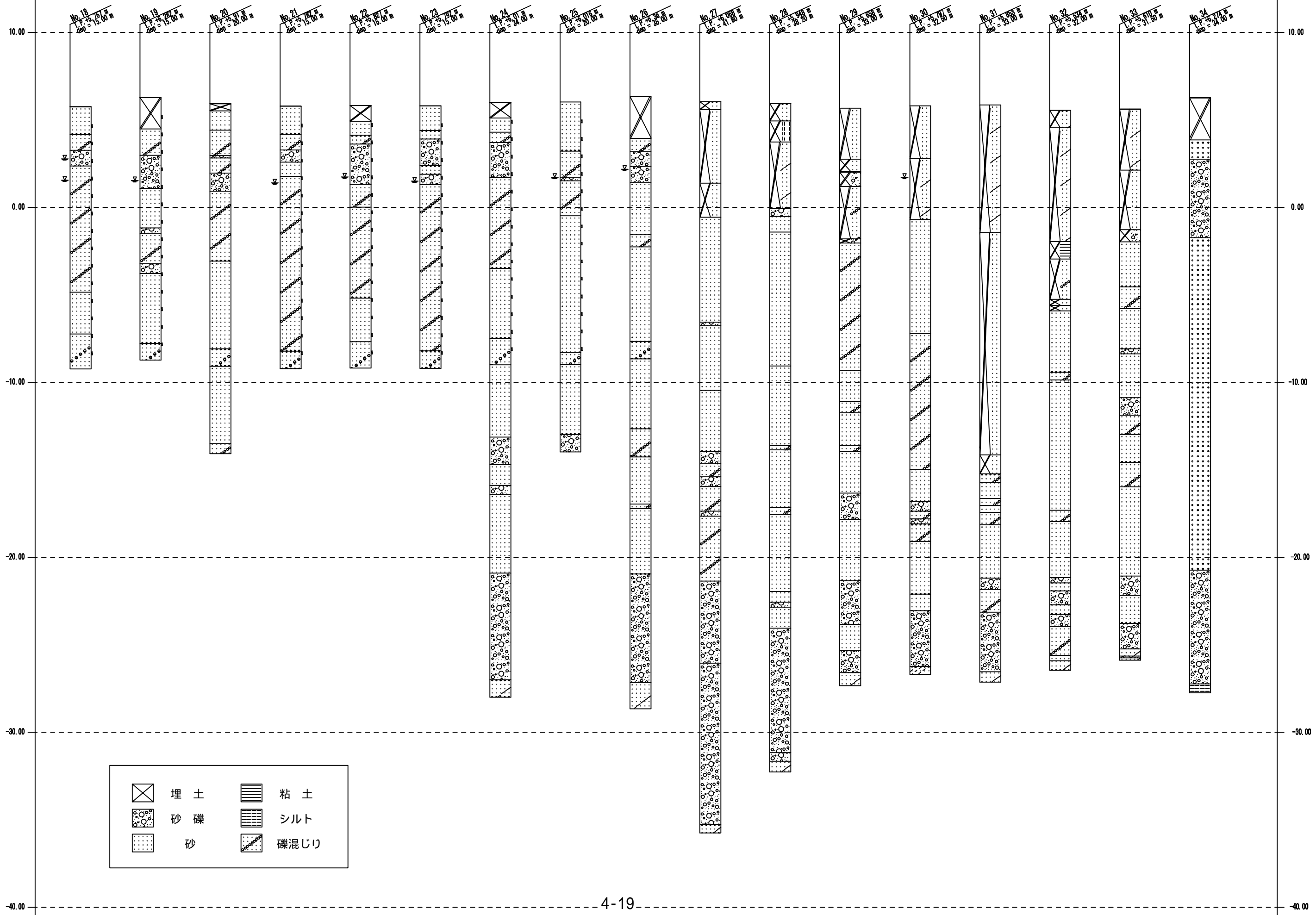
図4.2.6 環境ボーリング柱状図(2)
