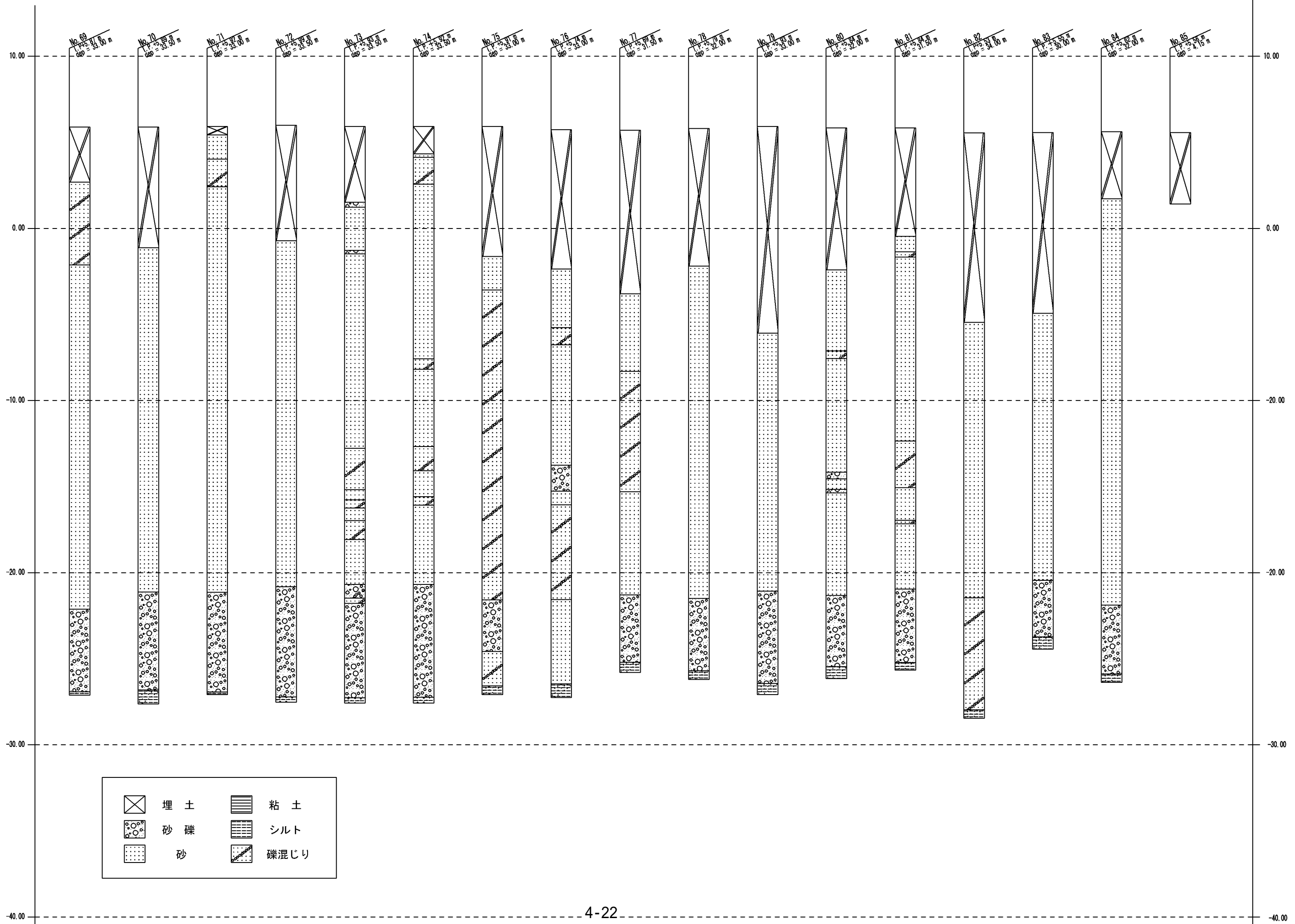
図4.2.6 環境ボーリング柱状図(5)
