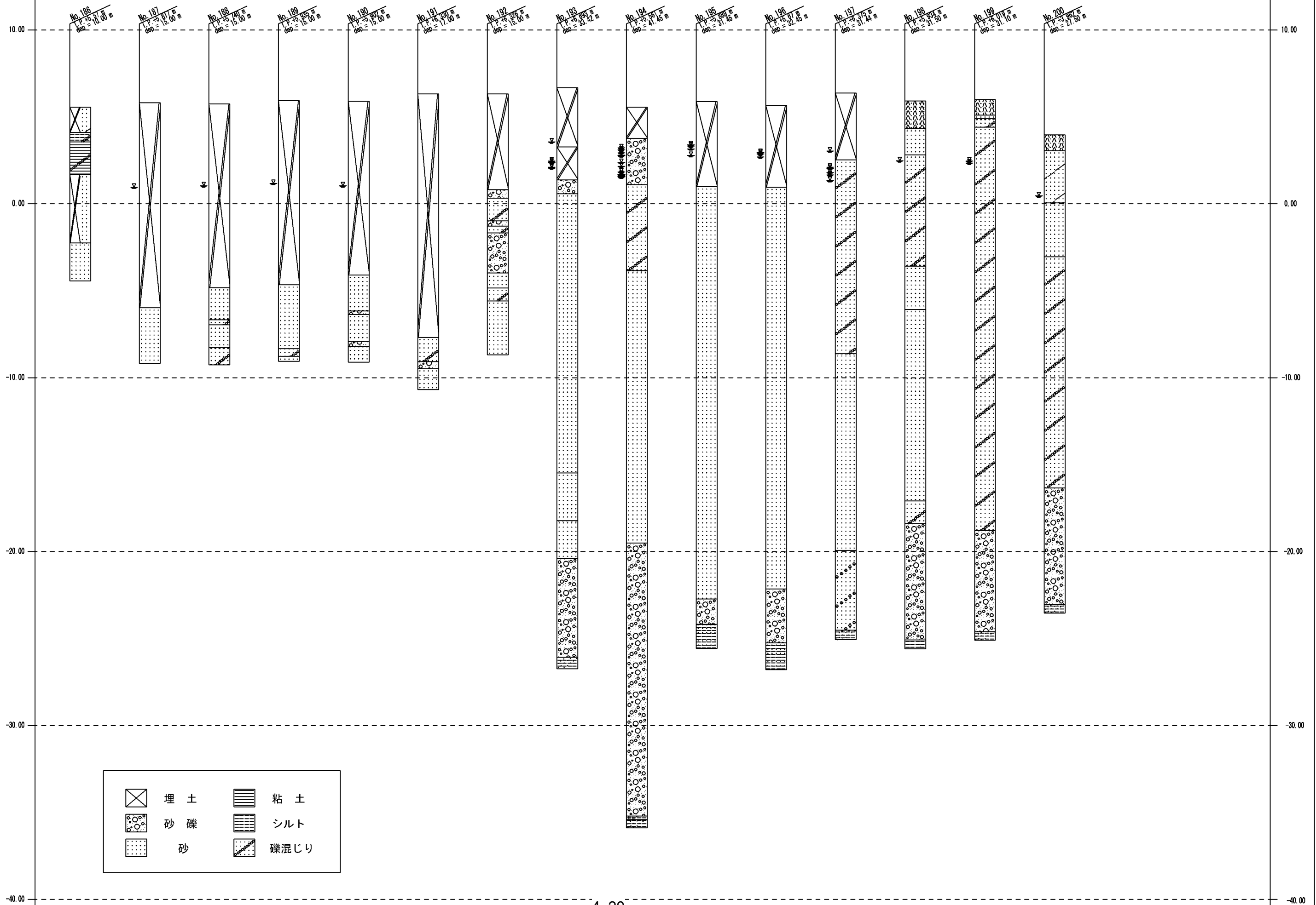
図4.2.6 環境ボーリング柱状図(12)
