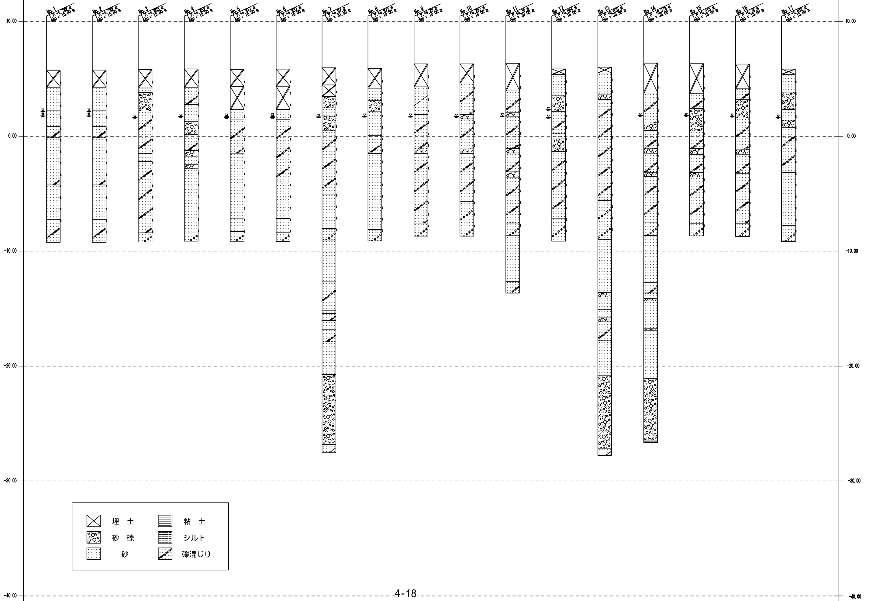
図4.2.6 環境ボーリング柱状図(1)
