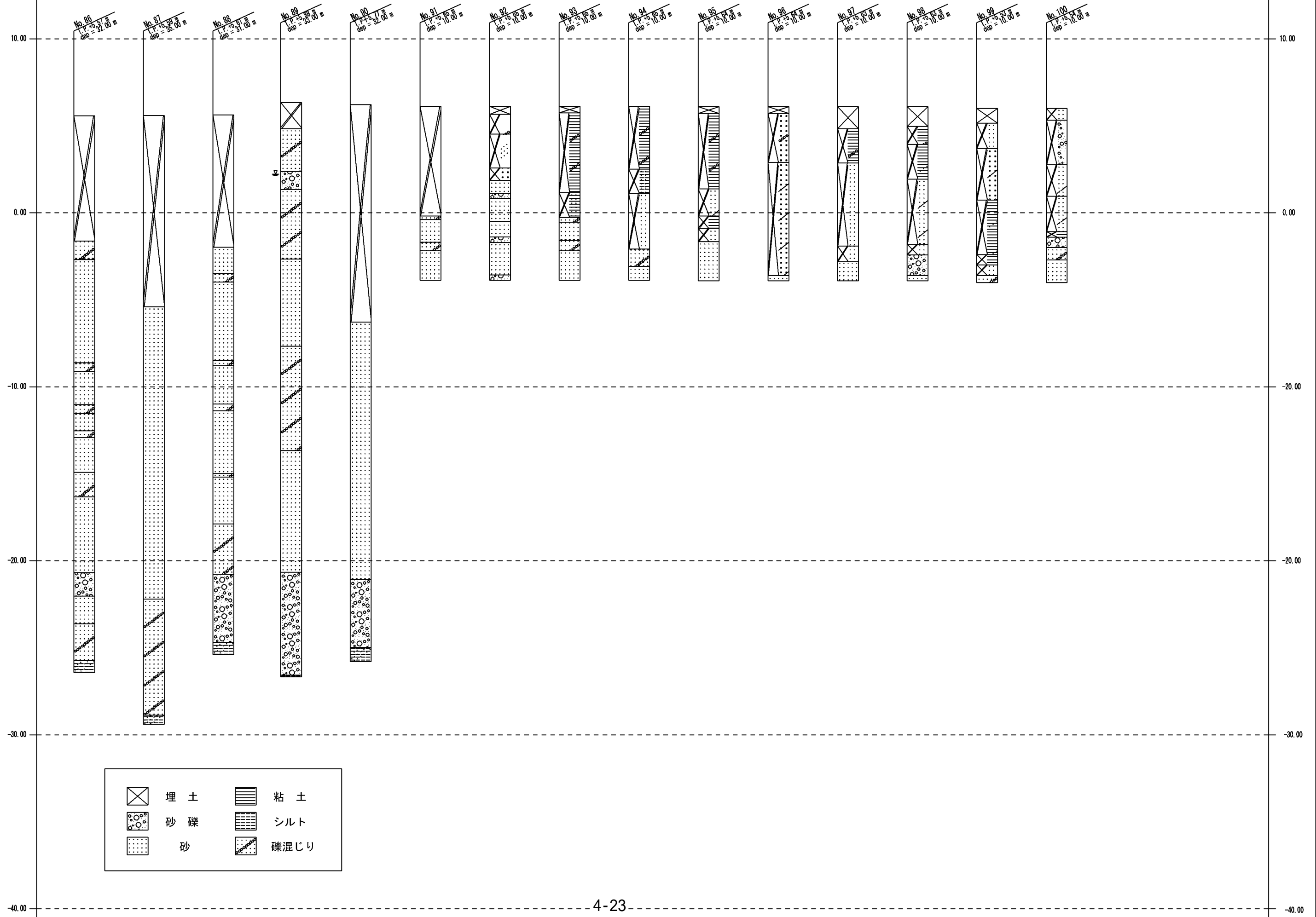
図4.2.6 環境ボーリング柱状図(6)
