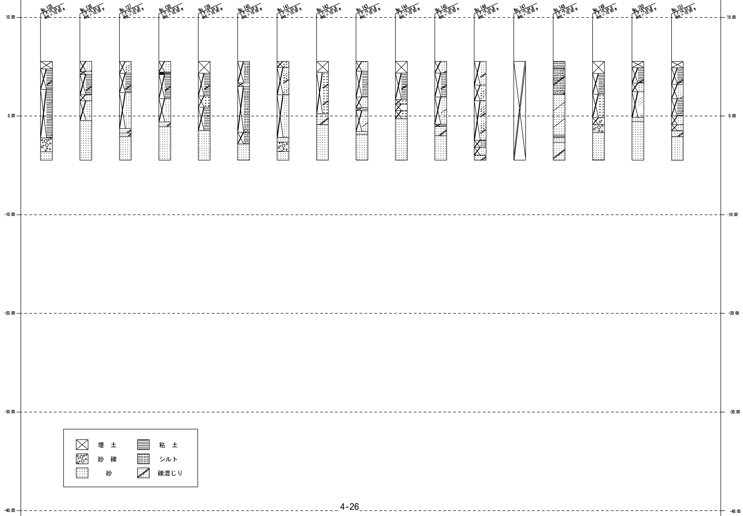
図4.2.6 環境ボーリング柱状図(9)
