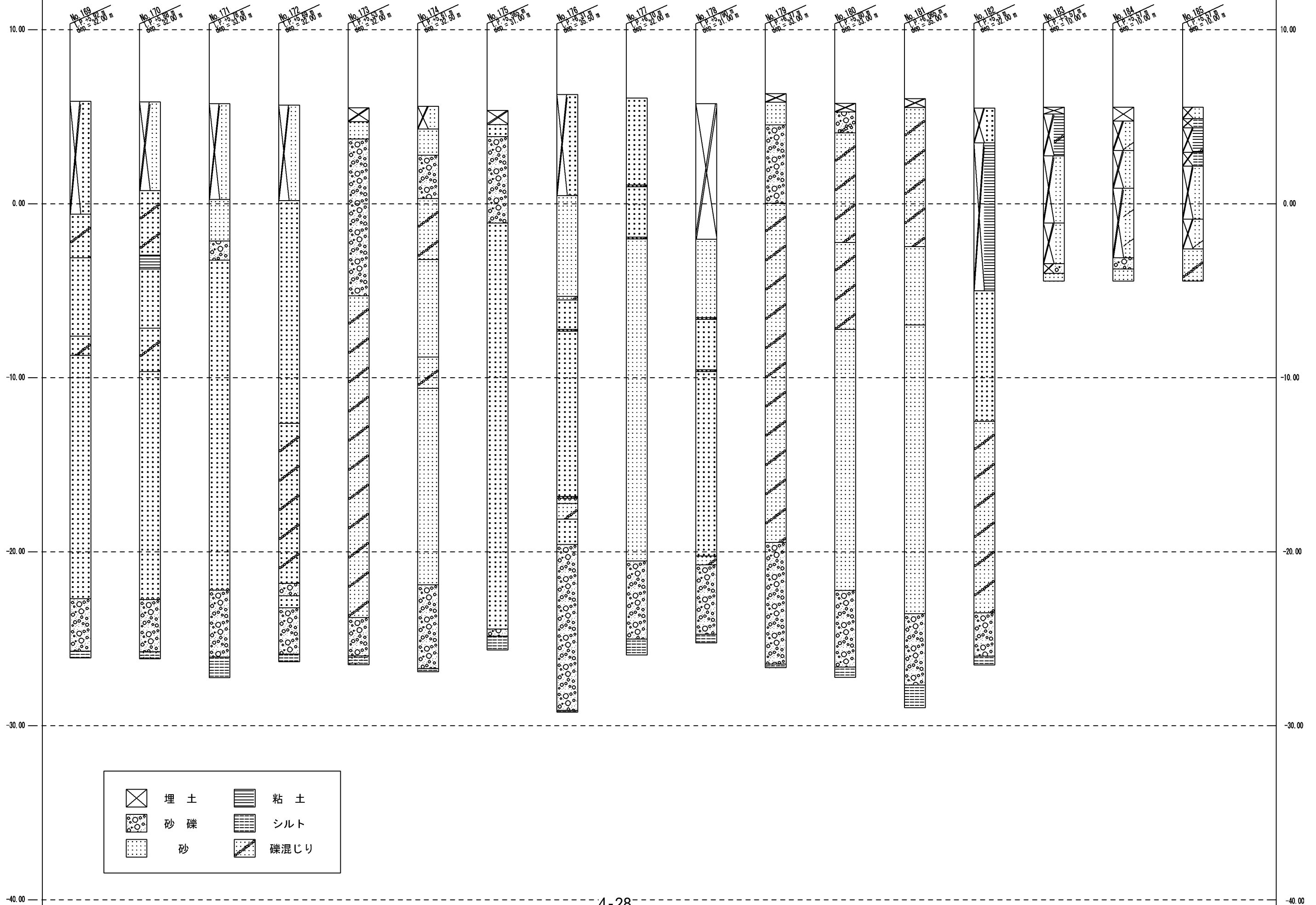
図4.2.6 環境ボーリング柱状図 (11)
