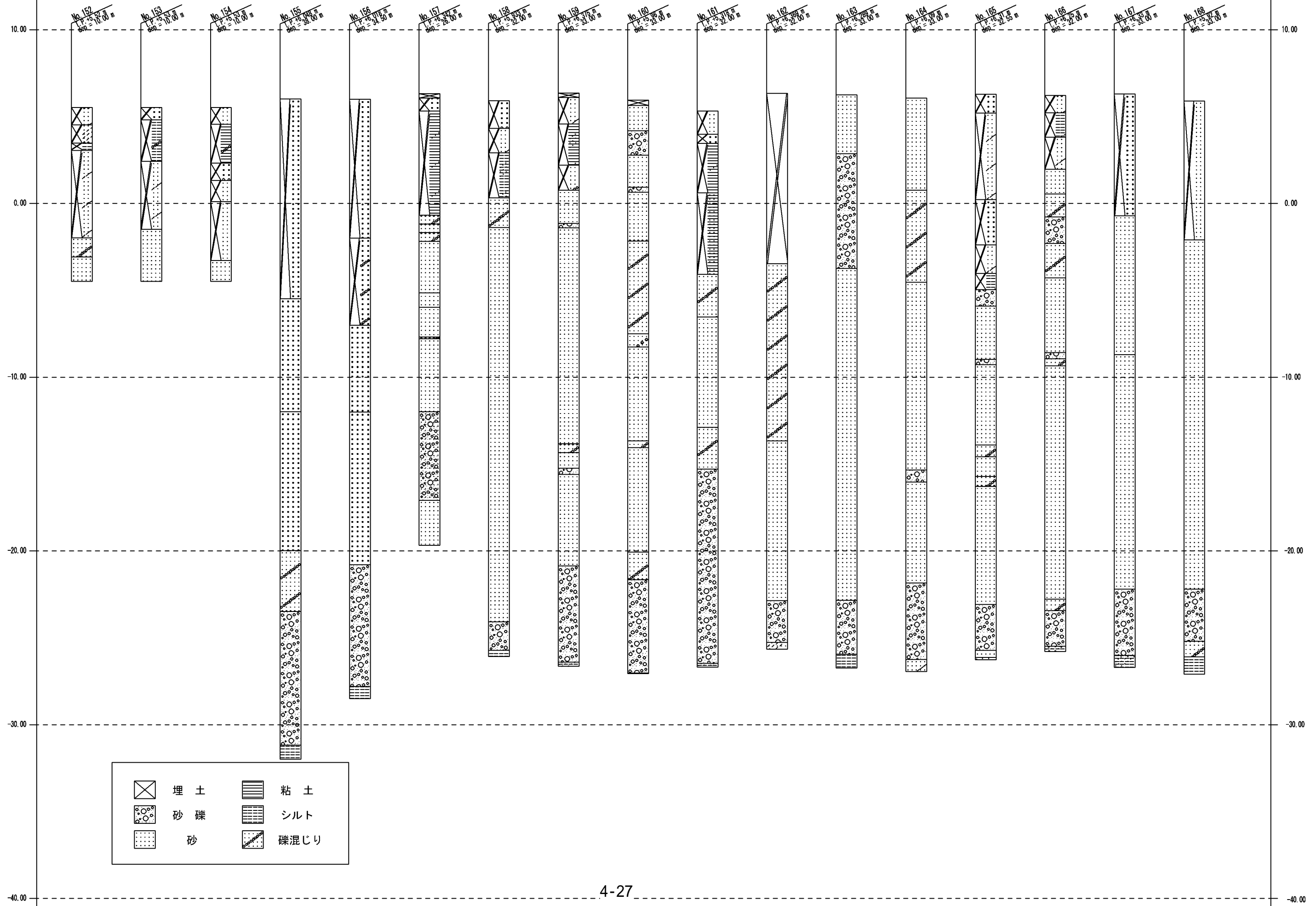
図4.2.6 環境ボーリング柱状図(10)
