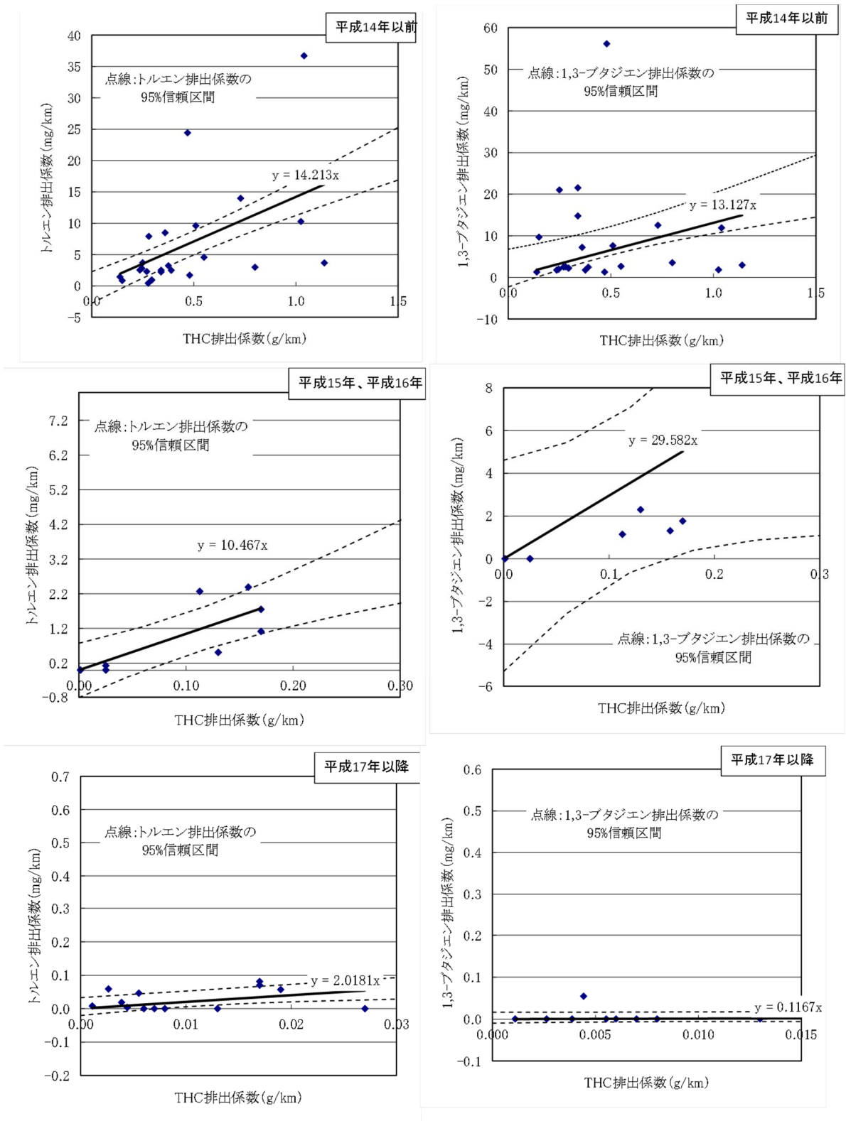
図11-40 ディーゼル自動車(ホットスタート:重量車)に係る THC 排出量と対象化学物質別排出量の比率(その 4)
