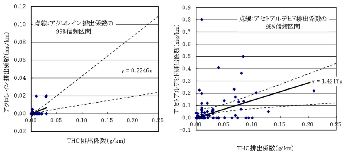
図11-37 ガソリン自動車(ホットスタート)に係る THC 排出量と対象化学物質別排出量の比率(その1)
