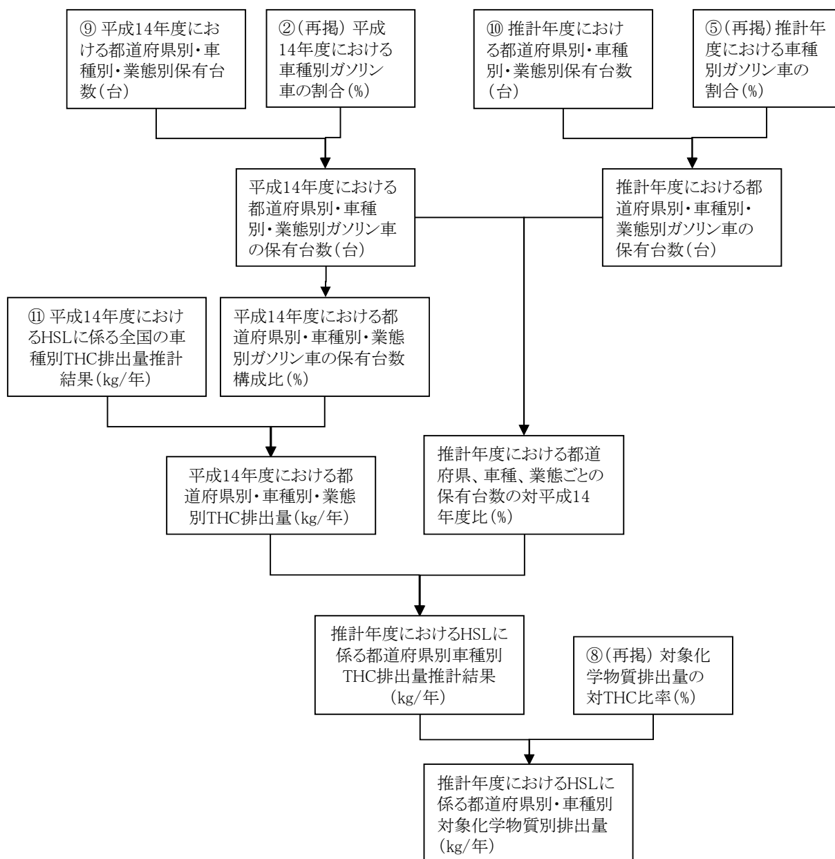
図11-34 燃料蒸発ガス(HSL)に係る対象化学物質別排出量推計フロー
