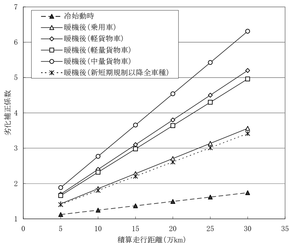
図11-22 経過年数(積算走行距離)による劣化補正係数
