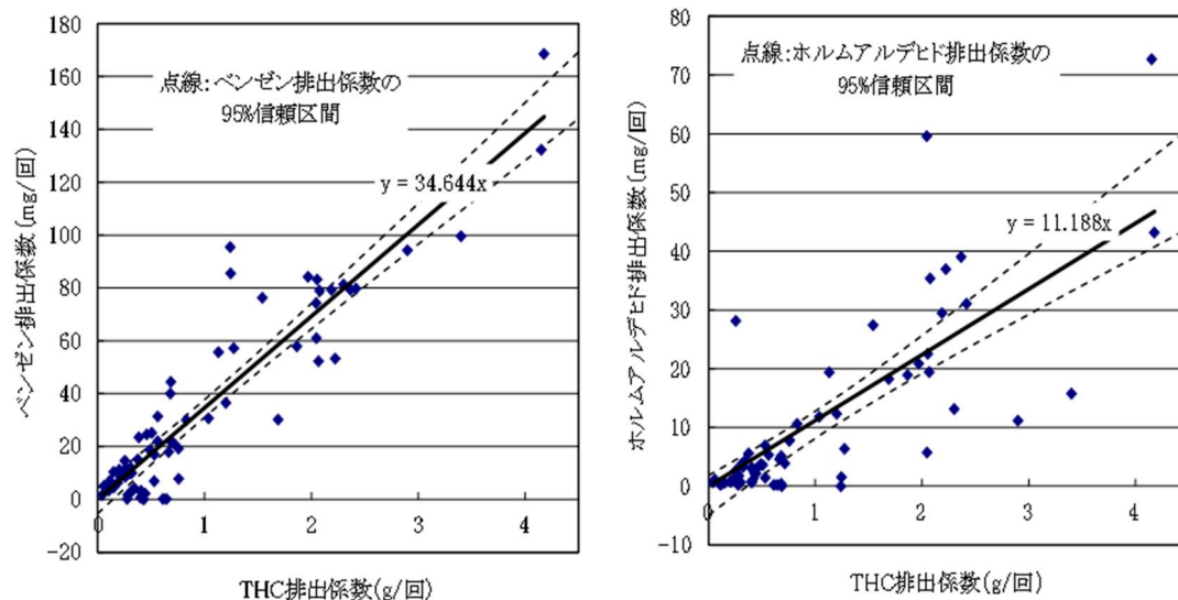
図11-41 ガソリン自動車(コールドスタート時の増分)に係るTHC排出量と対象化学物質別排出量の比率(その3)
