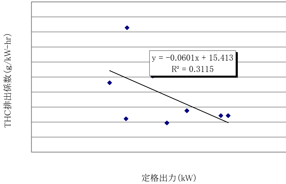
図 14-16 定格出力と THC 排出係数の関係の例(小型特殊船舶(4st))
