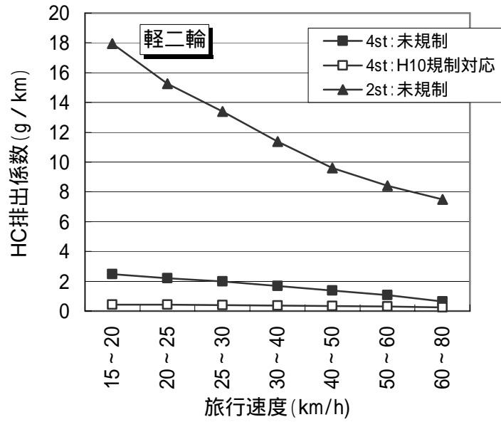
図 13-5 旅行速度区別THC 排出係数(軽二種)
