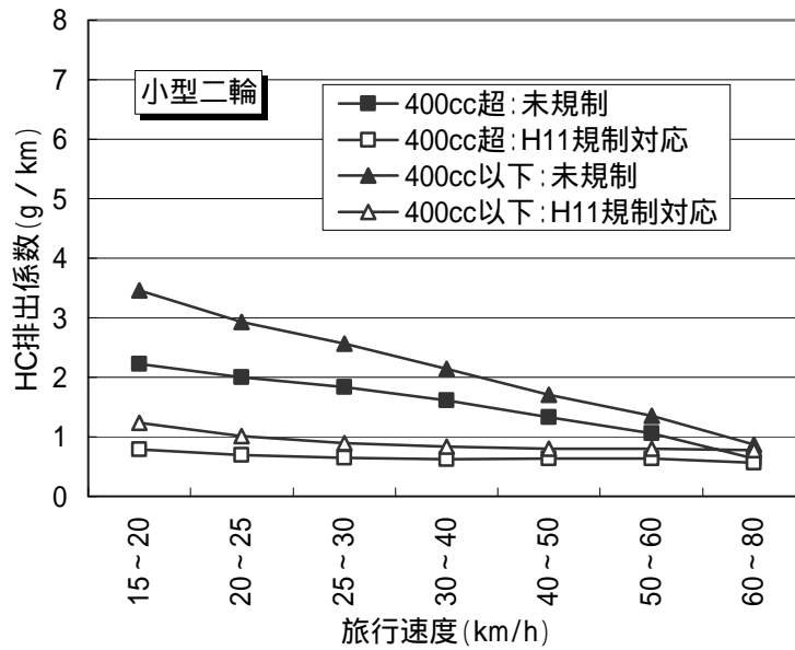
図 13-6 旅行速度区別THC 排出係数(小型二輪)
