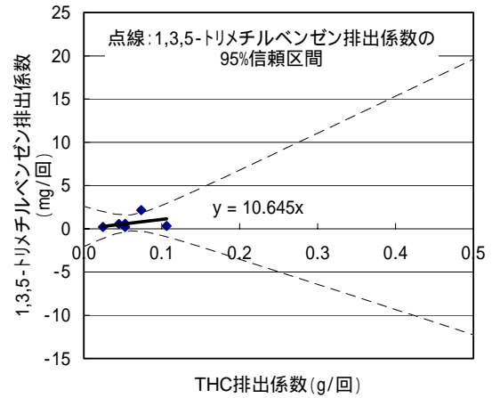
図 12-43 ディーゼル自動車(コールドスタート時の増分)に係る THC 排出量と対象化学物質別排出量の比率(その1)
