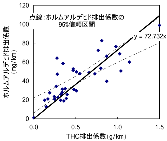
図 12-41 ディーゼル自動車(ホットスタート:重量車)に係る THC 排出量と対象化学物質別排出量の比率(その2)
