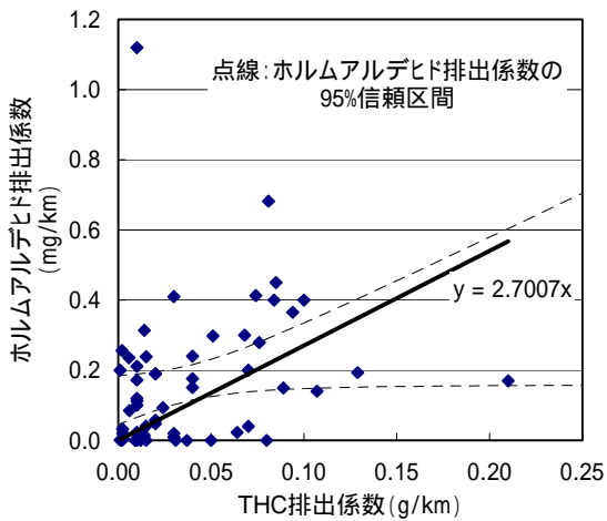
図 12-38 ガソリン自動車(ホットスタート)に係る THC 排出量と対象化学物質別排出量の比率(その2)
