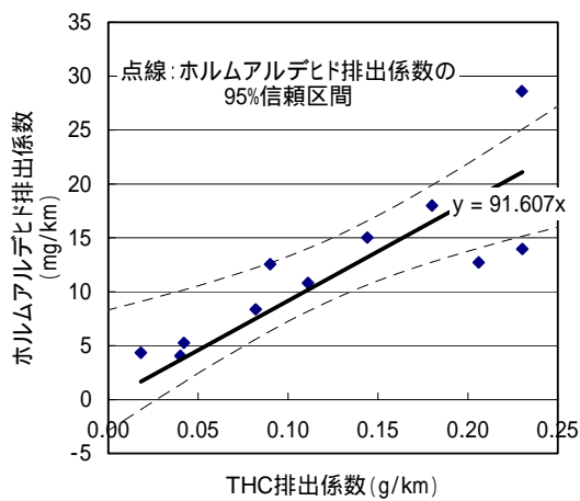
図 12-40 ディーゼル自動車(ホットスタート:重量車以外(触媒なし))に係る THC 排出量と対象化学物質別排出量の比率(その2)
