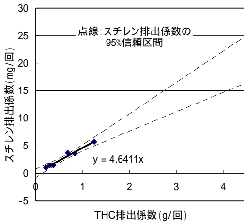
図 12-42 ガソリン自動車(コールドスタート時の増分)に係る THC 排出量と対象化学物質別排出量の比率(その1)
