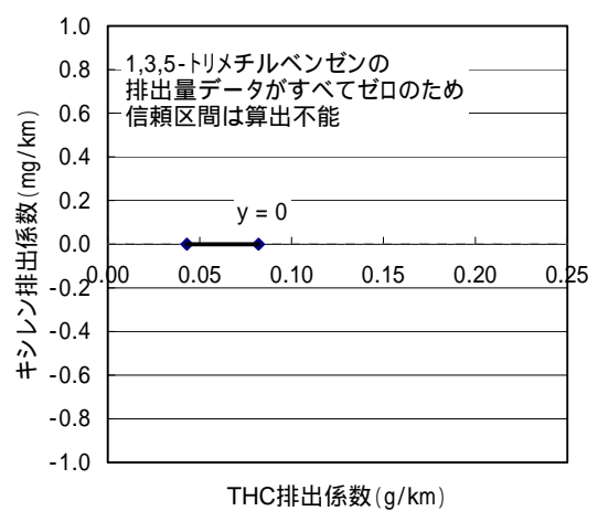
図 12-40 ディーゼル自動車(ホットスタート:重量車以外(触媒なし))に係る THC 排出量と対象化学物質別排出量の比率(その1)
