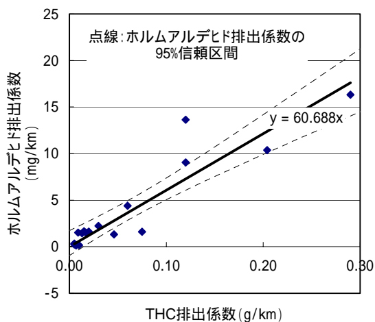
図 12-39 ディーゼル自動車(ホットスタート:重量車以外(触媒あり))に係る THC 排出量と対象化学物質別排出量の比率(その2)
