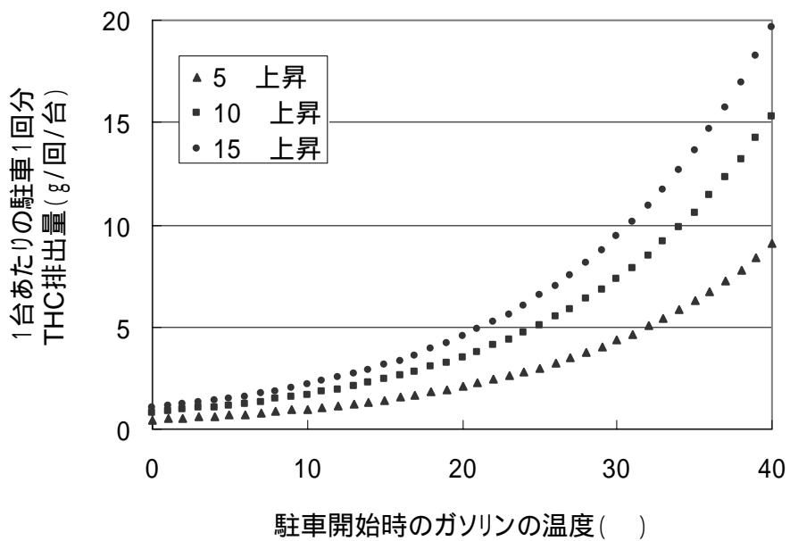
図 12-45 1台あたりの駐車1回分 THC 排出量(夏、普通乗用車の例)
