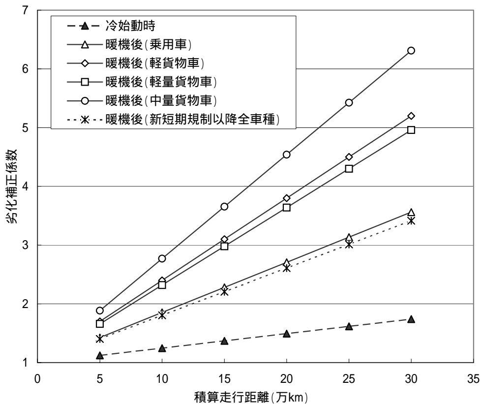
出典:「JCAP 技術報告書、大気モデル技術報告書(1)」(平成 14 年 3 月、(財)石油産業活性化センター・JCAP 推進室) 図 12-23 経過年数(積算走行距離)による劣化補正係数
