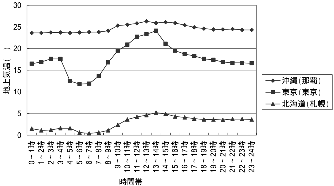
図 12-29 1日の地上気温変動の例(平成 19 年 4 月 1 日の例)
