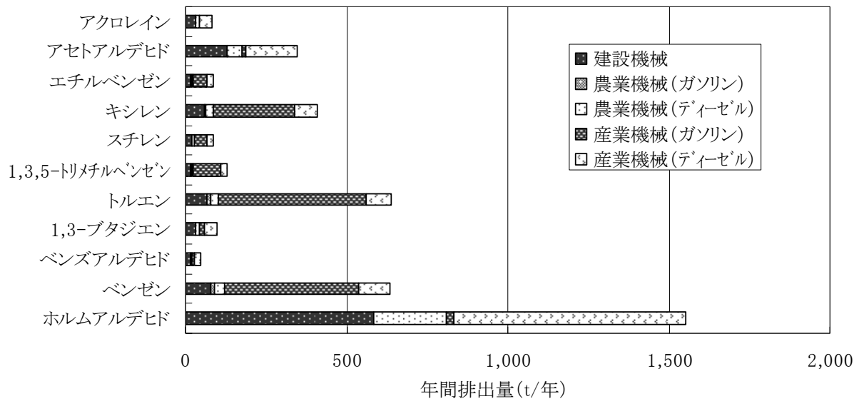
図 2 特殊自動車(建設機械・農業機械・産業機械)に係る全国合計の年間排出量の推計結果(平成 19 年度)
