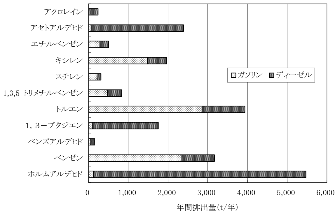
図7 自動車(ホットスタート)に係る対象化学物質別の全国排出量の推計結果(平成19年度)
