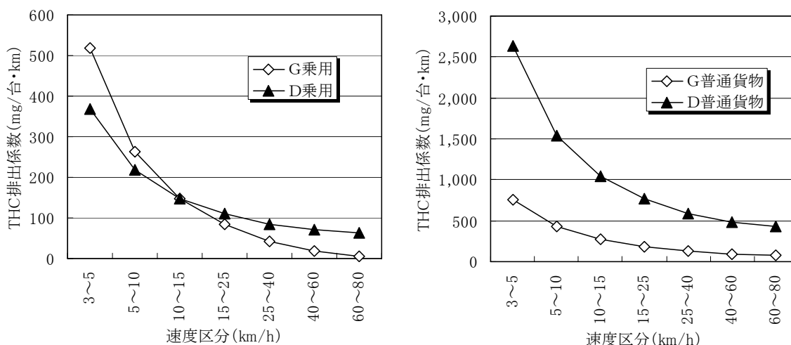
図1 車種別・旅行速度区別のTHC排出係数の例(平成19年度)
