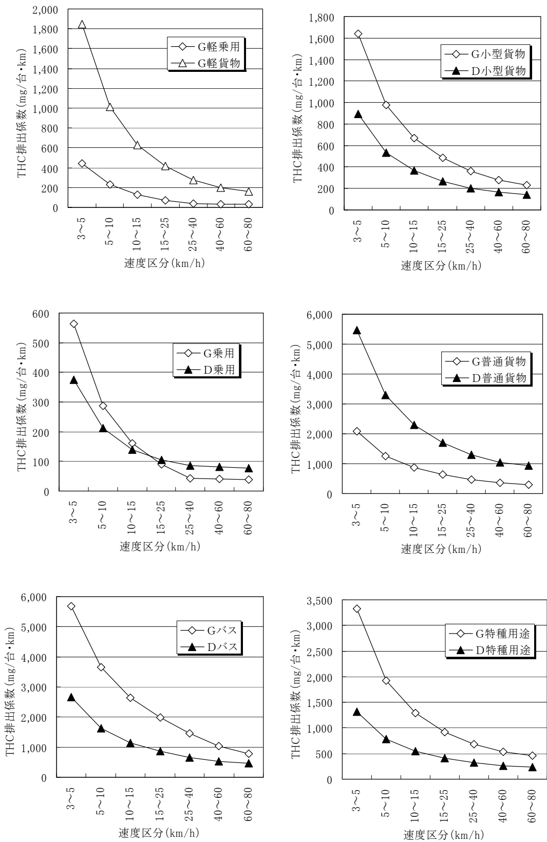
図 12-13 車種別・旅行速度区別の THC 排出係数(平成 16 年度;触媒の劣化補正後)
