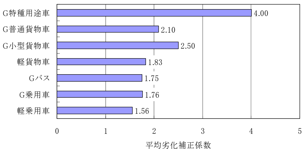
図 12-12 平均劣化補正係数の推計結果(平成16年度)
