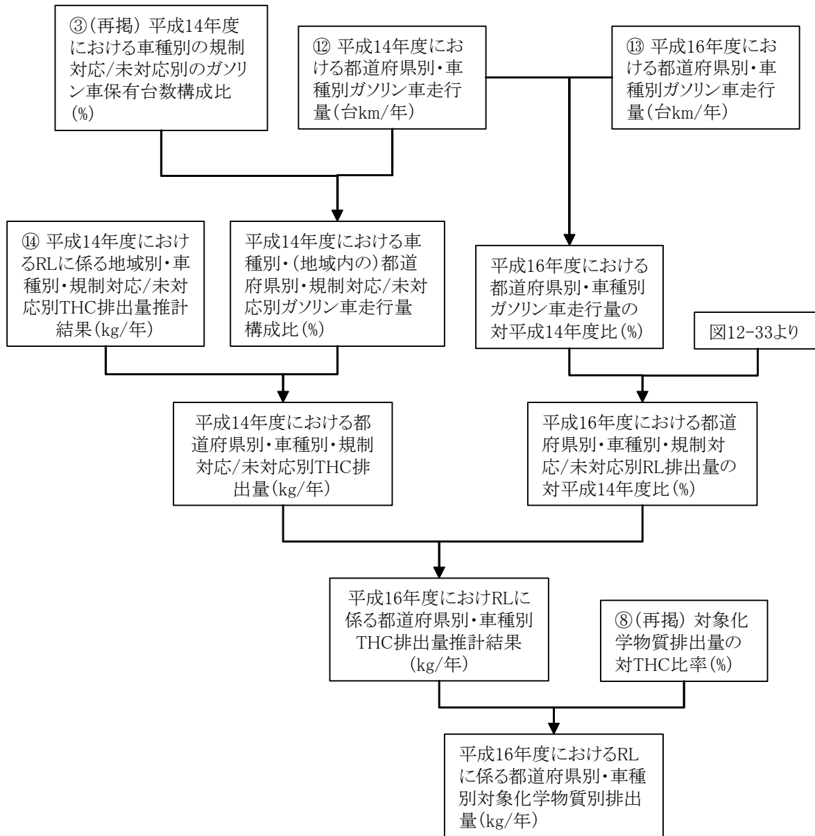
図 12-35 燃料蒸発ガス(RL)に係る対象化学物質別排出量の推計フロー
