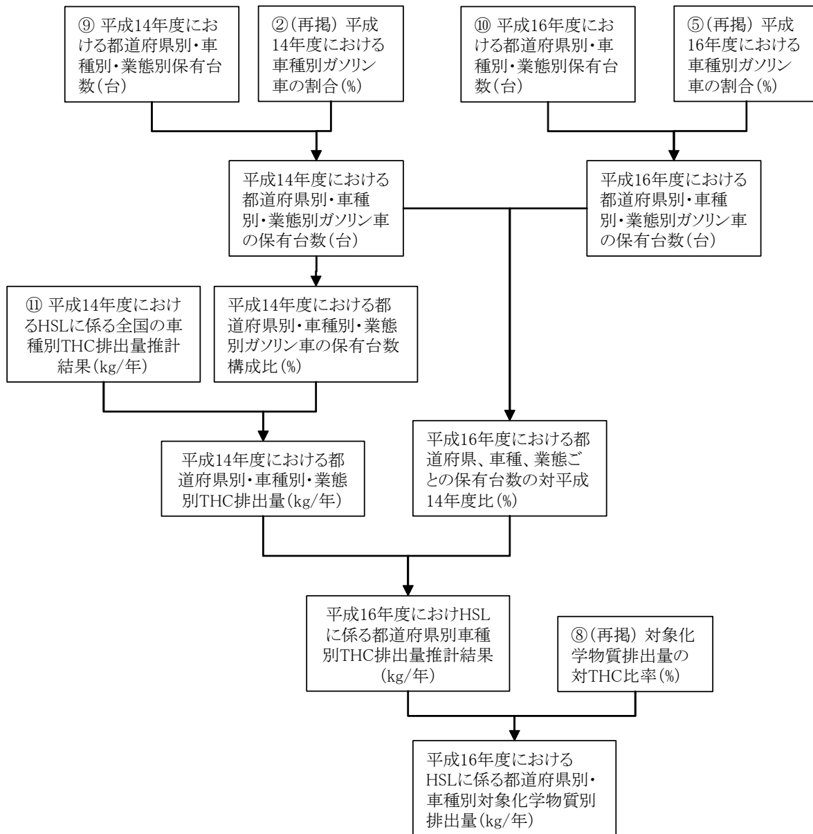
図 12-34 燃料蒸発ガス(HSL)に係る対象化学物質別排出量推計フロー
