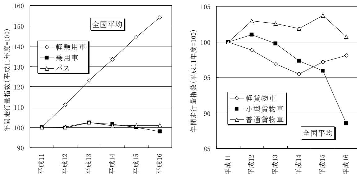
図 12-7 全国における車種別年間走行量指数の推移
