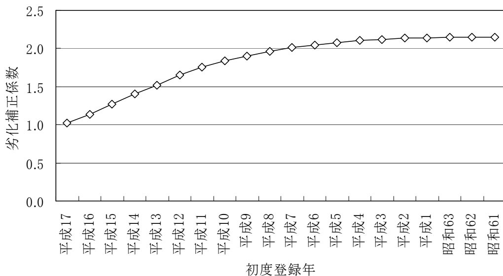
図 12-11 初度登録年別の劣化補正係数の推計結果 (平成16年度;ガソリン乗用車の例)
