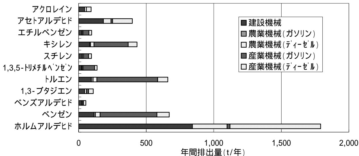
図2 特殊自動車(建設機械・農業機械・産業機械)に係る全国合計の年間排出量の推計結果(平成15年度)
