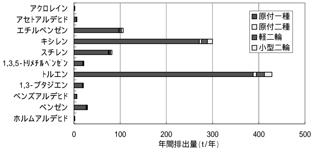
図5 コールドスタート時の増分に係る対象化学物質別の全国排出量の試算結果(平成15年度)
