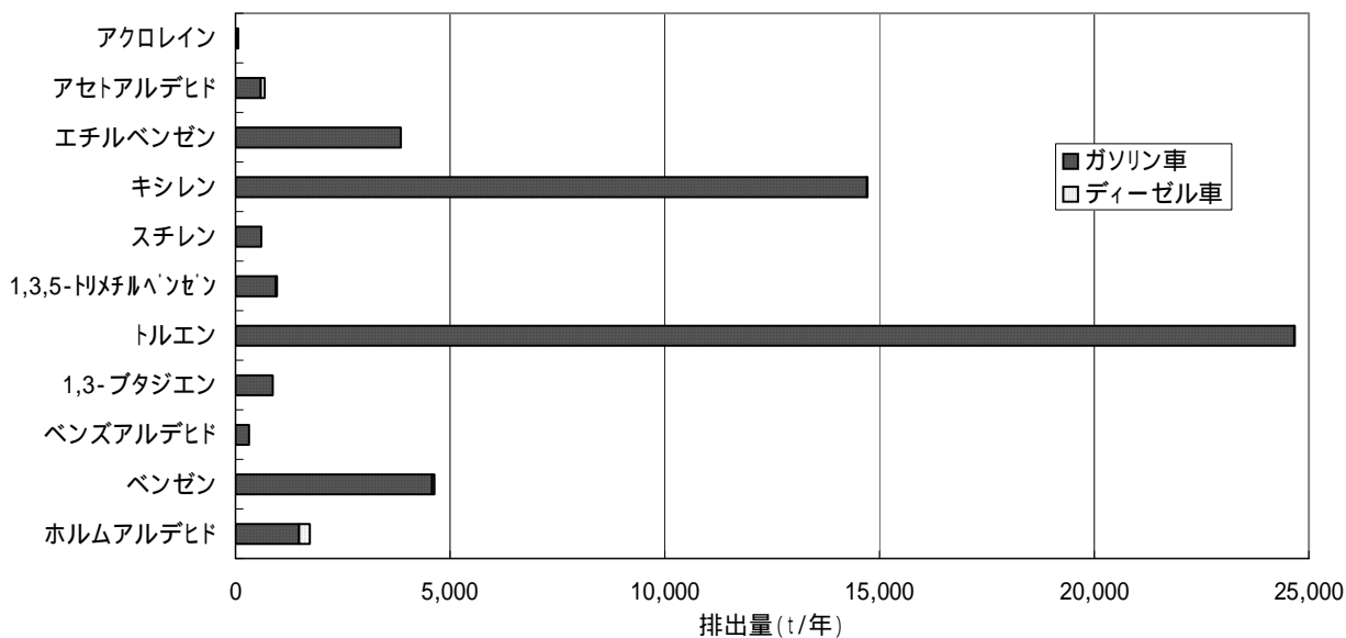
図 13 コールドスタート時の増分に係る排出量の推計結果 (平成 15 年度)
