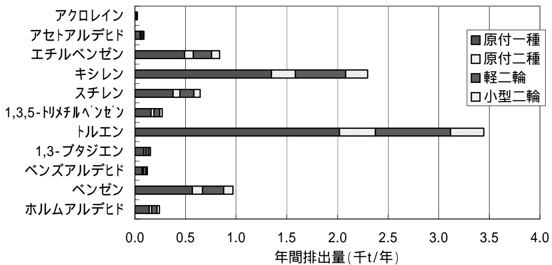
図3 ホットスタートに係る対象化学物質別の全国排出量の推計結果(平成 15 年度)
