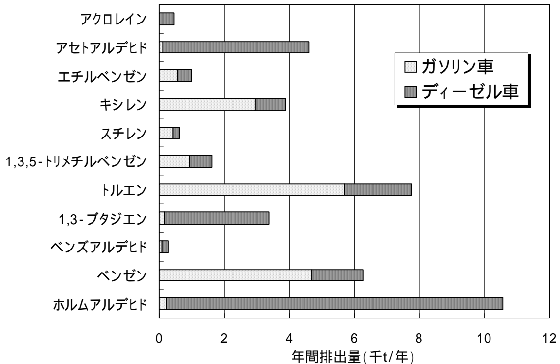
図7 自動車(ホットスタート)に係る対象化学物質別の全国排出量の推計結果(平成15年度)
