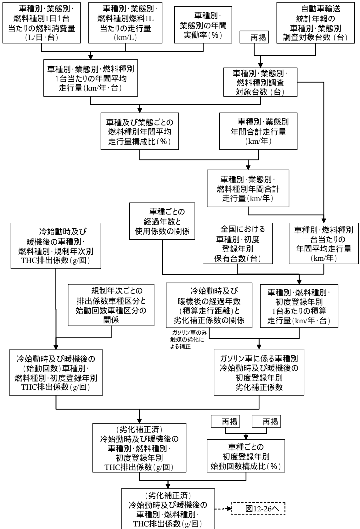
図 12-25 劣化補正済車種別・燃料種別 THC 排出係数の推計フロー
