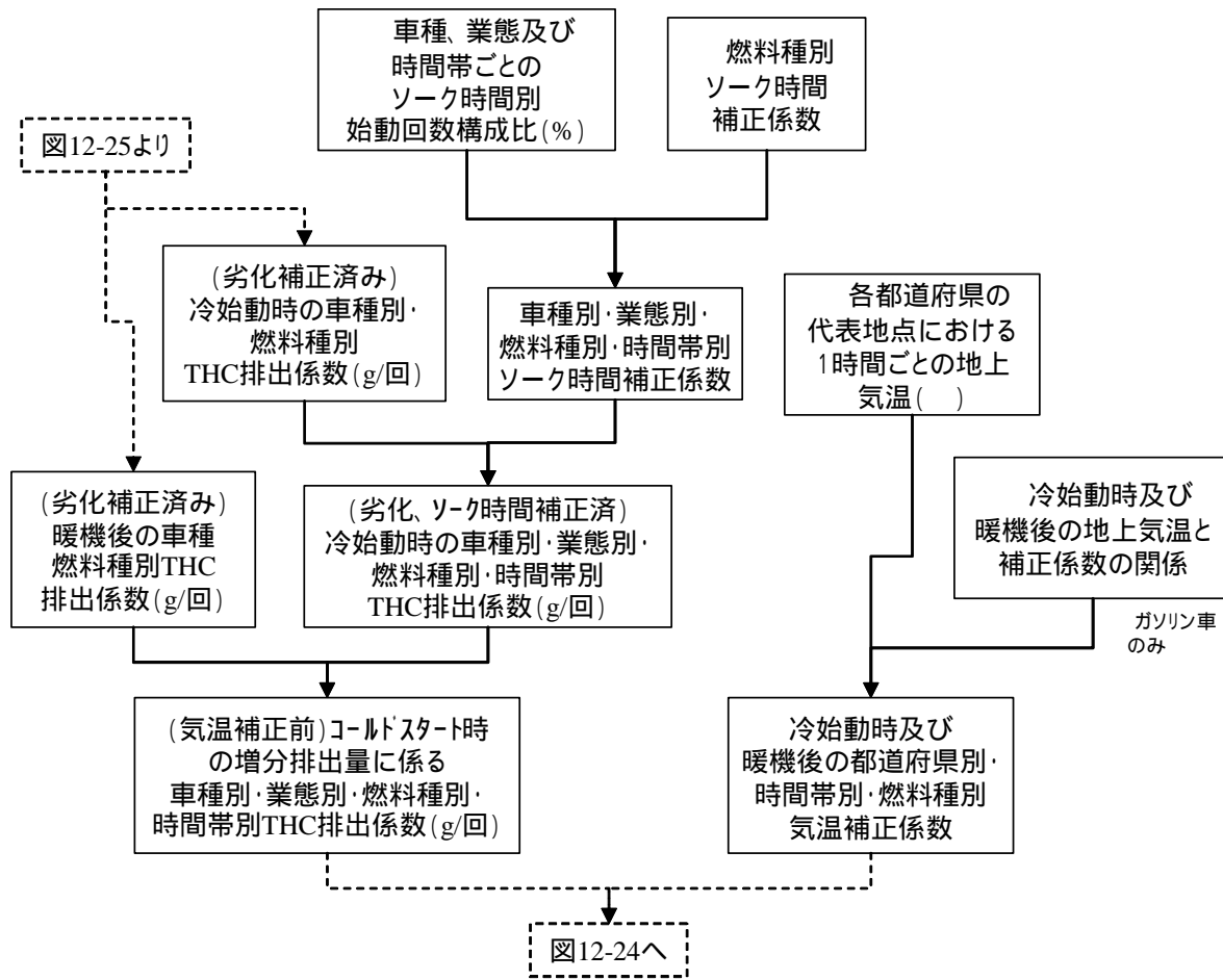
図 12-26 都道府県別・車種別・業態別・燃料種別・時間帯別 THC 排出係数の推計フロー
