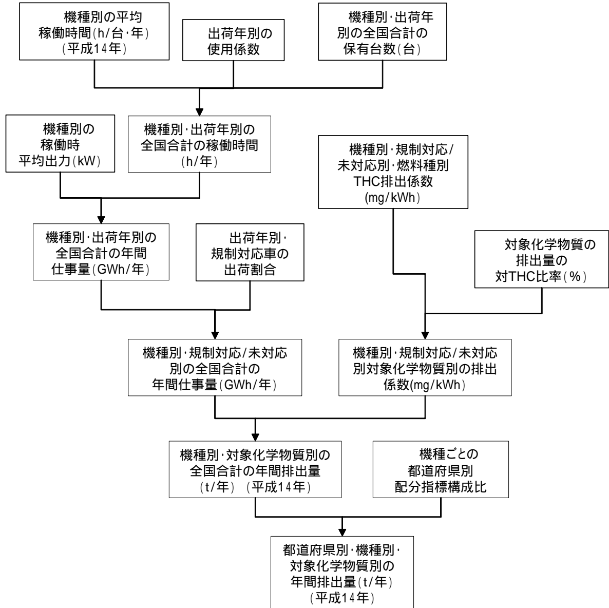
図 12-27 自動車(サブエンジン式機器)に係る排出量の推計フロー
