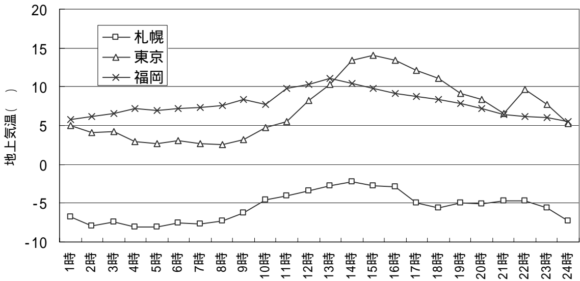
図 12-23 1日の地上気温変動の例(平成 14 年 1 月 1 日の例)
