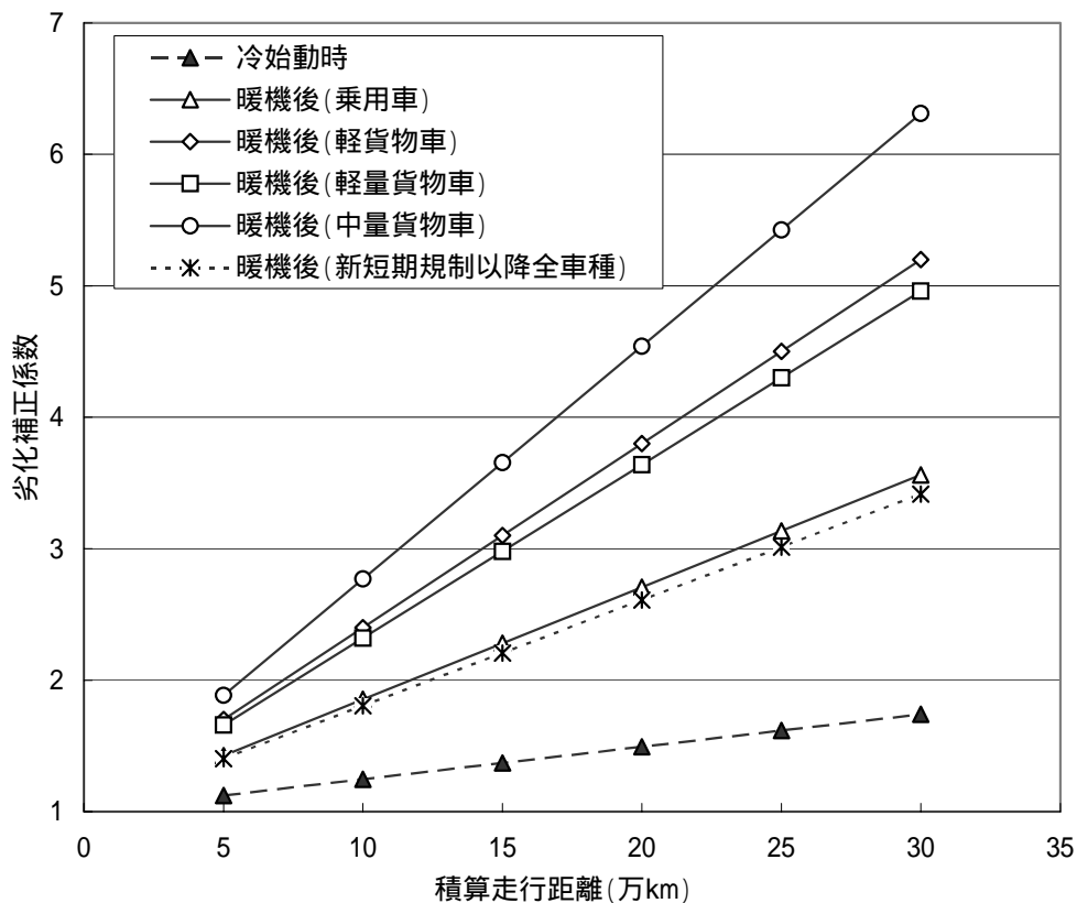
図 12-17 経過年数(積算走行距離)による劣化補正係数
