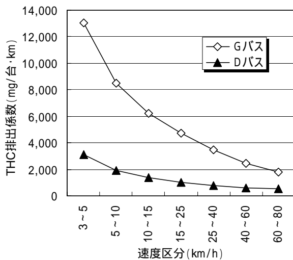
図 12-9 車種別・速度区別の THC 排出係数(平成 14 年度)
