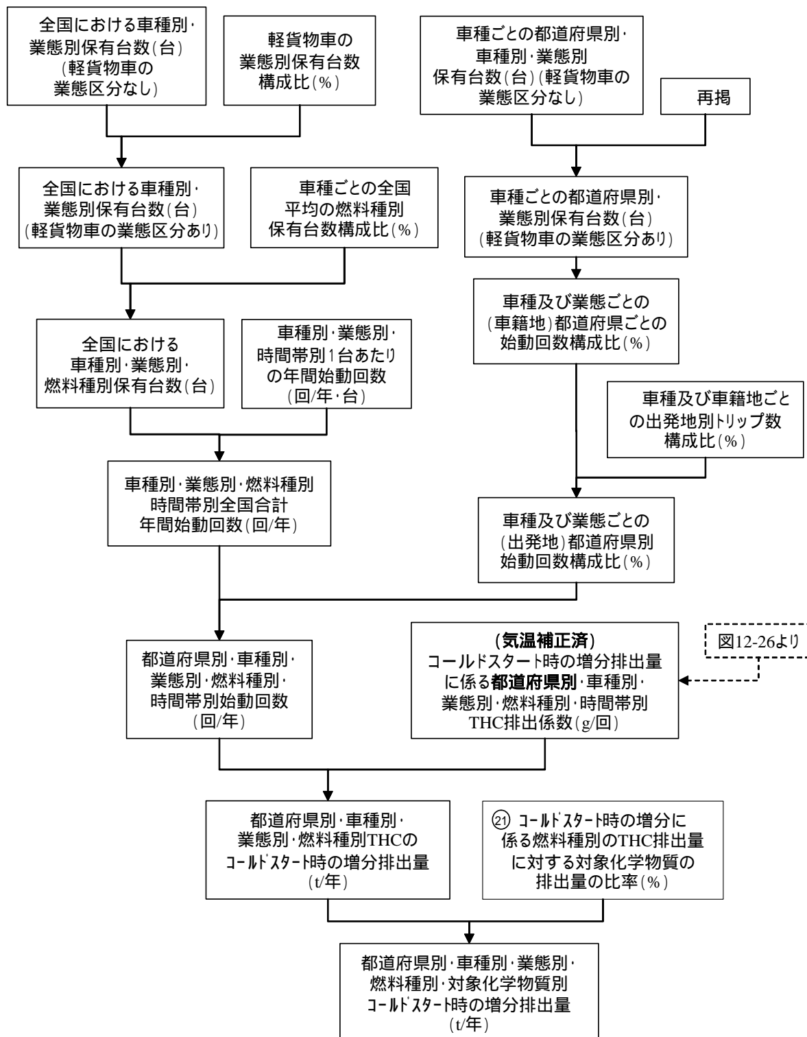
図 12-24 コールドスタート時の増分に係る排出量の推計フロー
