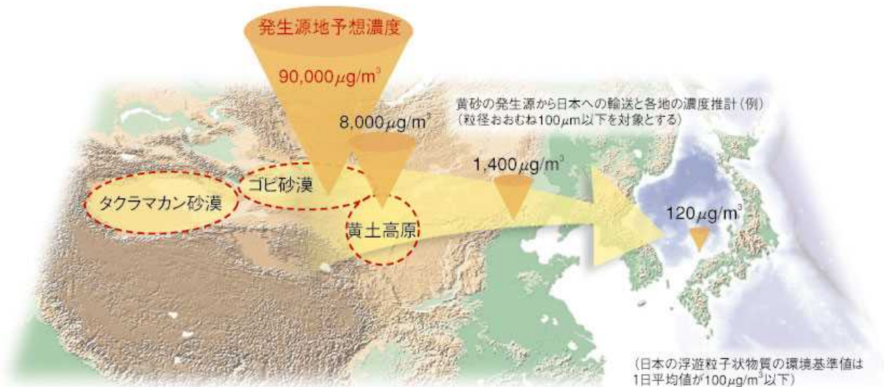
図 1-3 黄砂の発源地地域
