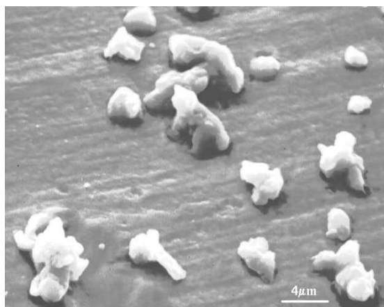
図 1-6 黄砂粒子の電子顕微鏡写真
