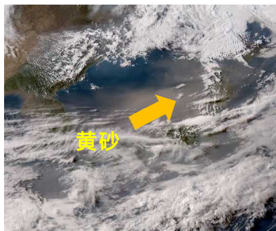
図 1-5 ひまわり 8 号による画像 (2016/5/7)
