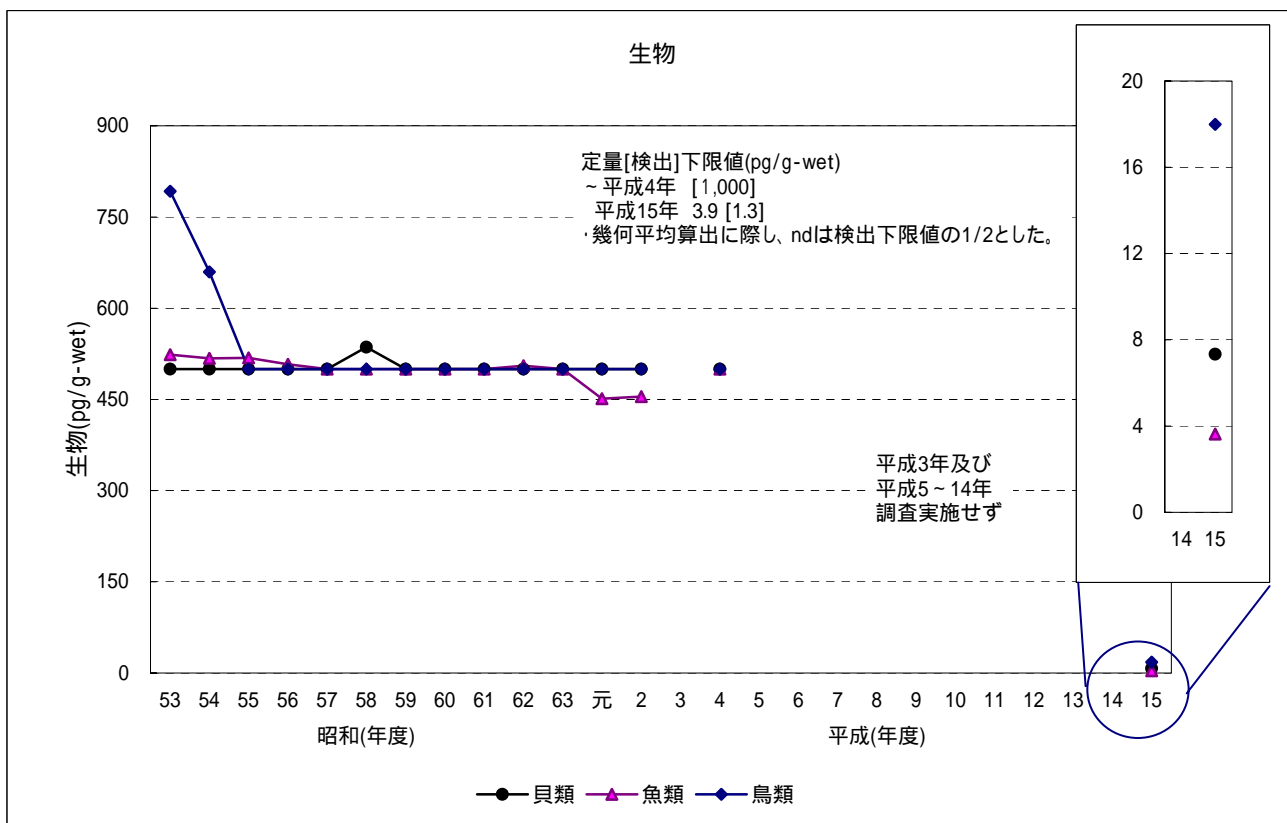
図31 -HCHの経年変化図(幾何平均値)
